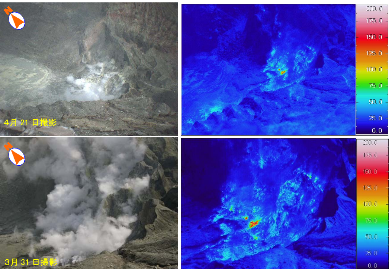
図 11 阿蘇山 赤外熱映像装置による中岳第一火口南側火口壁の地表面温度分布 南側火口壁の温度分布に特段の変化はありません。
