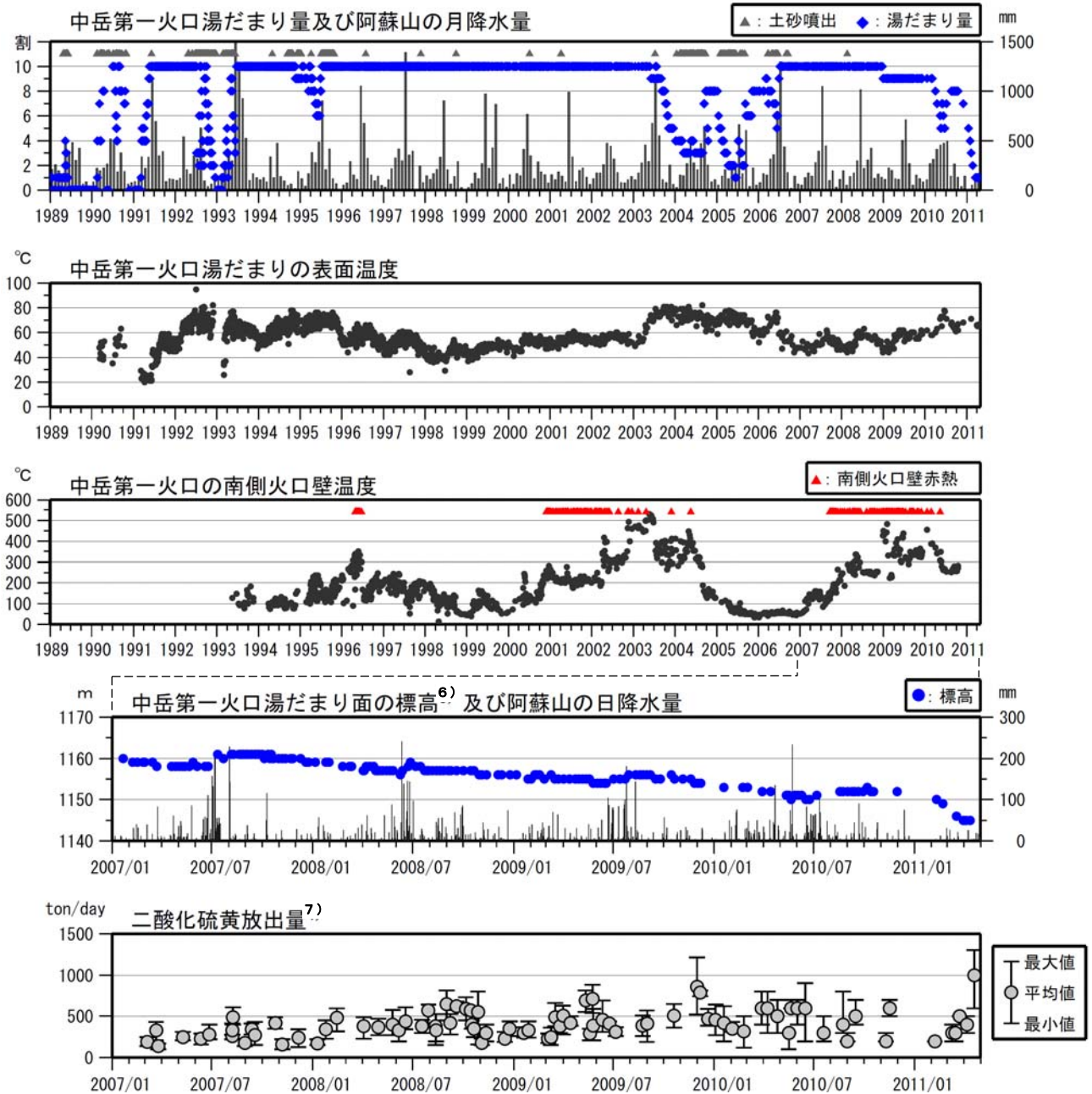
図 3※ 阿蘇山 湯だまり、火口壁、二氧化硫黄放出量の状況（1989 年 1 月～2011 年 4 月） < 4 月の状況 >
