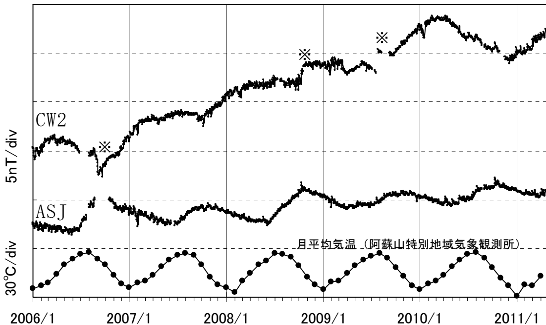
図 7 阿蘇山 全磁力連続観測による阿蘇山麓 (AHK) を基準とした中岳第一火口周辺の全磁力変化及び阿蘇山特別地域気象観測所における月平均気温 (2006 年 1 月～2011 年 4 月) 中岳第一火口の北西側火口縁にある観測点 (CW2) では、2010 年 4 月頃から全磁力が減少していましたが、2010 年 12 月以降は増加に転じています。
