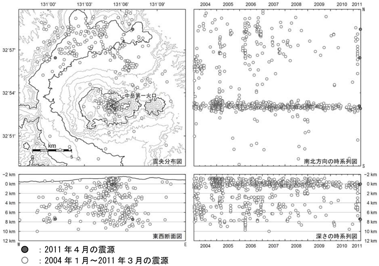
図 4※ 阿蘇山 震源分布図 (2004 年 1 月～2011 年 4 月)
