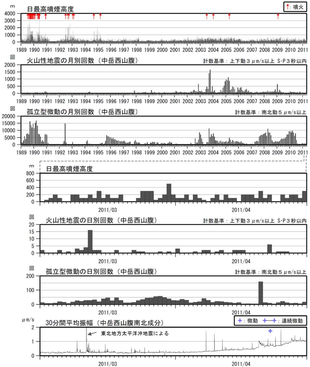
図2 阿蘇山 噴煙、火山性地震、孤立型微動の状況（1989年1月～2011年4月）
