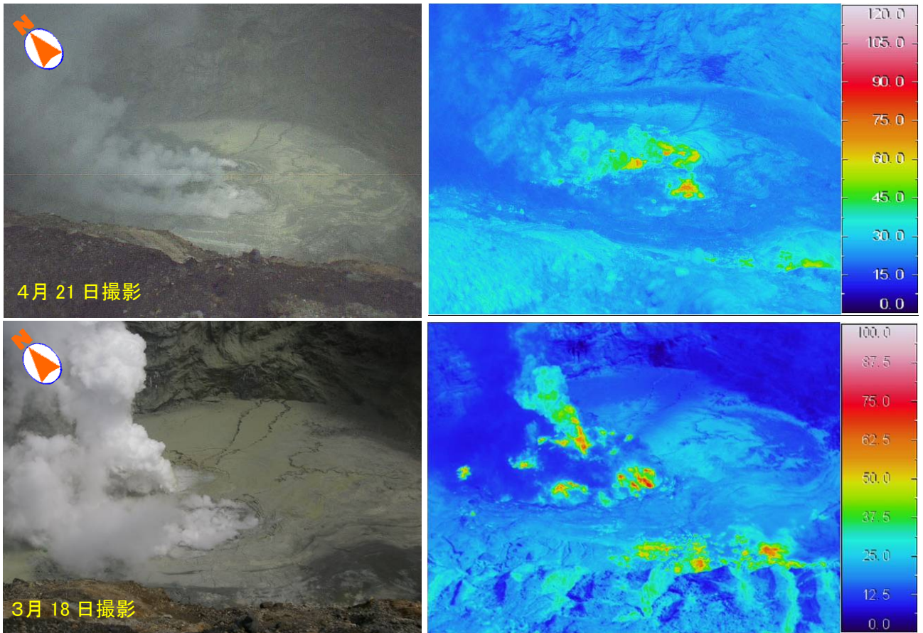
図 10 阿蘇山 赤外熱映像装置による中岳第一火口底の地表面温度分布 火口底の温度分布に特段の変化はありません。
