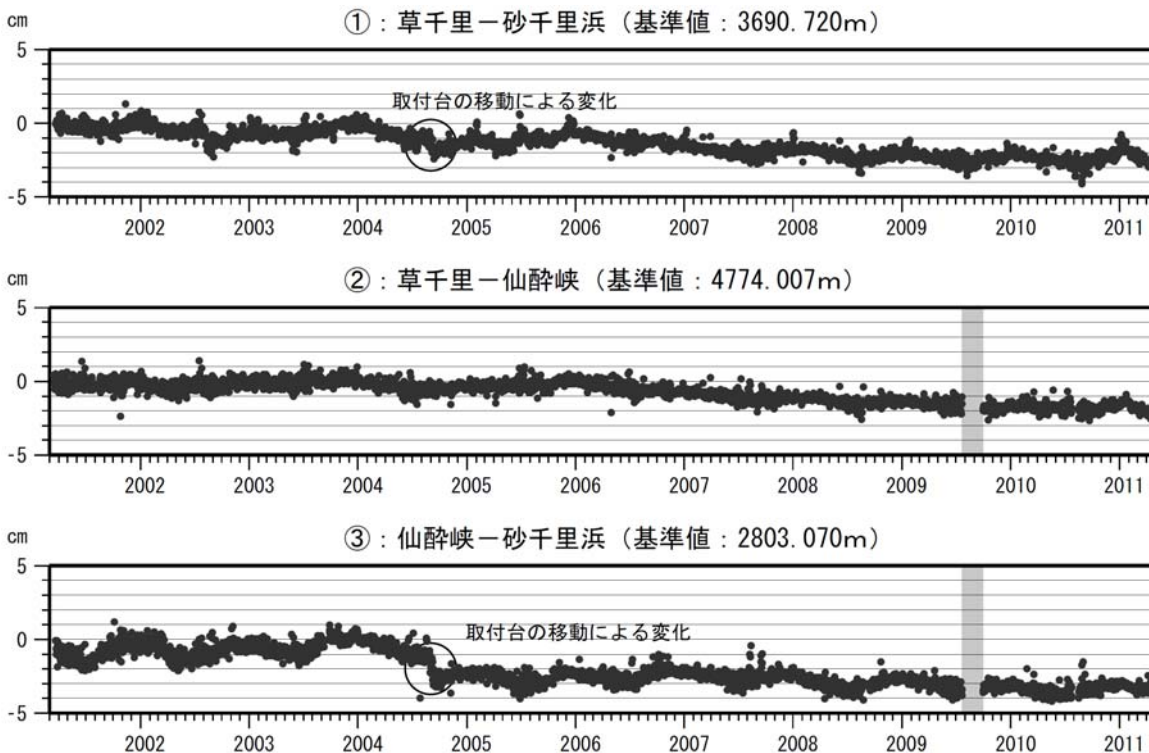
図 5 阿蘇山 GPS連続観測による基線長変化 (2001 年 3 月～2011 年 4 月)
