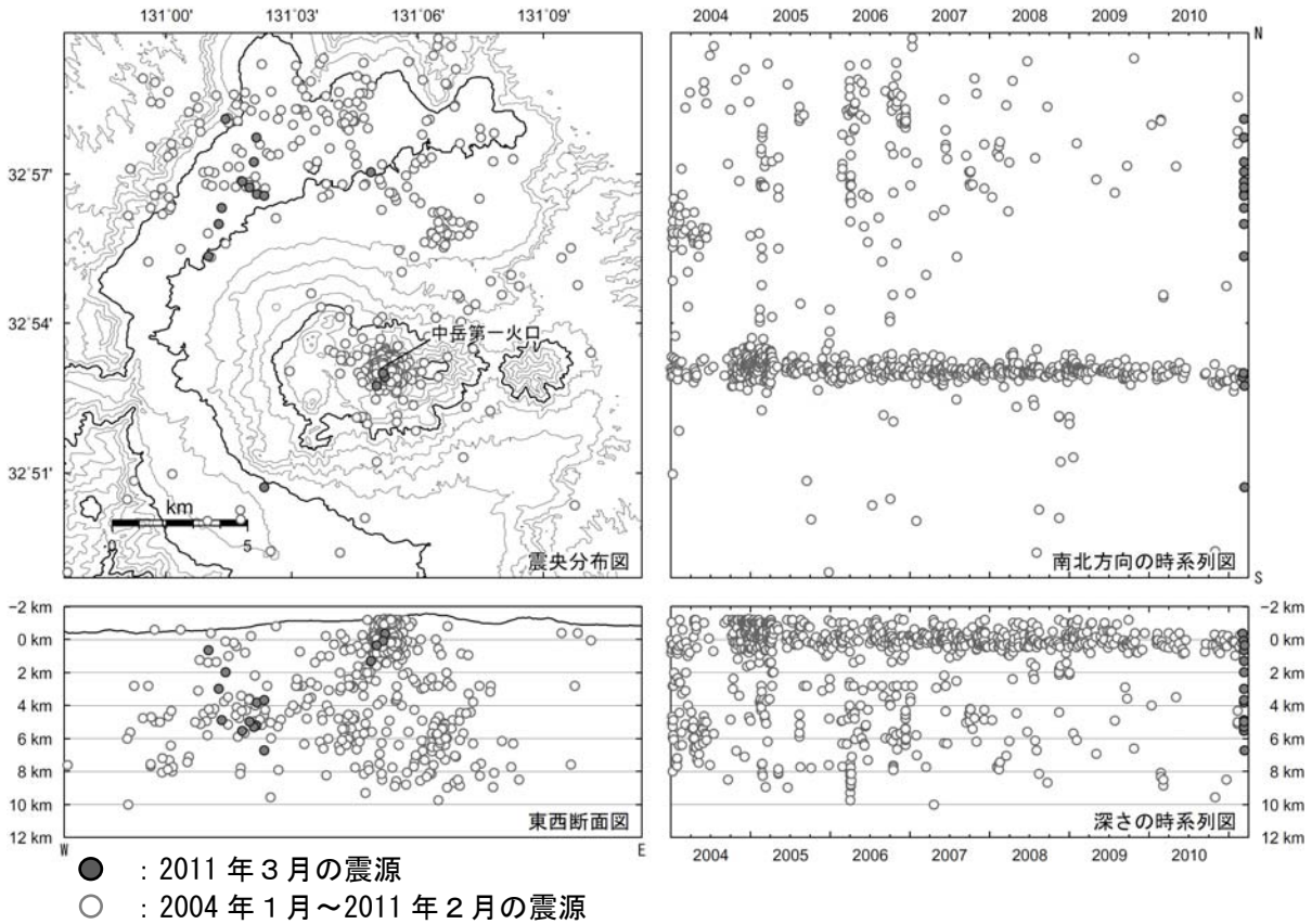
図 4※ 阿蘇山 震源分布図 (2004 年 1 月～2011 年 3 月)
