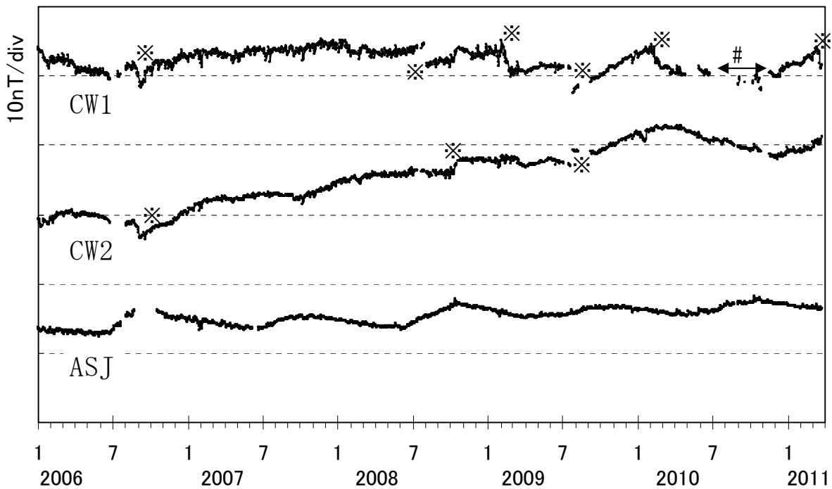
図 7 阿蘇山 全磁力連続観測による阿蘇山麓 (AHK) を基準とした中岳第一火口周辺の全磁力変化 (2006 年 1 月～2011 年 3 月)
