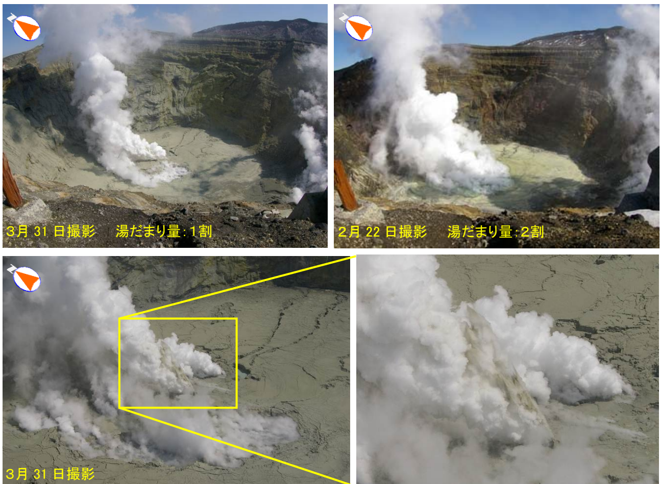
図 9 阿蘇山 中岳第一火口南西側定点から第一火口内の状況
