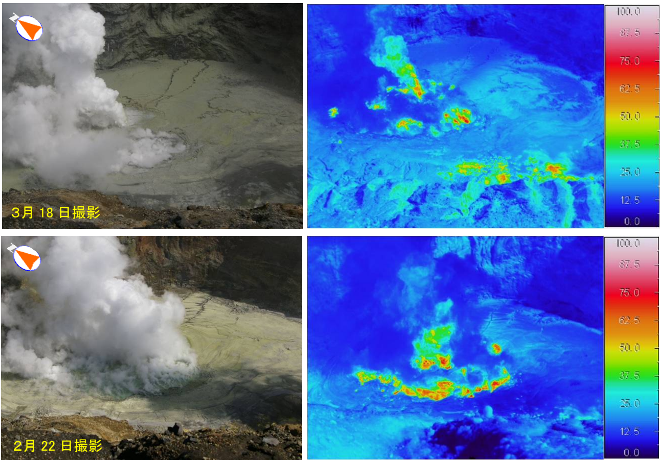
図 10 阿蘇山 熱映像による中岳第一火口南西側定点から火口底の状況 火口底の温度分布に特段の変化はありません。
