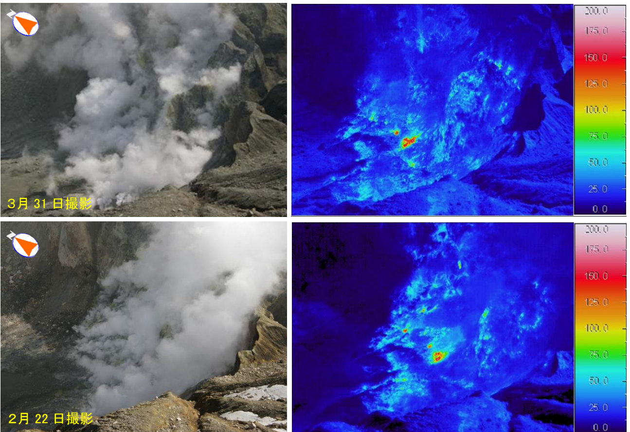
図 11 阿蘇山 熱映像による中岳第一火口南西側定点から南側火口壁の状況 南側火口壁の温度分布に特段の変化はありません。
