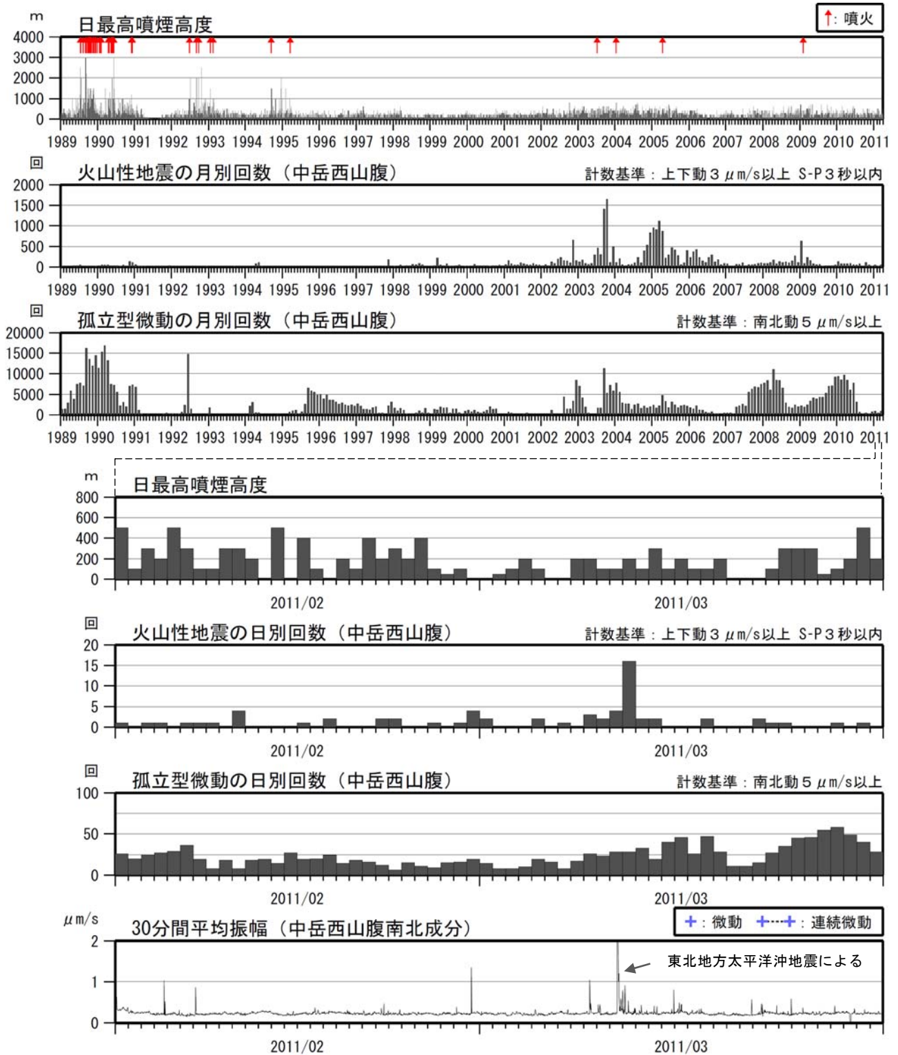
図2 阿蘇山 噴煙、火山性地震、孤立型微動の状況（1989年1月～2011年3月）
