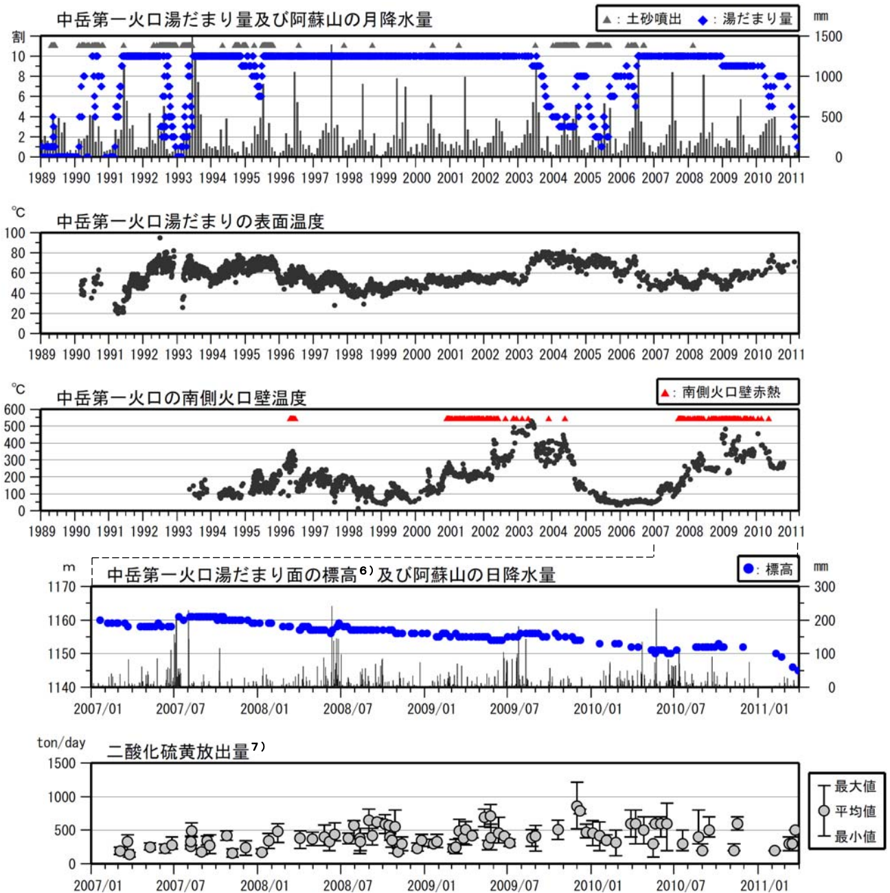
図 3※ 阿蘇山 湯だまり、火口壁、二氧化硫黄放出量の状況（1989 年 1 月～2011 年 3 月） < 3 月の状況 >
