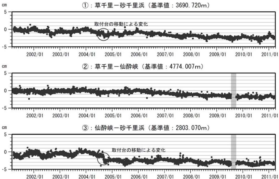
図 5 阿蘇山 GPS連続観測による基線長変化 (2001 年 3 月～2011 年 3 月)
