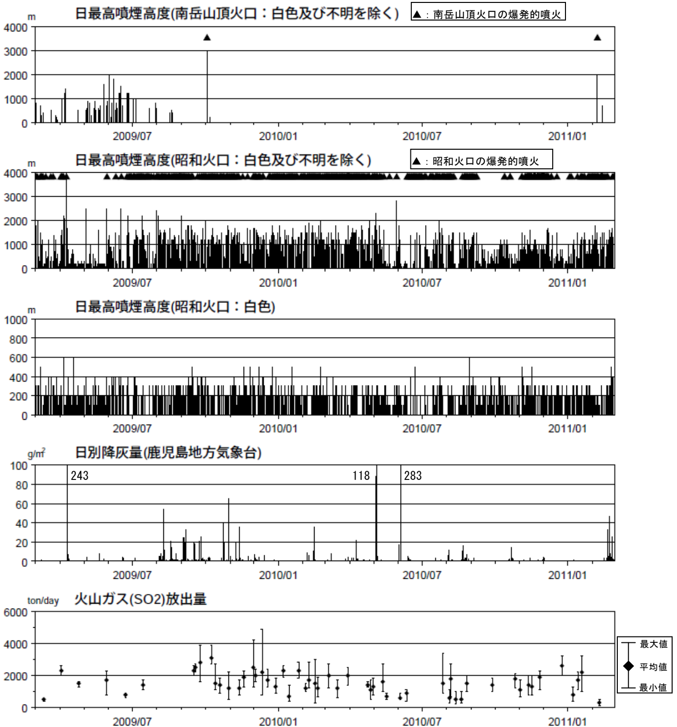
図 4 桜島 最近 2 年間の噴煙、降灰、火山ガス（2009 年 3 月～2011 年 2 月）
