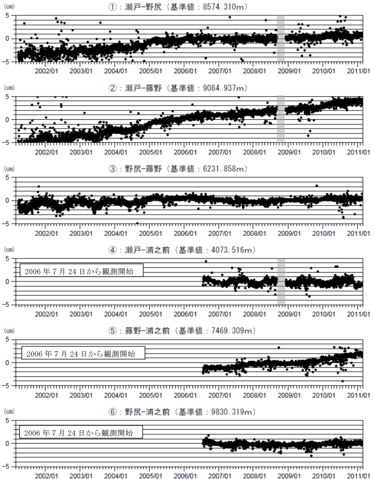
図 8 桜島 GPS 連続観測による長期の基線長変化（2001 年 3 月～2011 年 2 月） 桜島島内で火山活動に起因する特段の変化はありませんでした。
