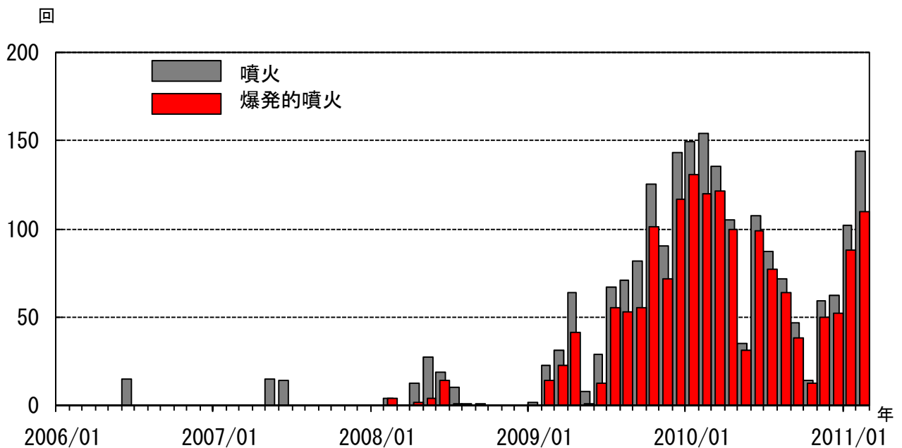
図3 桜島 昭和火口月別噴火回数（灰色）と昭和火口月別爆発回数（赤色） （2006年1月～2011年2月）
