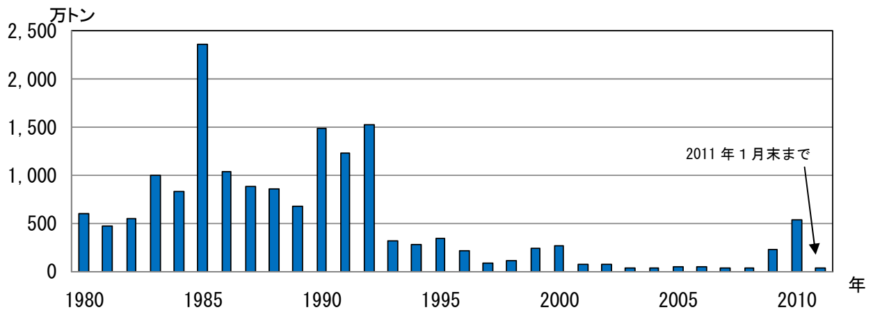
図 11※ 桜島 鹿児島県が実施している降灰量観測による年別降灰量 (1980 年～2011 年)
