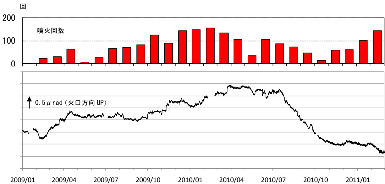
図 7※ 桜島 有村観測坑道の水管傾斜計の変化（2009 年 1 月～2011 年 2 月）
