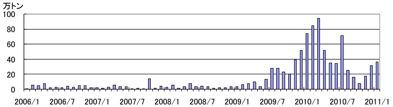
図 10※ 桜島 鹿児島県が実施している降灰量観測による月別降灰量 (2006 年 1 月～2011 年 1 月)
