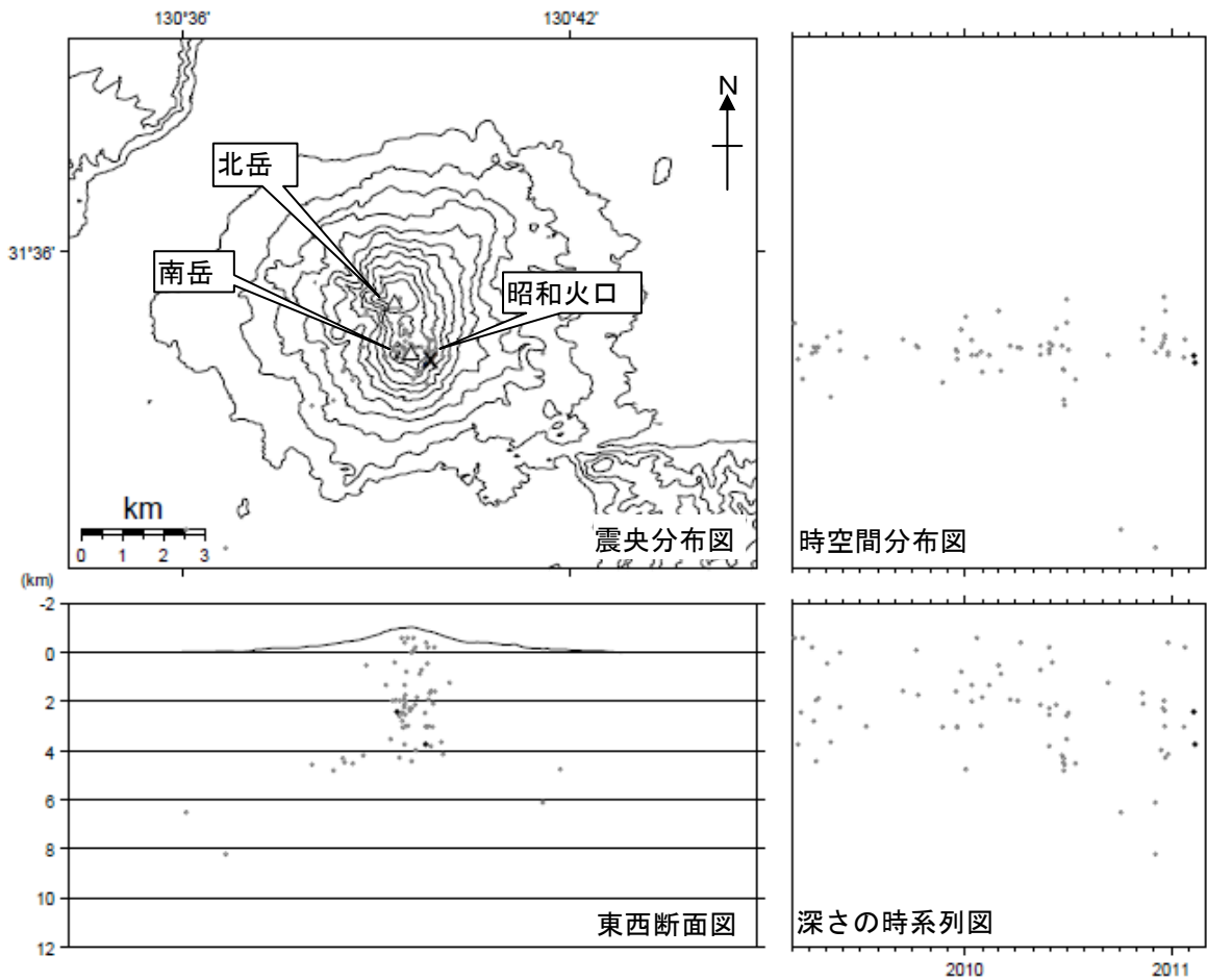
図 6※ 桜島 震源分布図（2009 年 3 月～2011 年 2 月）
