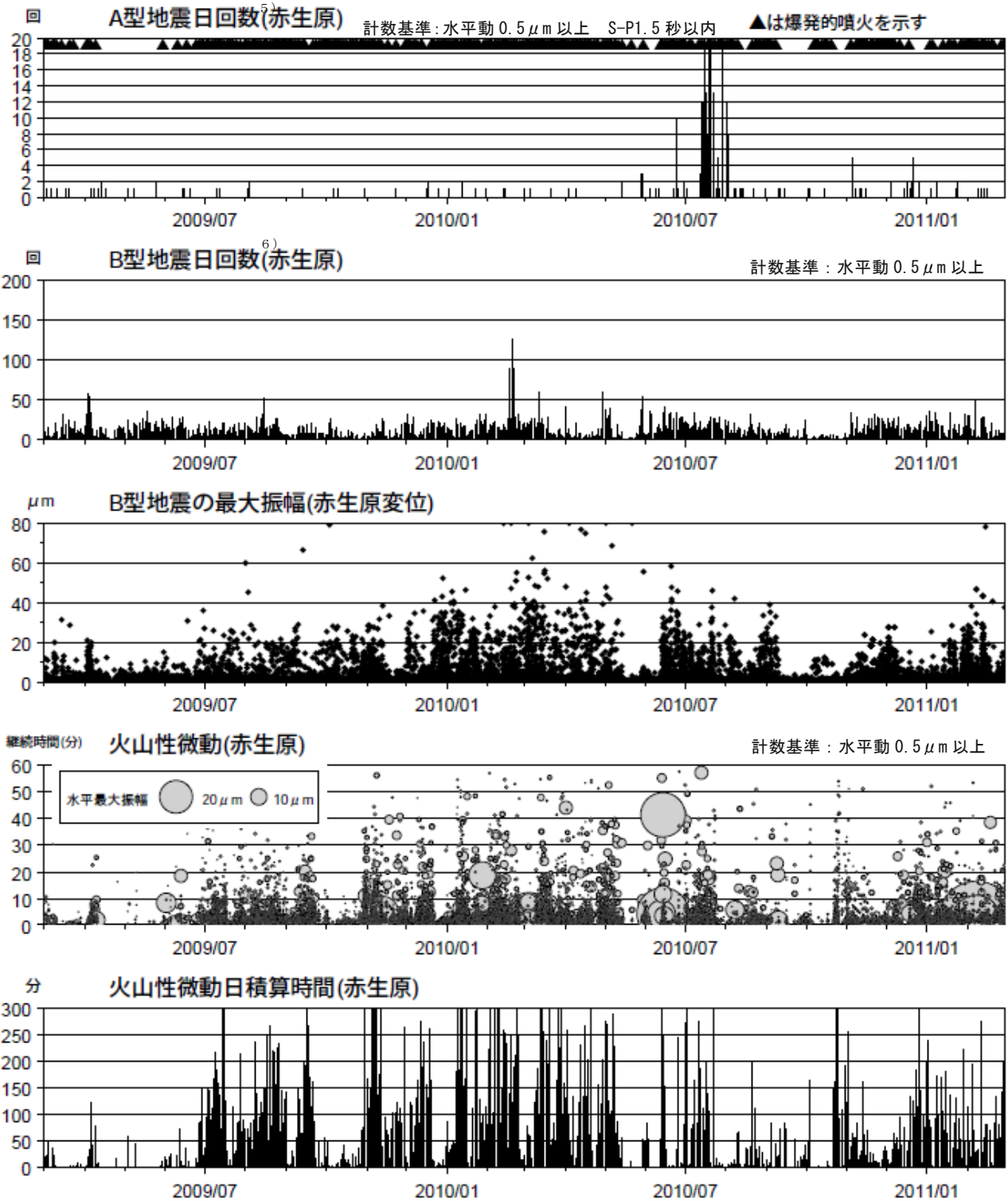
図5 桜島 最近2年間の火山性地震、火山性微動（2009年3月～2011年2月） < 2月の状況 >
