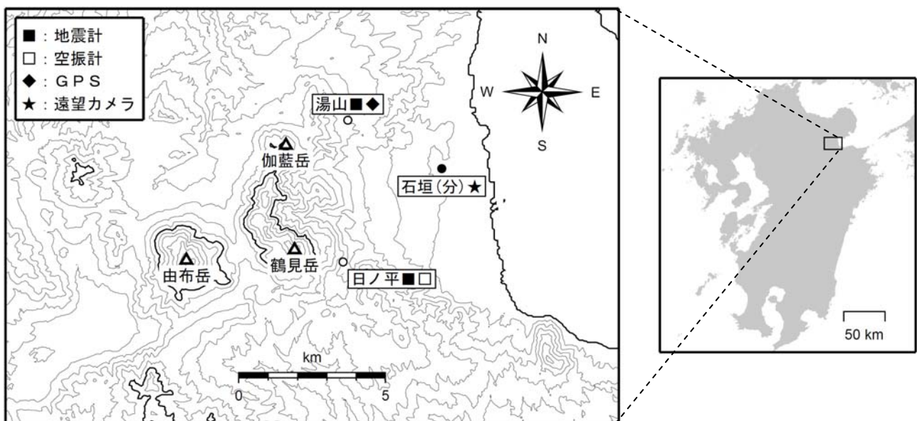
図 1 鶴見岳・伽藍岳 観測点配置図
