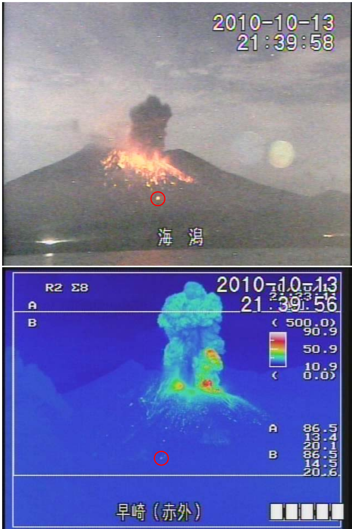
図 桜島 13日21時39分の爆発的噴火（上：海潟カメラの可視画像、下：早崎カメラの熱画像） 噴煙は火口縁上1200mまで上がり、弾道を描いて飛散する大きな噴石は4合目（昭和火口から800～1300m）まで達しました。 ※図中の赤丸は4合目まで飛散した大きな噴石を示す ※九州地方整備局大隅河川国道事務所設置の監視カメラ（海潟カメラ：昭和火口から南南東約6km、早崎カメラ：昭和火口から南東約5km）による
