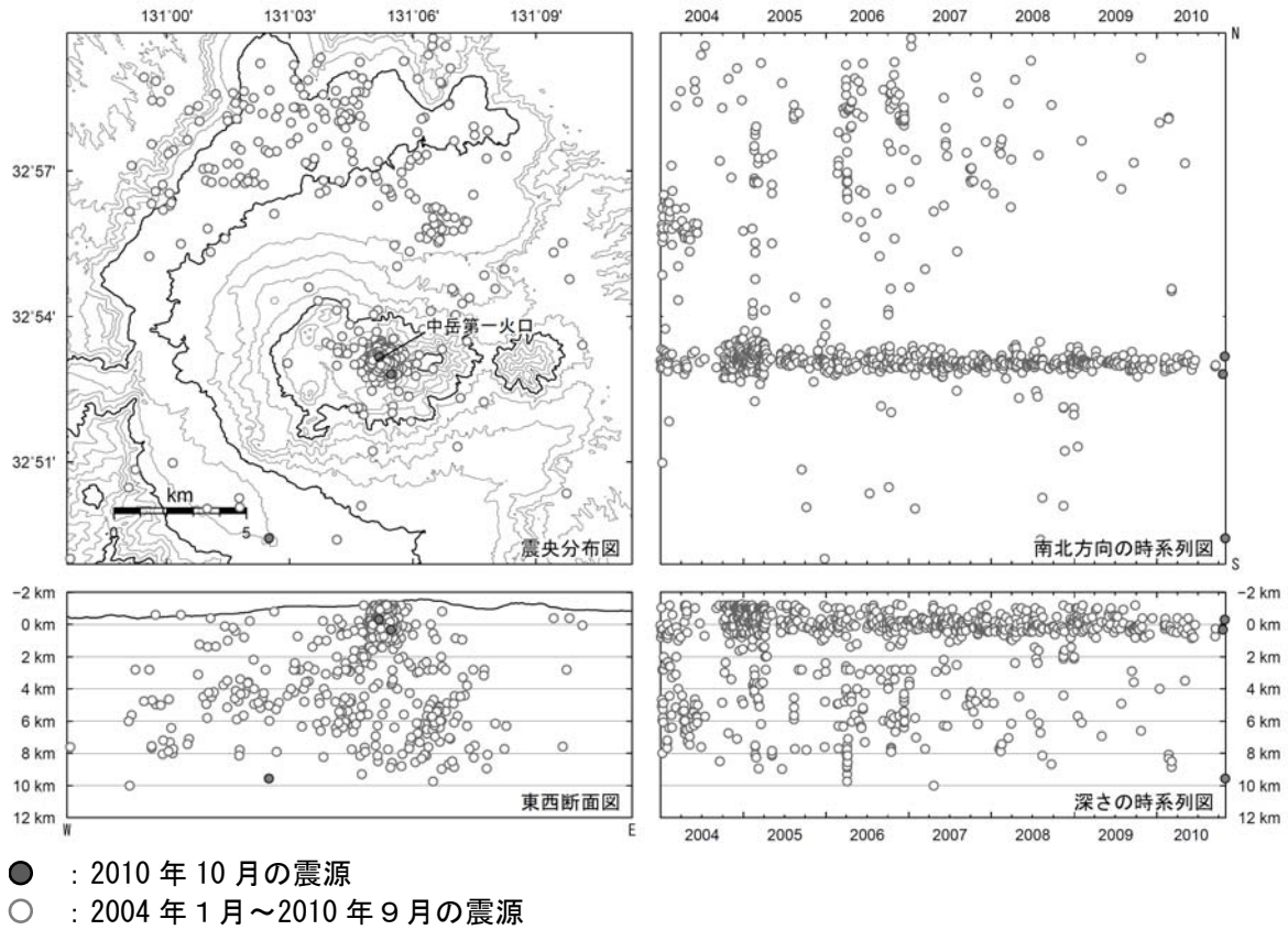
● : 2010 年 10 月の震源 ○ : 2004 年 1 月～2010 年 9 月の震源
