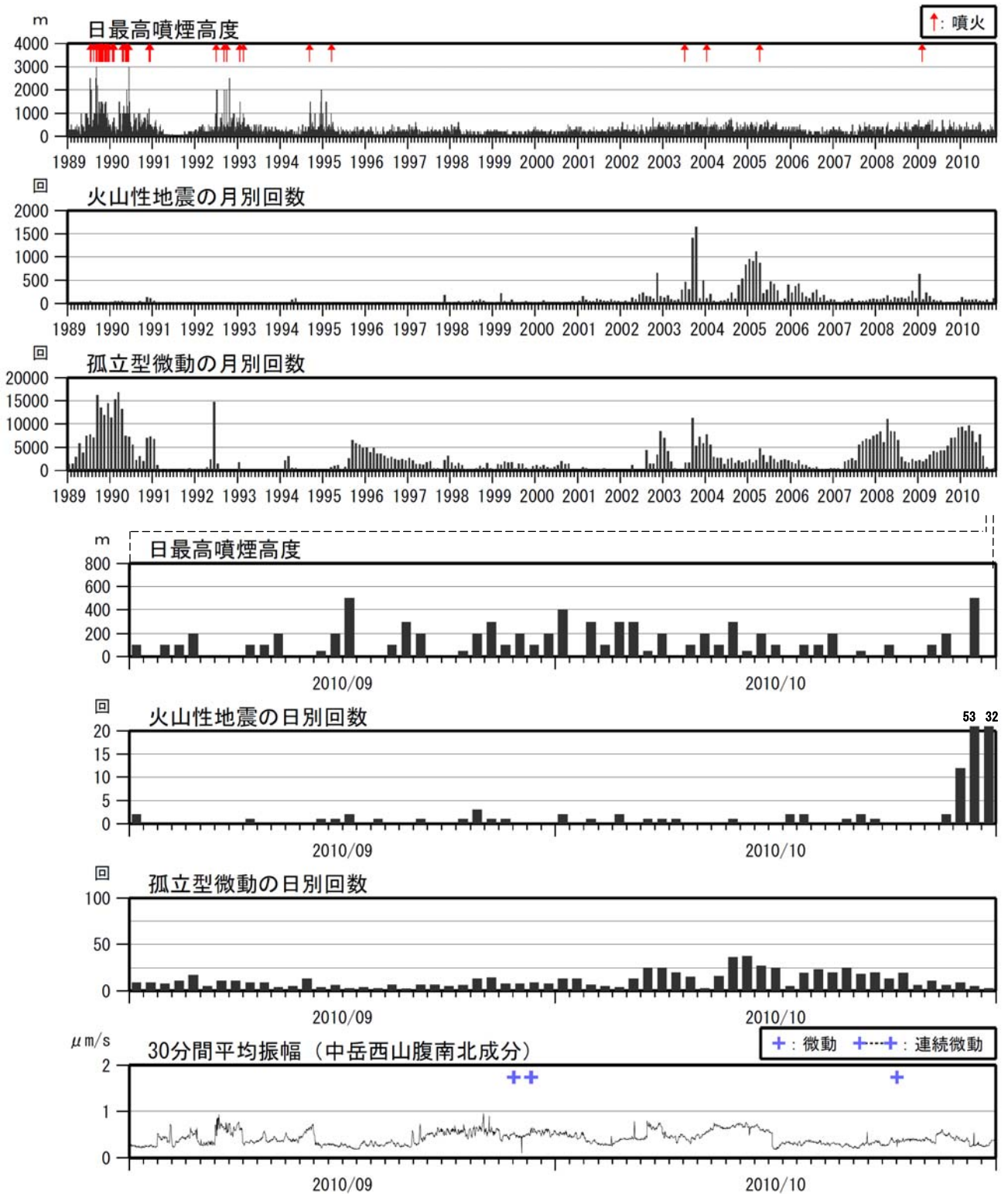
図 2 阿蘇山 噴煙、火山性地震、孤立型微動の状況（1989 年 1 月～2010 年 10 月）
