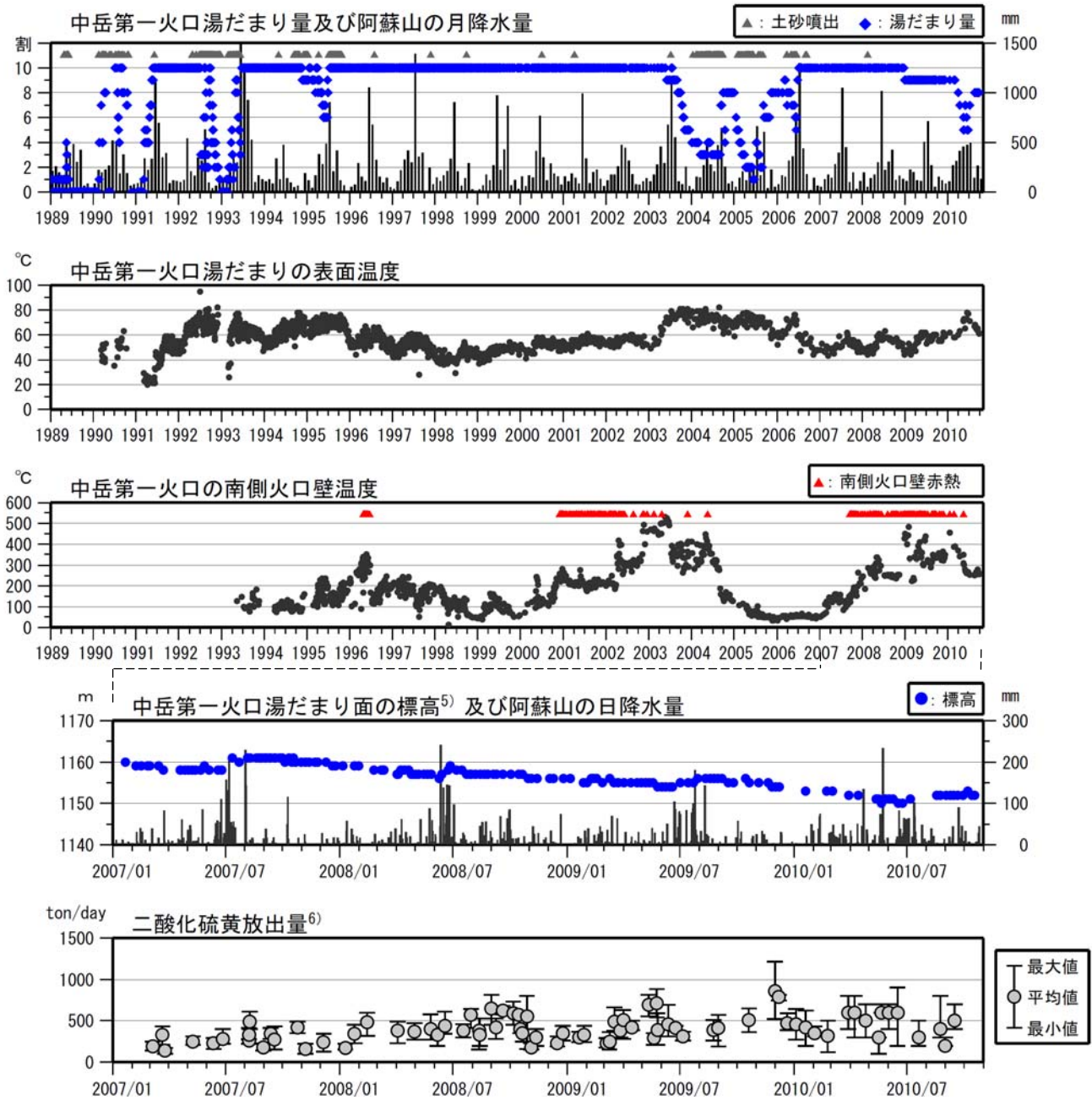
図 3※ 阿蘇山 湯だまり、火口壁、二氧化硫黄放出量の状況（1989 年 1 月～2010 年 10 月） <10 月の状況>
