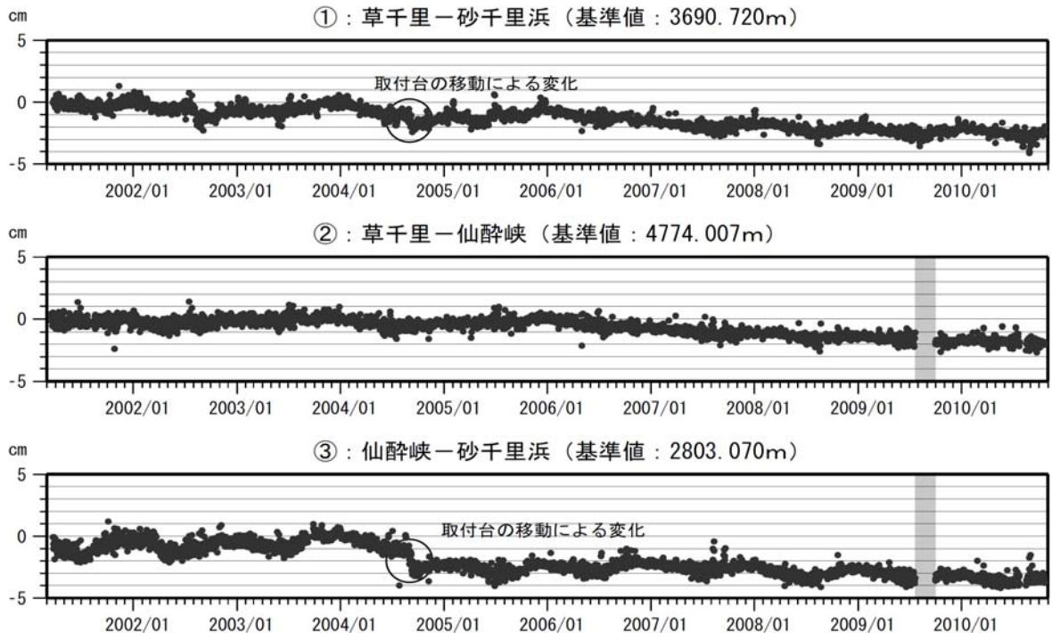
図 5 阿蘇山 GPS連続観測による基線長変化（2001 年 3 月～2010 年 10 月）
