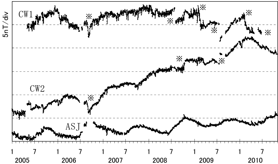
図 7 阿蘇山 全磁力連続観測による阿蘇山麓 (AHK) を基準とした中岳第一火口周辺の全磁力変化 (2005 年 1 月～2010 年 10 月)
