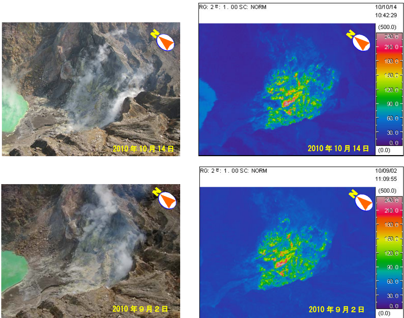
図 8 阿蘇山 赤外熱映像装置 7) による中岳第一火口南側火口壁の地表面温度分布 熱異常域の分布は前期間と比べて特段の変化はありませんでした。
