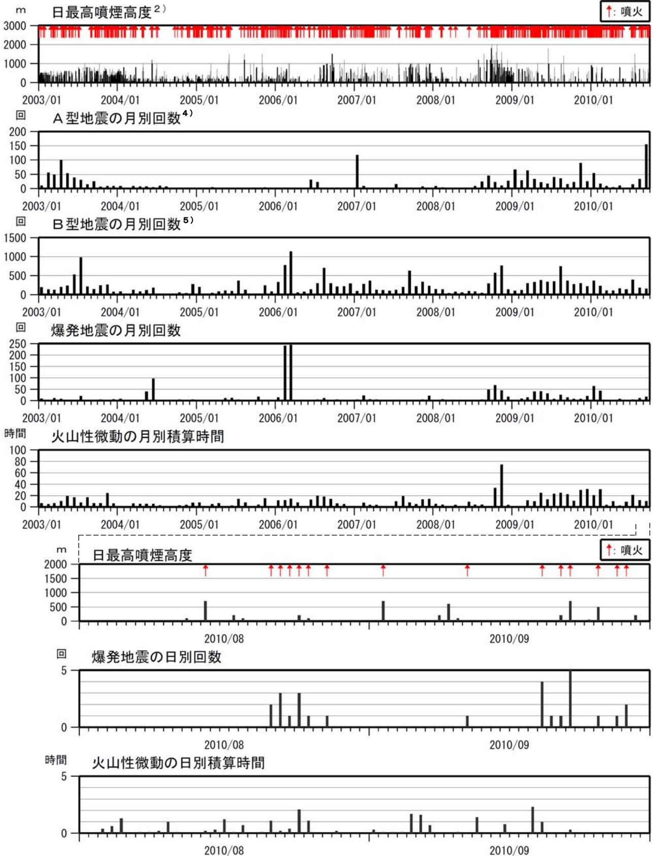
図 1 諏訪之瀬島 火山活動経過図（2003 年 1 月～2010 年 9 月）
