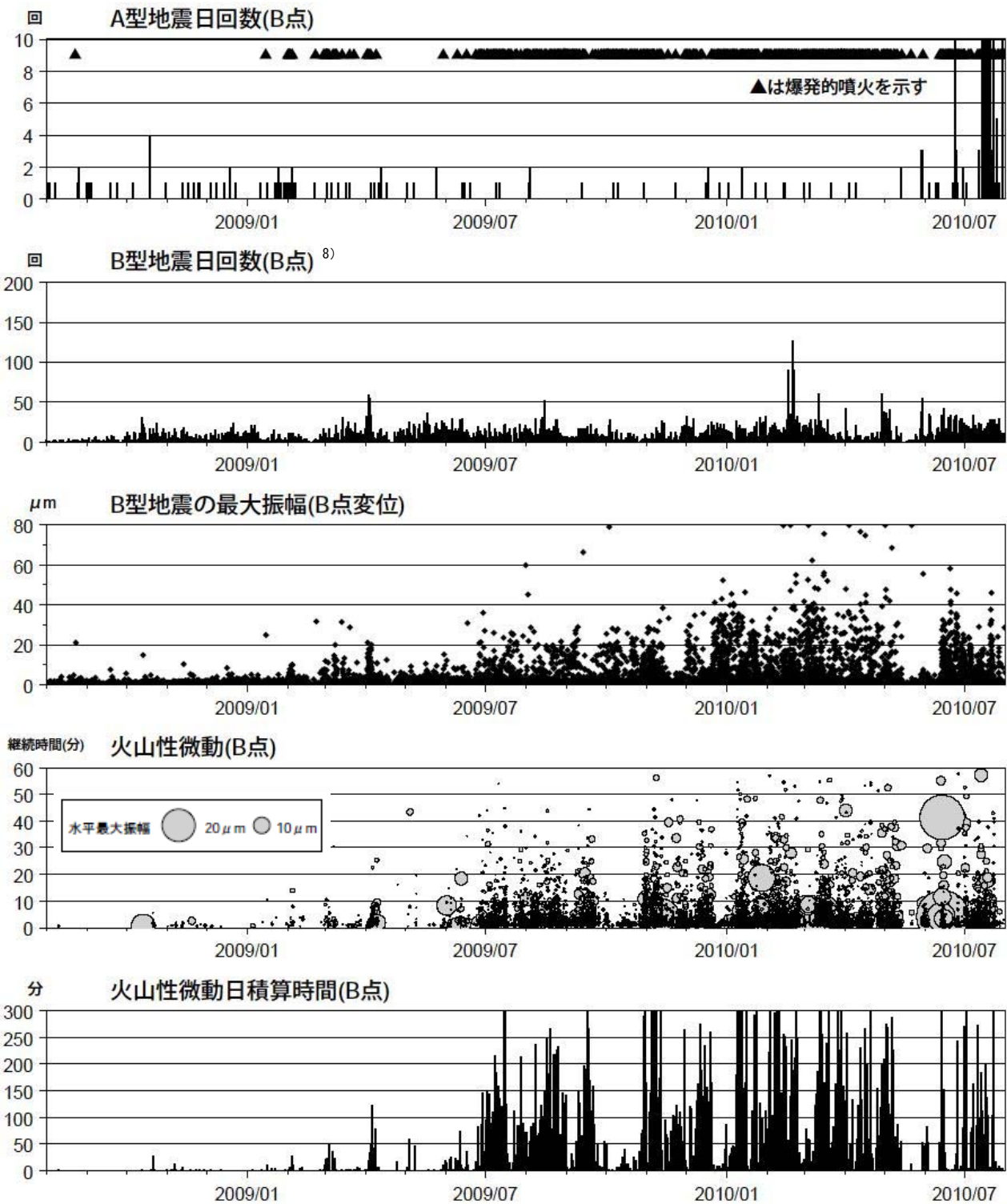
図 3 桜島 最近 2 年間の火山性地震、火山性微動（2008 年 8 月～2010 年 7 月） < 7 月の状況 >
