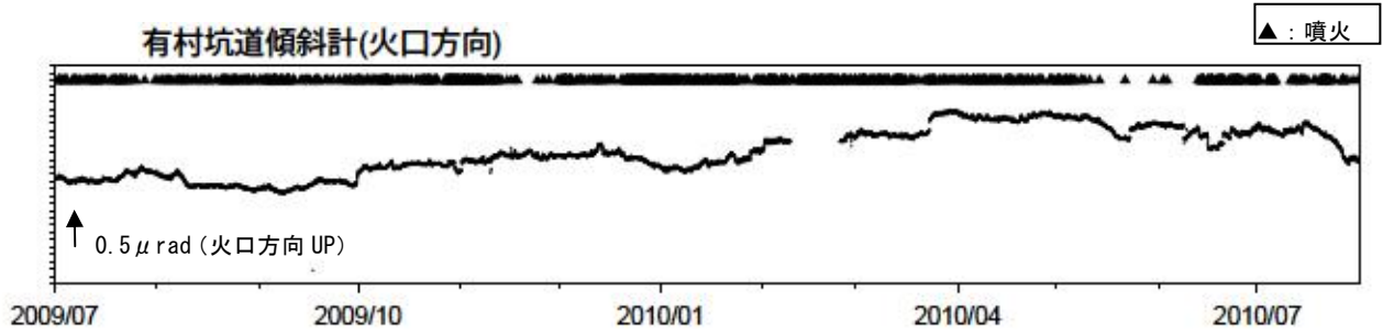
図 5※ 桜島 有村観測坑道の水管傾斜計の変化（2009 年 6 月～2010 年 7 月） < 7 月の状況 >
