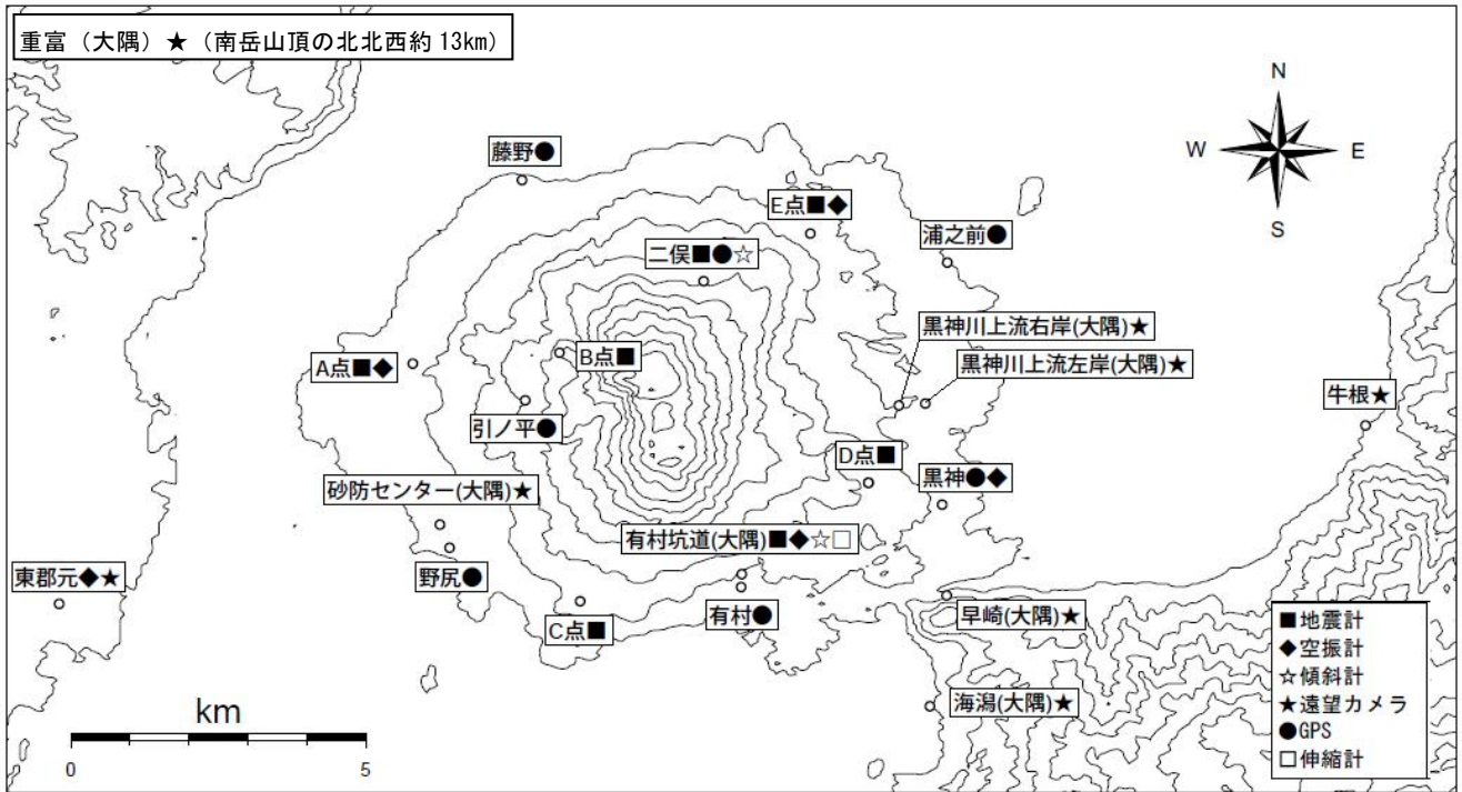
図 11 桜島 観測点配置図 (大隅) : 大隅河川国道事務所設置
