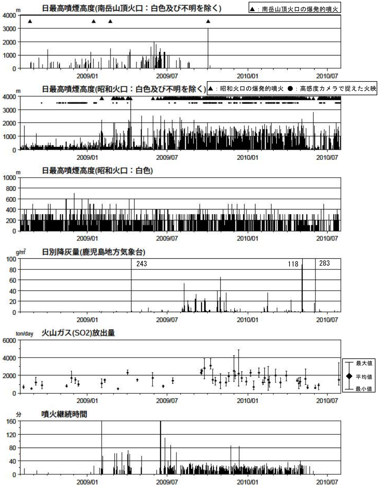
図2 桜島 最近2年間の噴煙、降灰、火山ガス（2008年8月～2010年7月）
