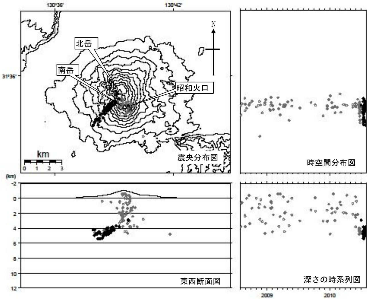
● : 2010 年 7 月の震源 ○ : 2008 年 8 月～2010 年 6 月の震源 図 4※ 桜島 震源分布図（2008 年 8 月～2010 年 7 月）
