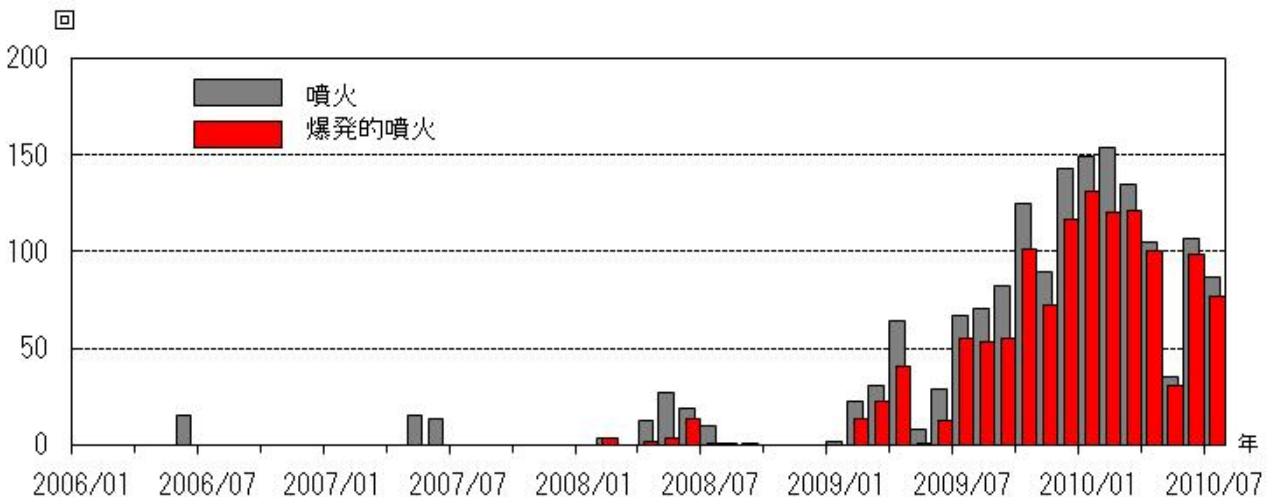
図 1 桜島 昭和火口月別噴火回数（灰色）と昭和火口月別爆発回数（赤色）
