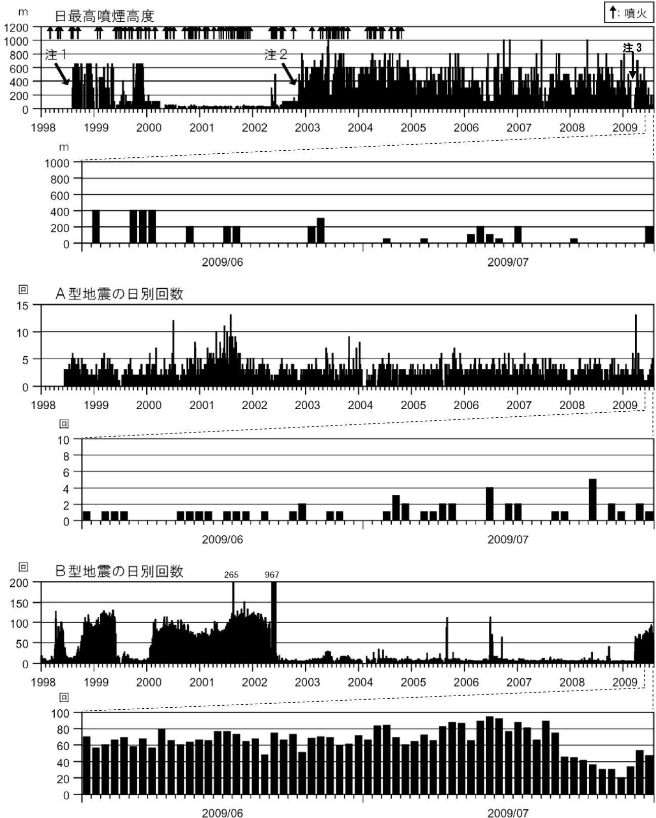
図2 薩摩硫黄島 火山活動経過図（1998年1月～2009年7月）
