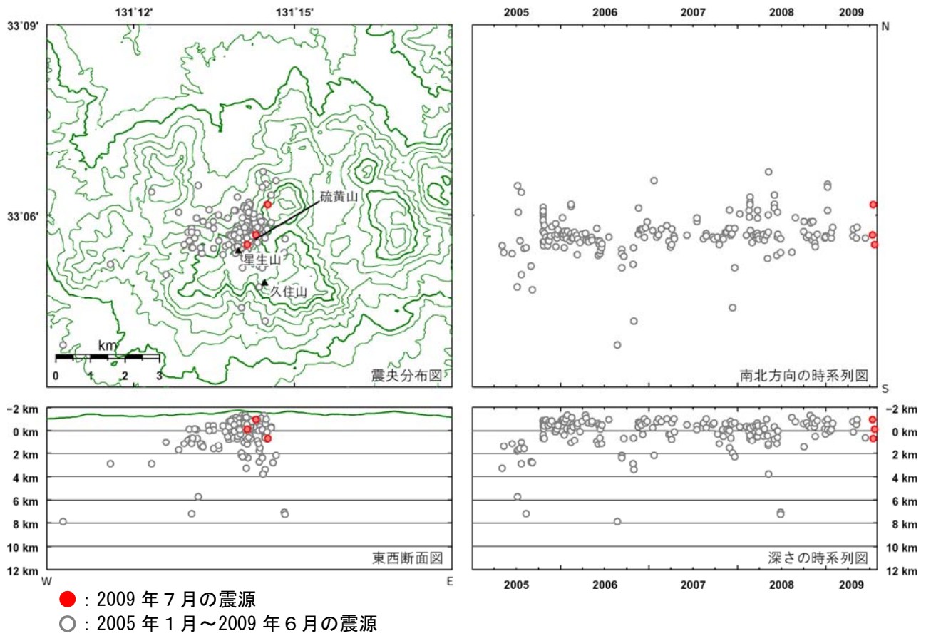
図 4 ※ 九重山 震源分布図（2005 年 1 月～2009 年 7 月）
