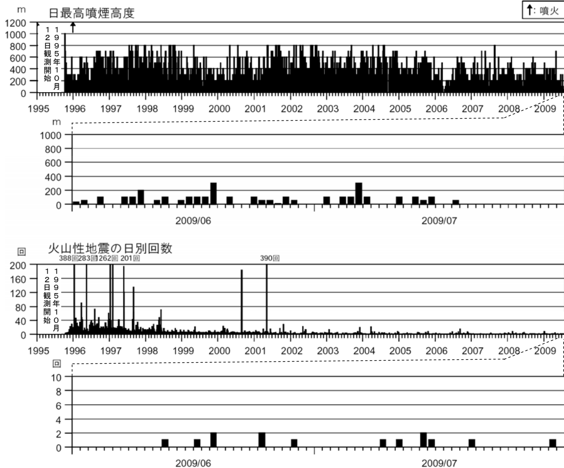
図 2 九重山 火山活動経過図（1995 年 10 月～2009 年 7 月）
