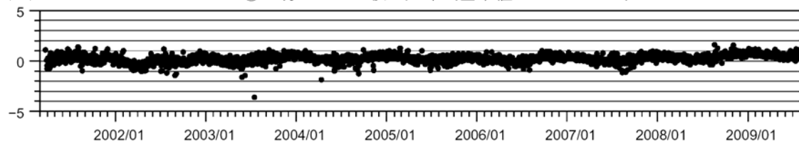
図 3 九重山 GPS 連続観測による基線長変化（2001 年 3 月～2009 年 7 月）
