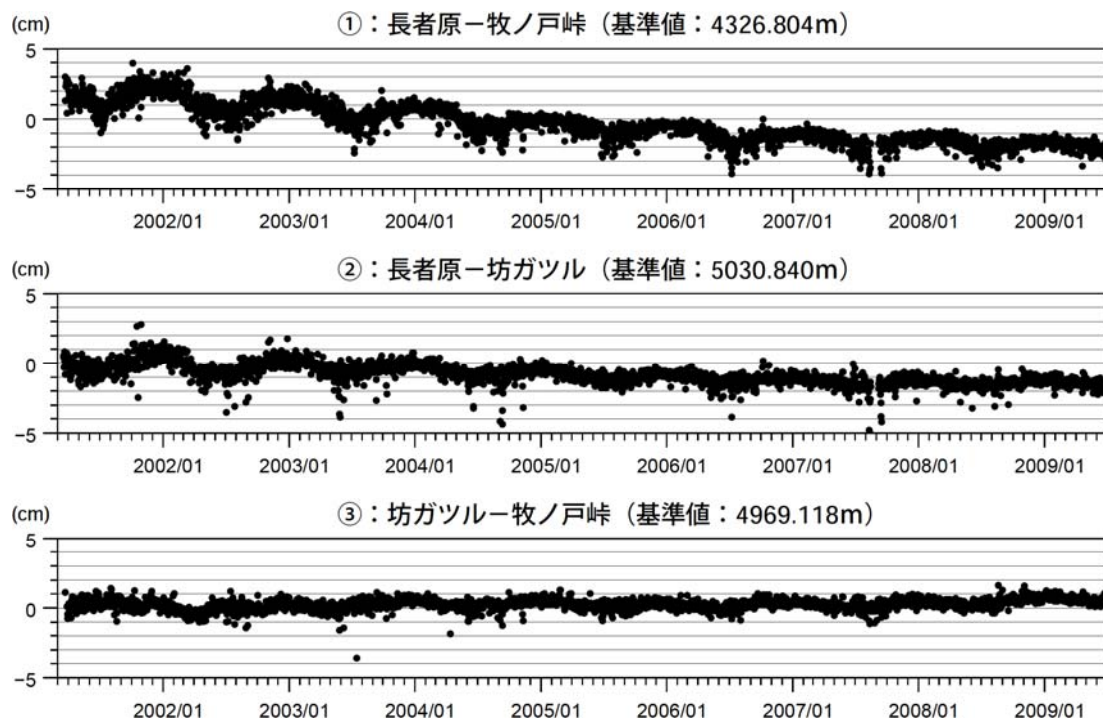
図 3 九重山 GPS 連続観測による基線長変化（2001 年 3 月～2009 年 6 月）
