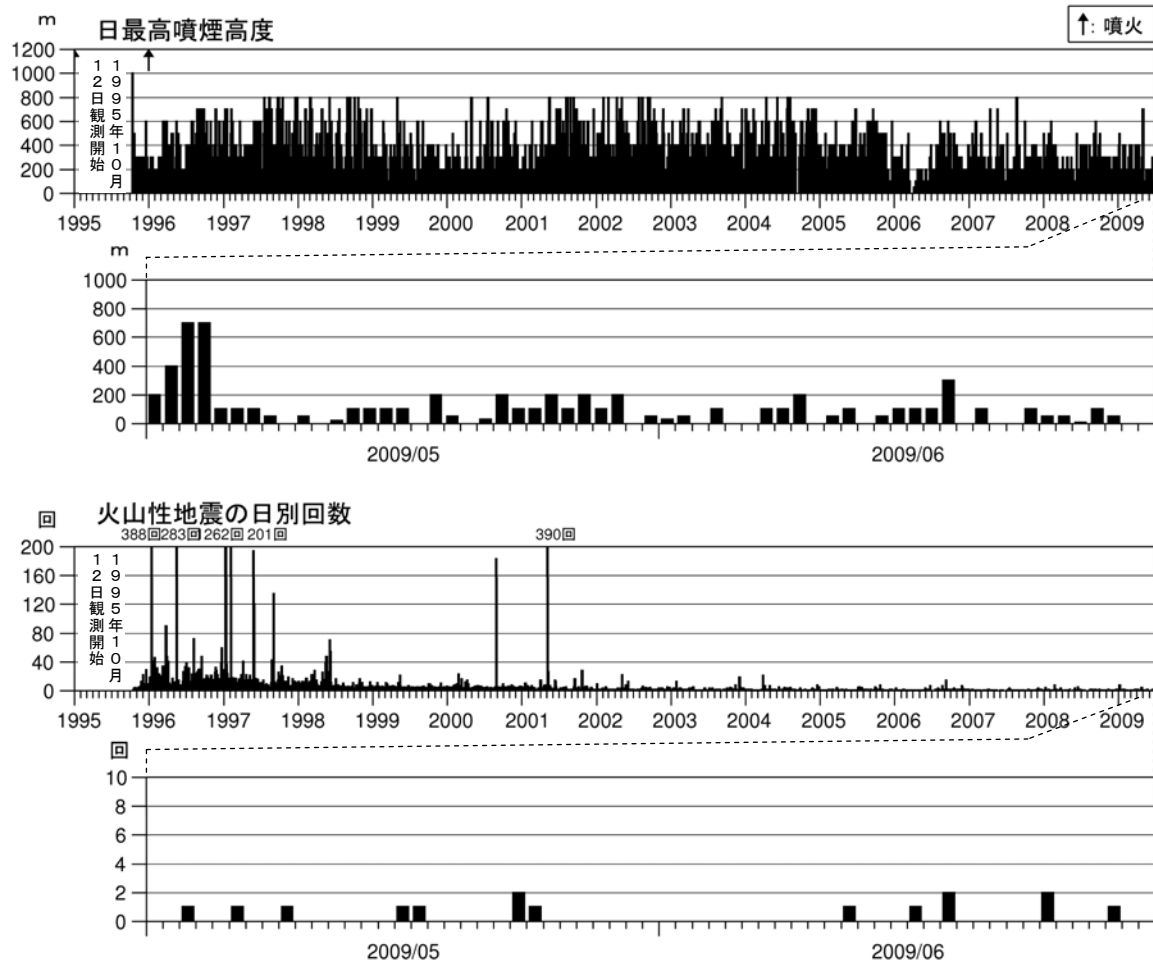
図 2 九重山 火山活動経過図（1995 年 10 月～2009 年 6 月）
