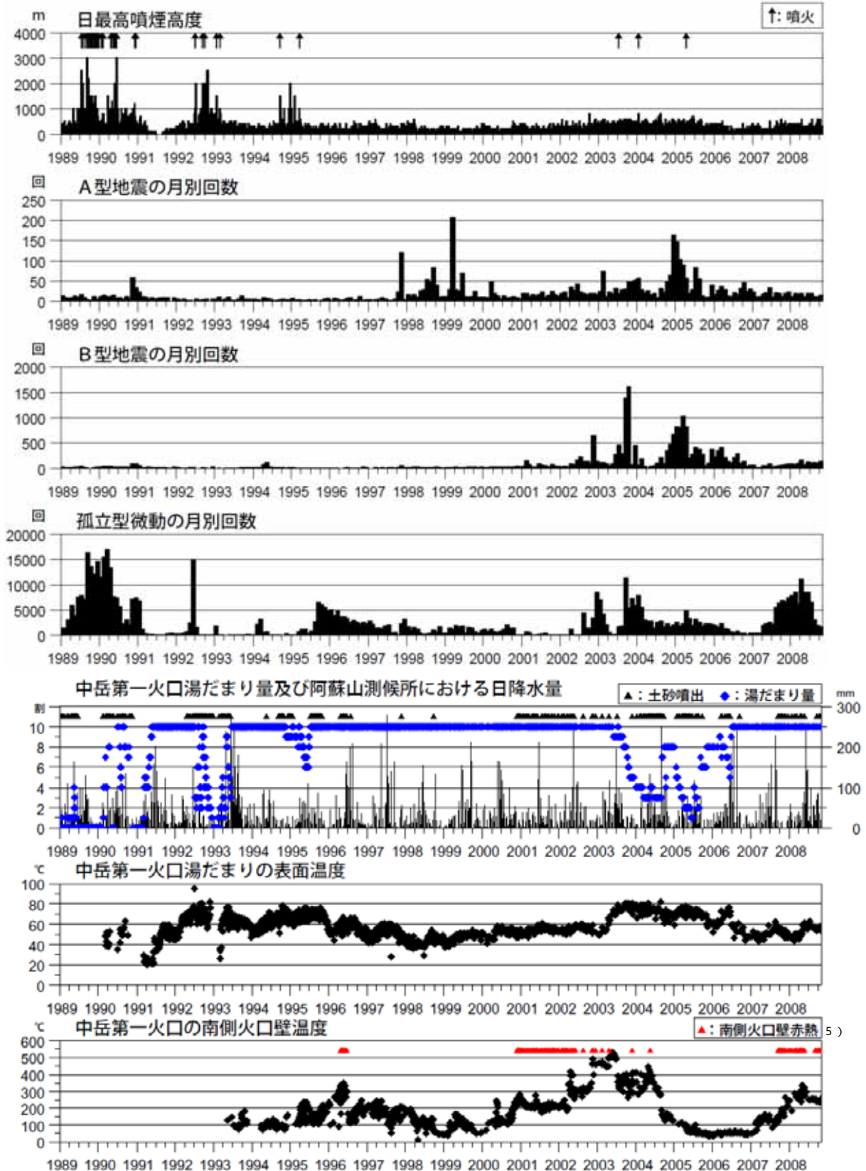
図2 阿蘇山 火山活動経過図(1989年1月～2008年10月)
