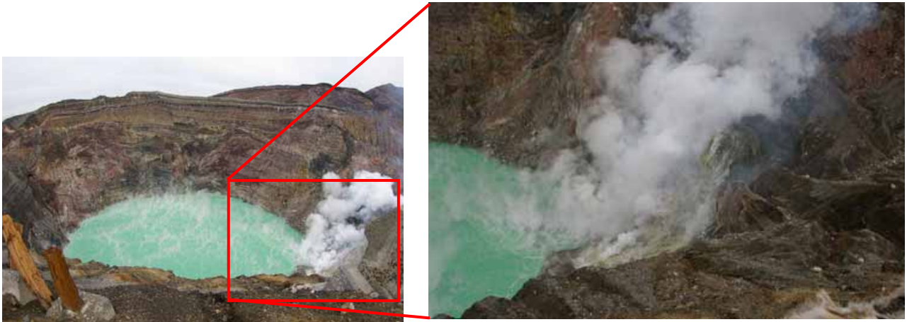
図9 阿蘇山 中岳第一火口の状況 (2008年10月30日、南西側より撮影) 湯だまりの色は緑色で、湯だまりの量は10割でした。
