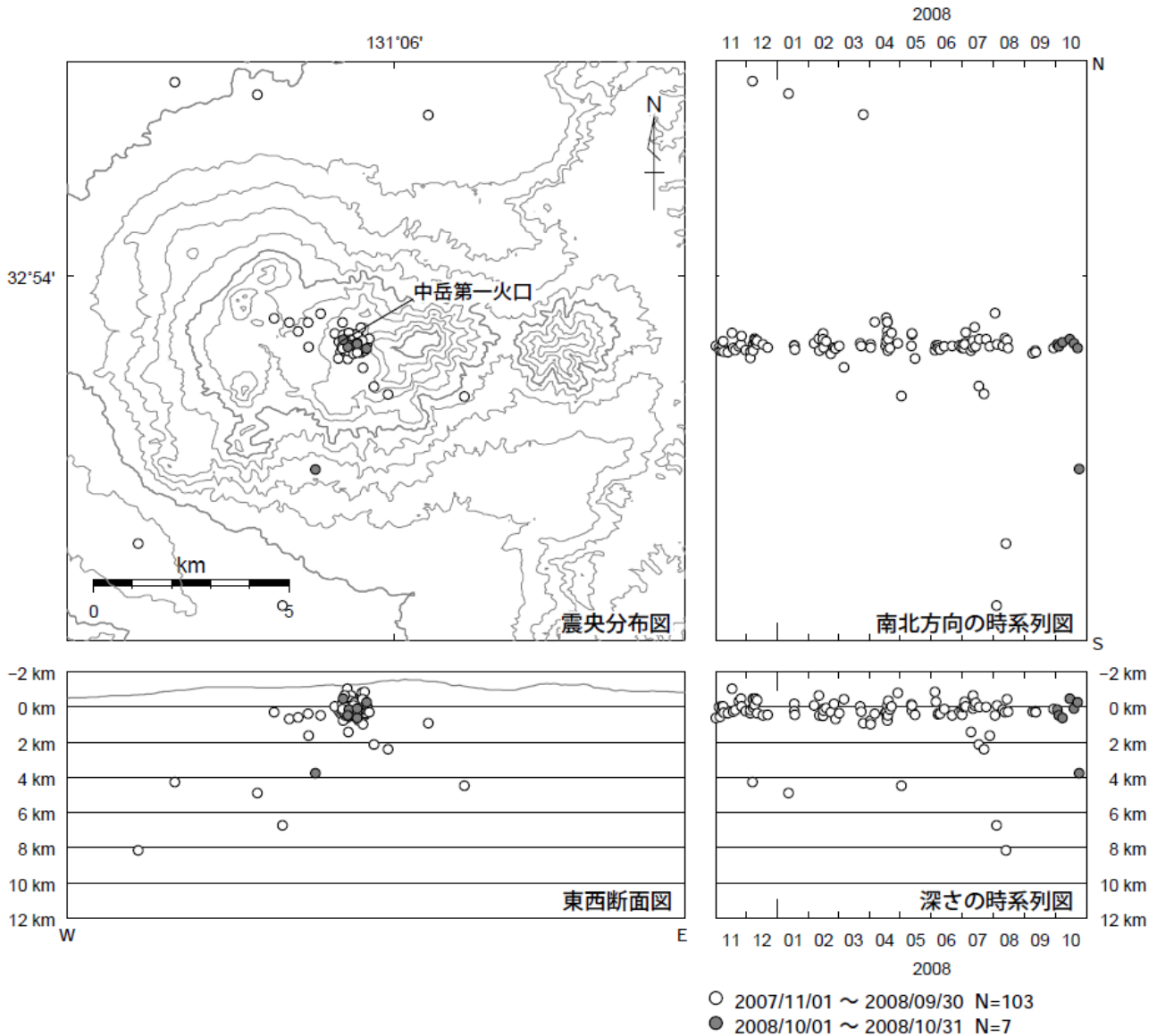
図1 阿蘇山 震源分布図(2007年11月~2008年10月)
