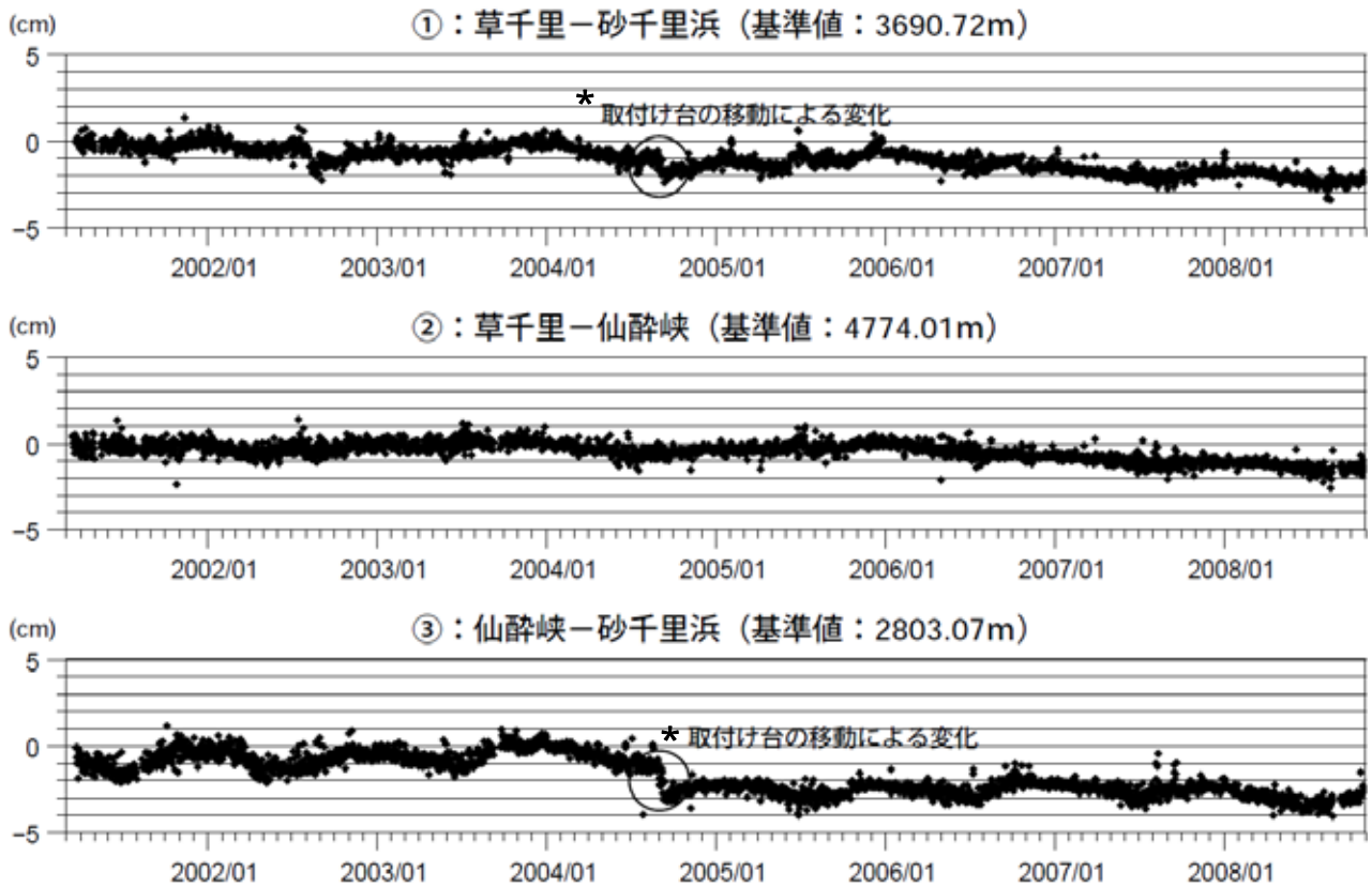
図5 阿蘇山 GPS連続観測による基線長変化(2001年3月15日~2008年10月31日)
