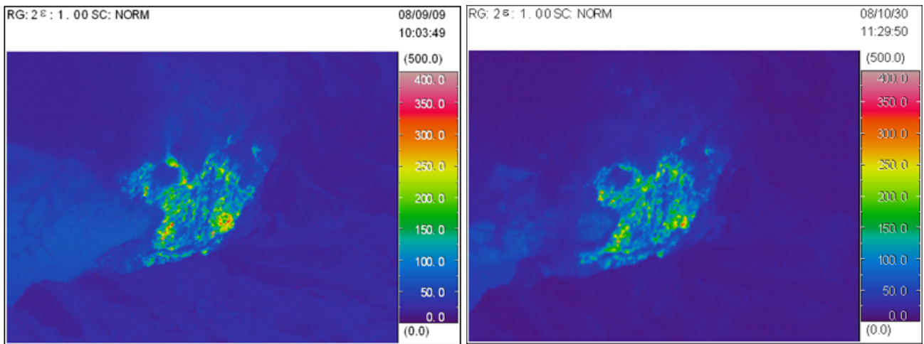
図9 阿蘇山 中岳第一火口の状況 (2008年10月30日、南西側より撮影) 湯だまりの色は緑色で、湯だまりの量は10割でした。
