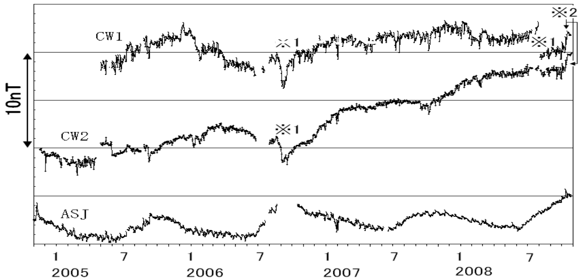
図8 阿蘇山 阿蘇山麓(AHK)を基準とした阿蘇中岳火口周辺の全磁力変化 (2004年11月~2008年10月)
