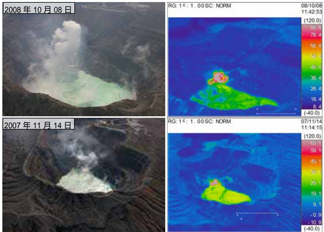
図11 阿蘇山 阿蘇中岳第一火口 陸上自衛隊第8師団の協力により北側から撮影 (左:可視、右:熱画像)
