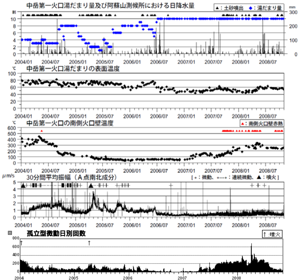
図3 阿蘇山 火山活動経過図(2004年1月~2008年10月)
