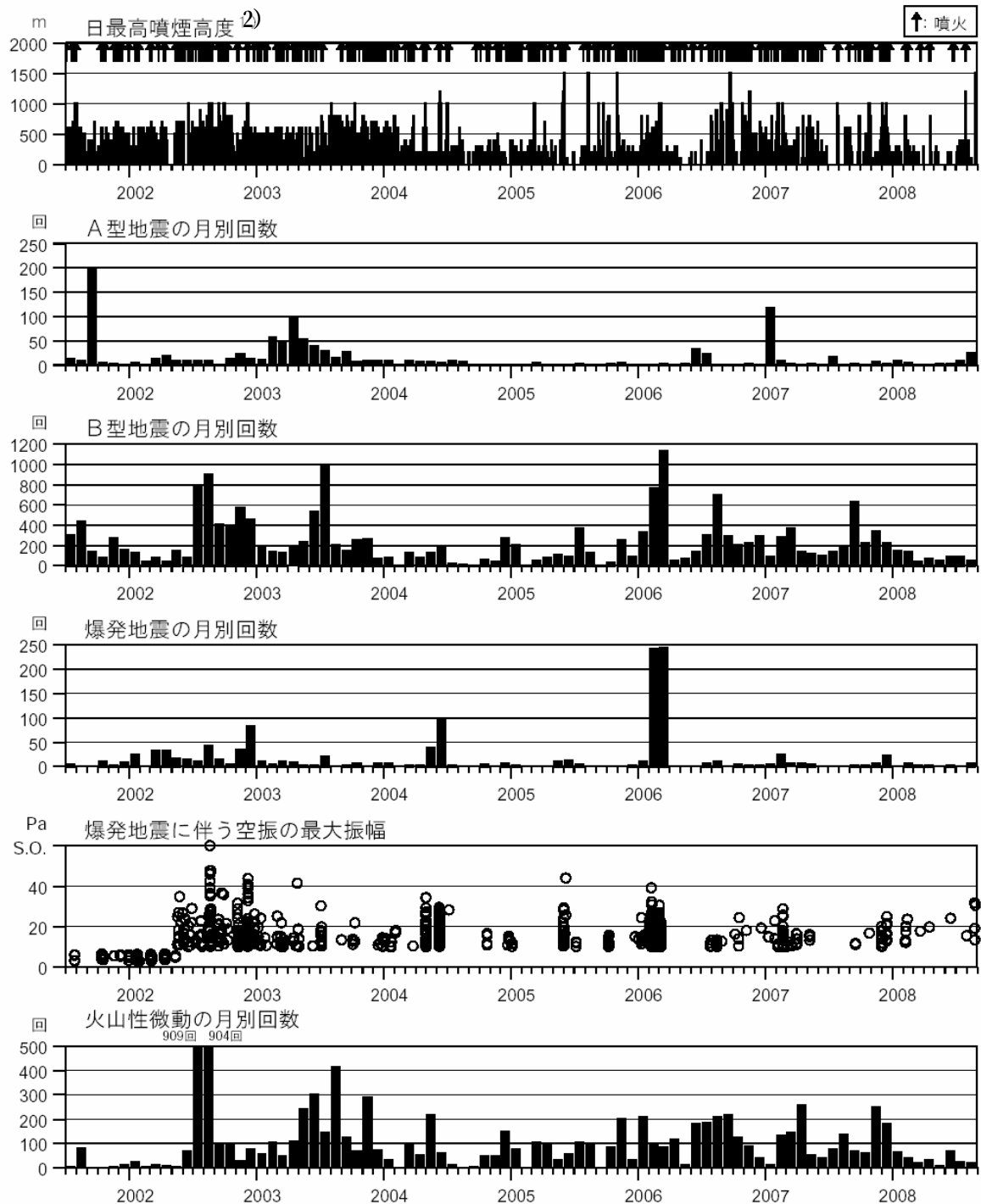
図2 諏訪之瀬島 火山活動経過図(2001年7月～2008年8月)
