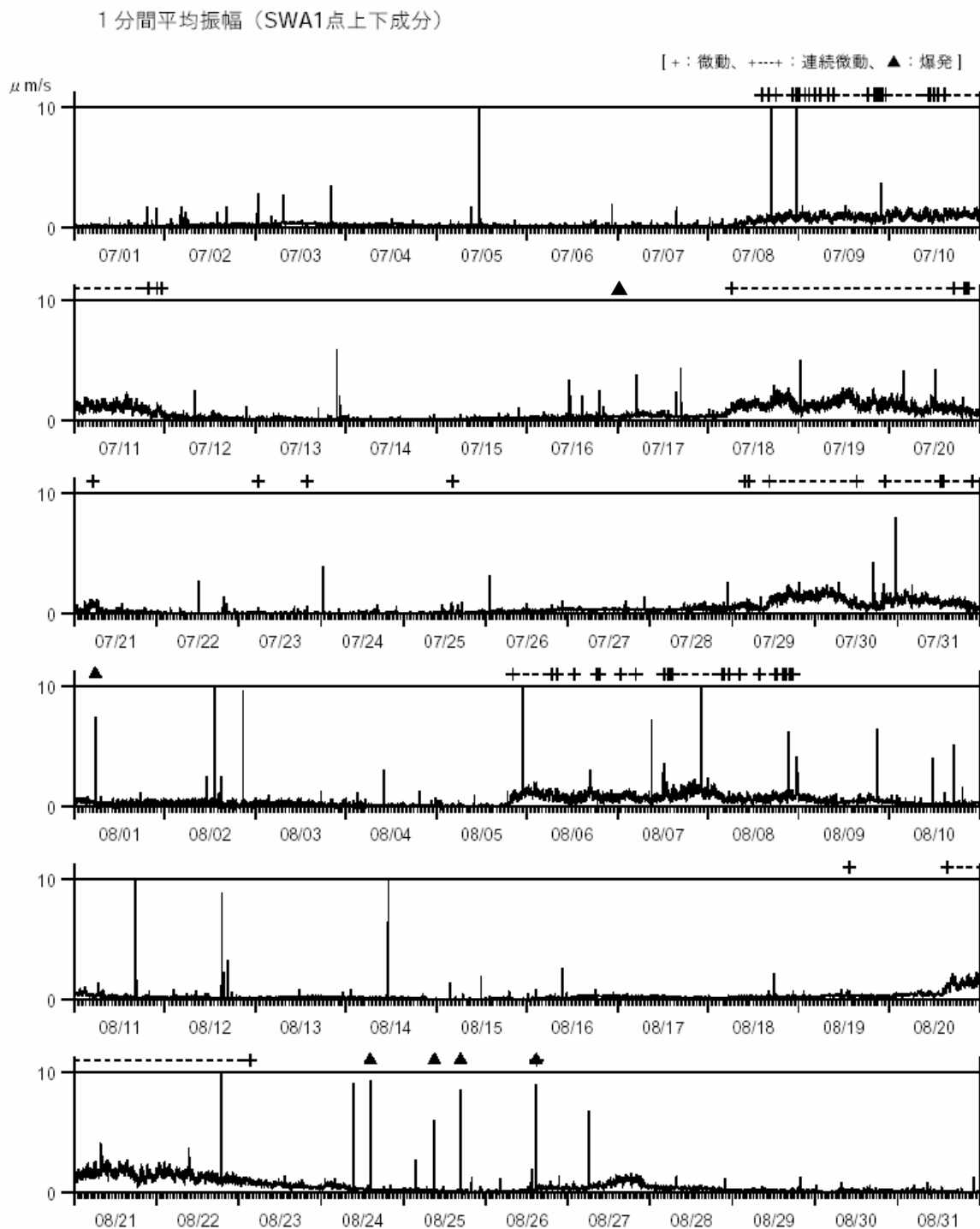
図3 諏訪之瀬島 1分間平均振幅の時間変化（SWA1上下成分）（2008年7月～2008年8月）
