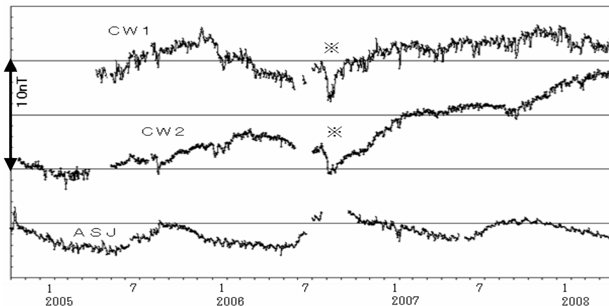
図 8 阿蘇山 阿蘇中岳火口周辺の全磁力変化（2004 年 11 月～2008 年 4 月）
