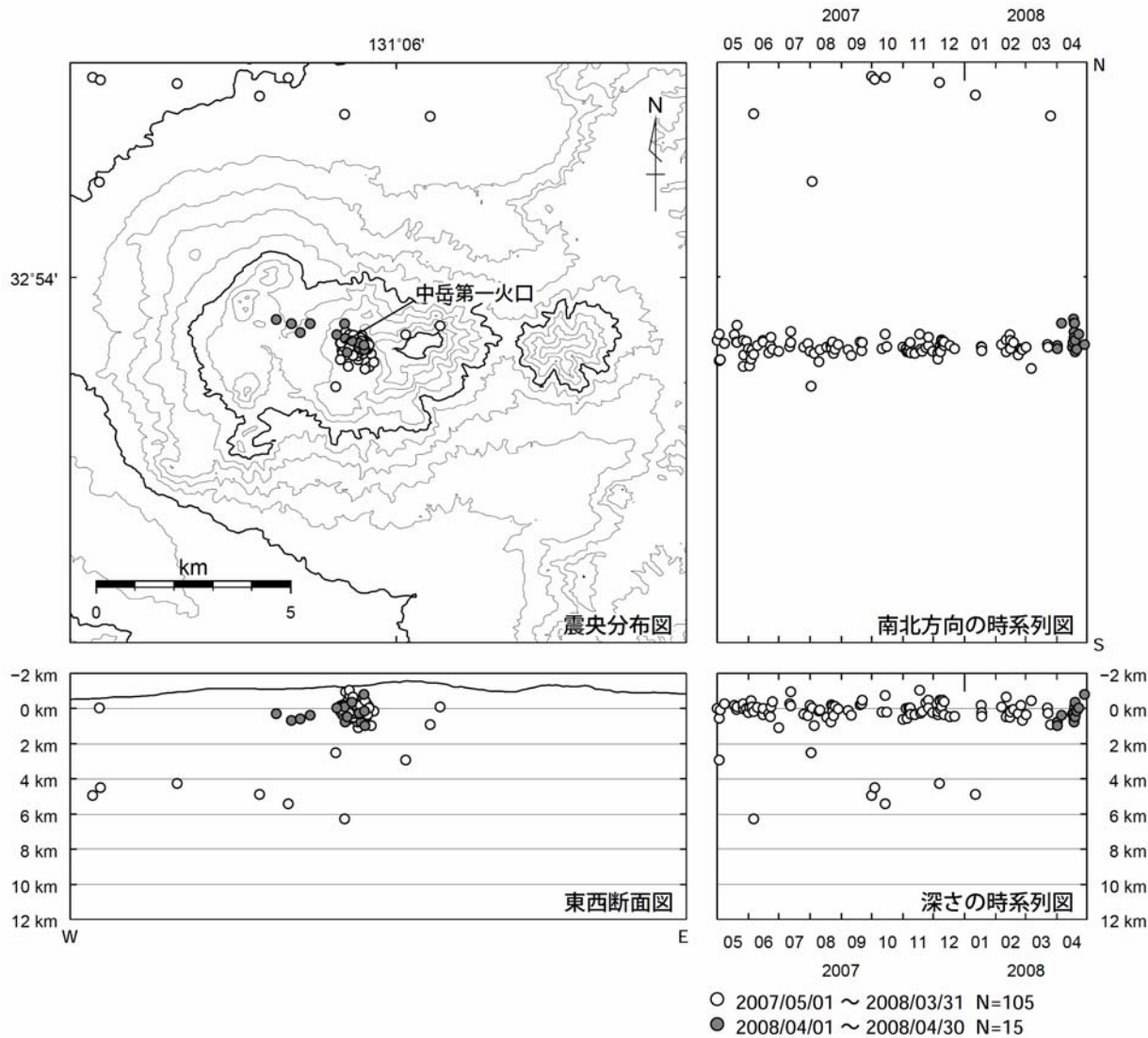
図 1 ※ 阿蘇山 震源分布図(2007 年 5 月～2008 年 4 月)
