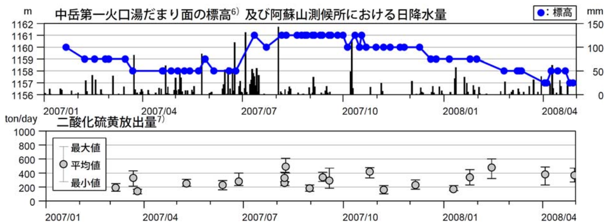
図4 阿蘇山 火山活動経過図(2007年1月～2008年4月)
