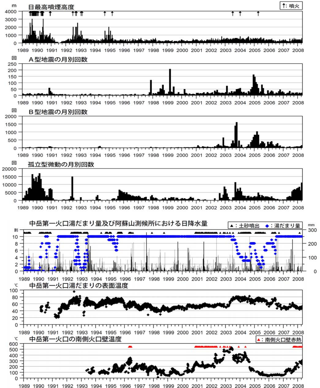
図2 阿蘇山 火山活動経過図(1989年1月～2008年4月)
