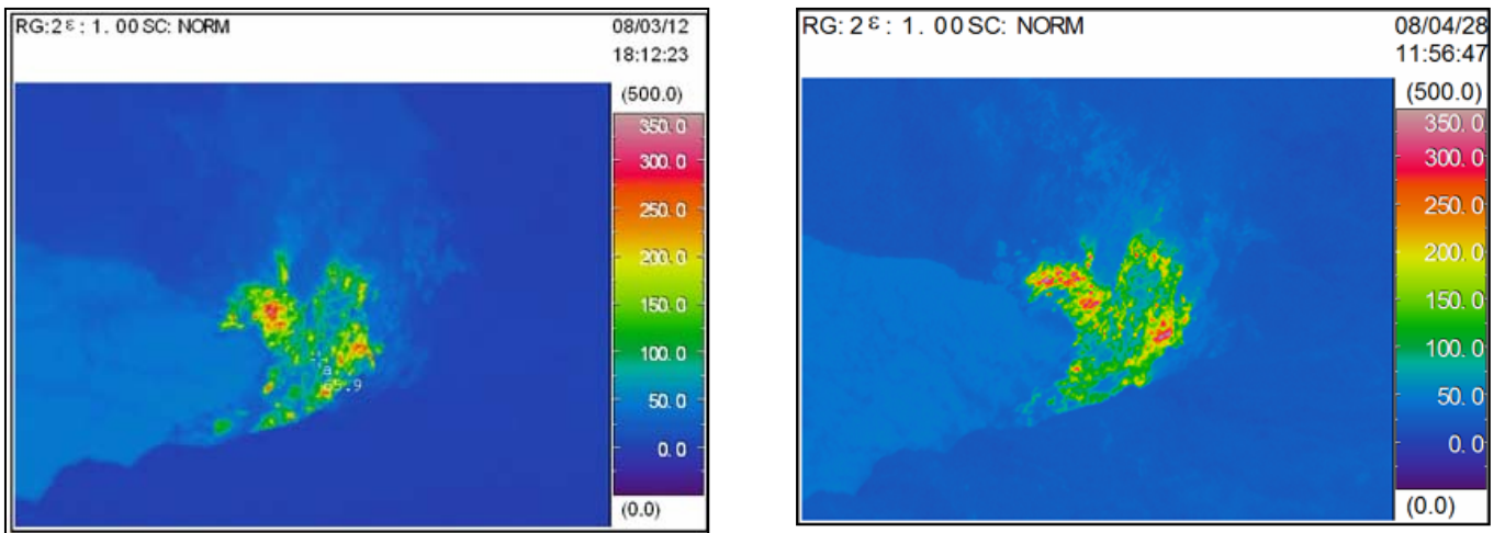
図 10 阿蘇山 中岳第一火口南側火口壁の状況（左:2008 年 3 月 12 日、右:2008 年 4 月 28 日南西側より撮影） ・赤外熱映像装置 8) では熱領域の拡がりに大きな変化はありません。
