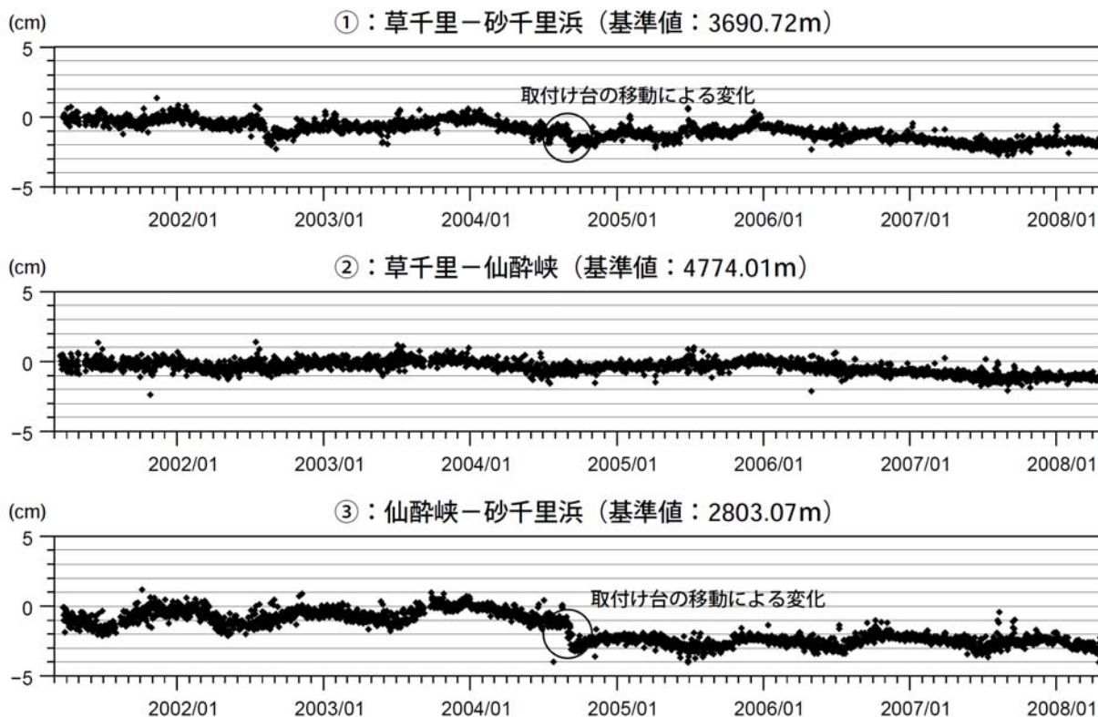
図 5 阿蘇山 GPS 連続観測による基線長変化(2001 年 3 月 15 日～2008 年 4 月 30 日)
