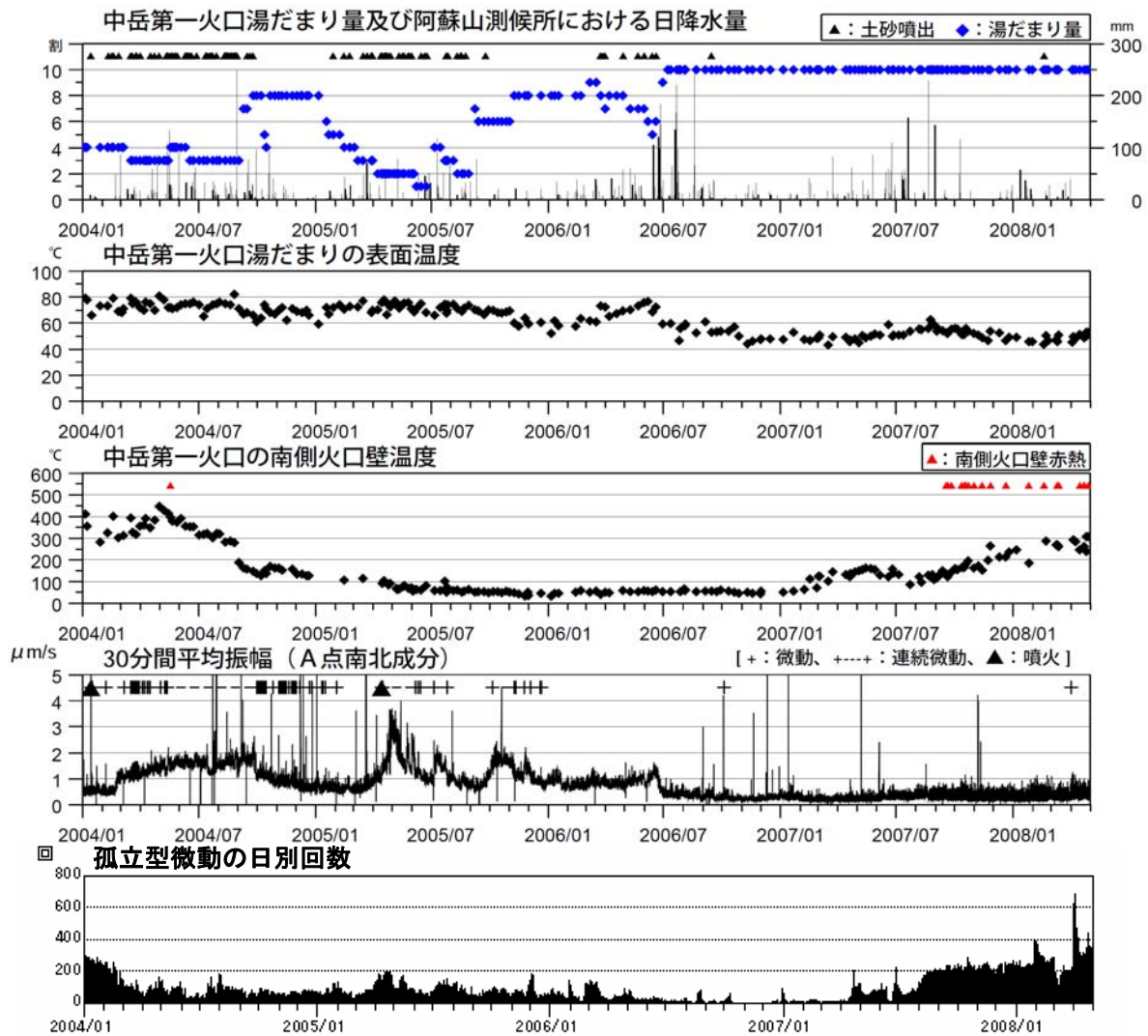
図3 阿蘇山 火山活動経過図(2004年1月～2008年4月)
