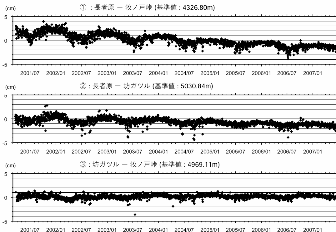
図4 九重山 GPS 連続観測による基線長変化(2001 年 3 月 1 日～2007 年 6 月 30 日) GPS による連続観測では、長者原—牧ノ戸峠の基線長は、1995 年から 1996 年の噴火後の火山ガスの放出に伴うと考えられる長期的な縮みの傾向が見えます。
