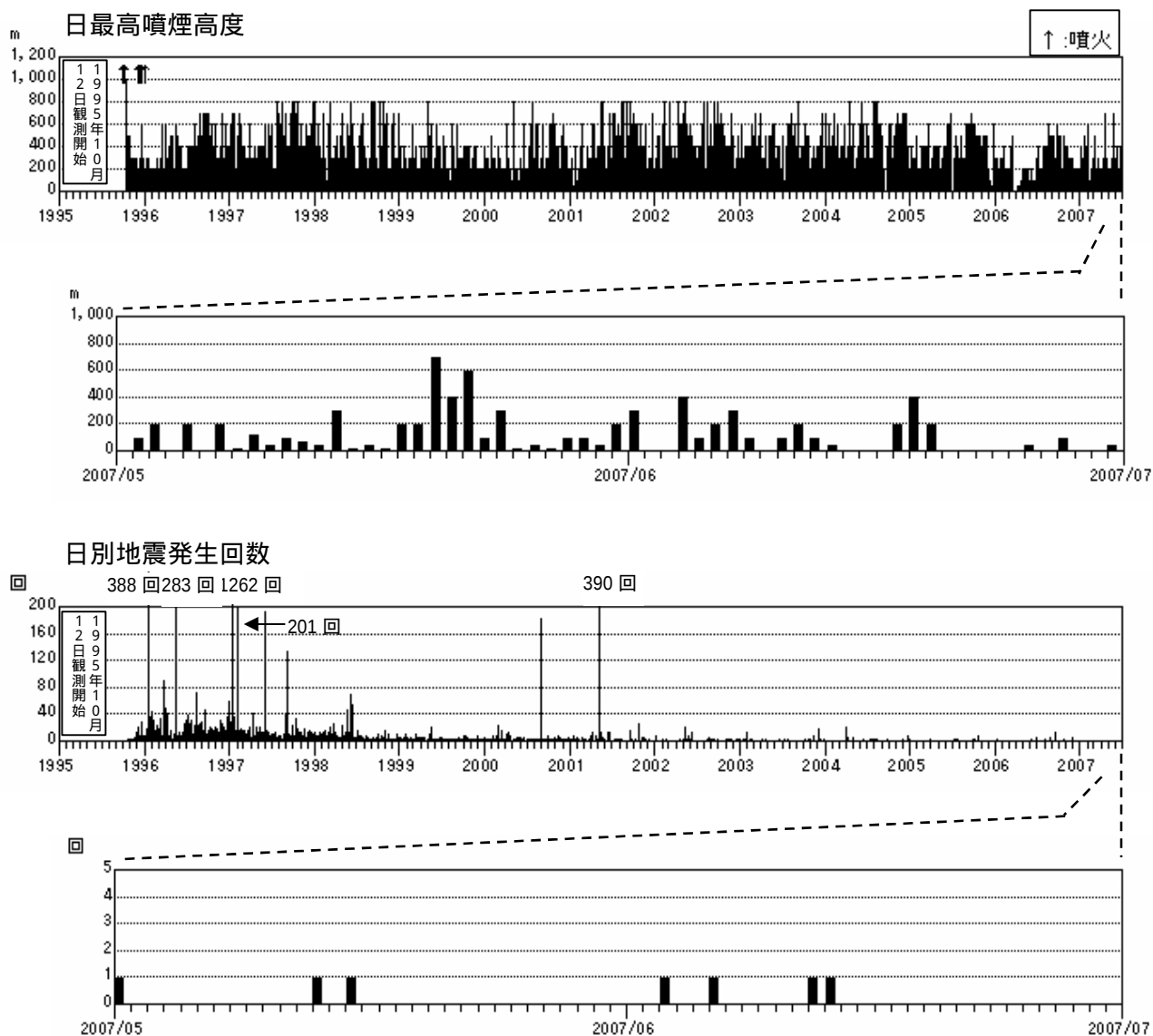
図 2 九重山 火山活動経過図(1995 年 10 月 12 日～2007 年 6 月 30 日)
