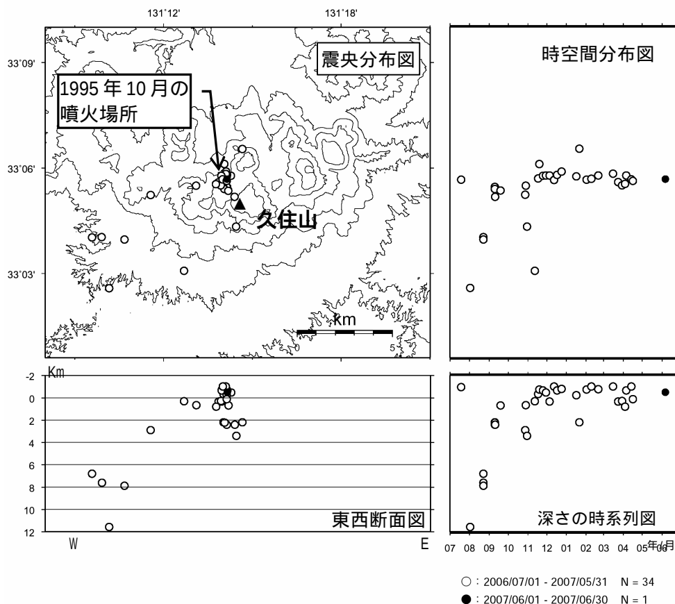
図3 九重山 震源分布図(2006 年 7 月 1 日～2007 年 6 月 30 日) 2007 年 6 月は山体付近の浅いところに 1 個震源が決まりました。
