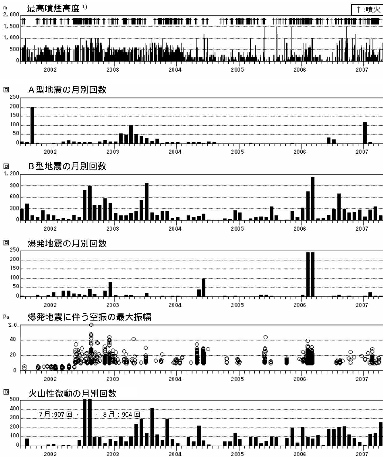
図 2 諏訪之瀬島 火山活動経過図(2001 年 7 月～2007 年 4 月)
