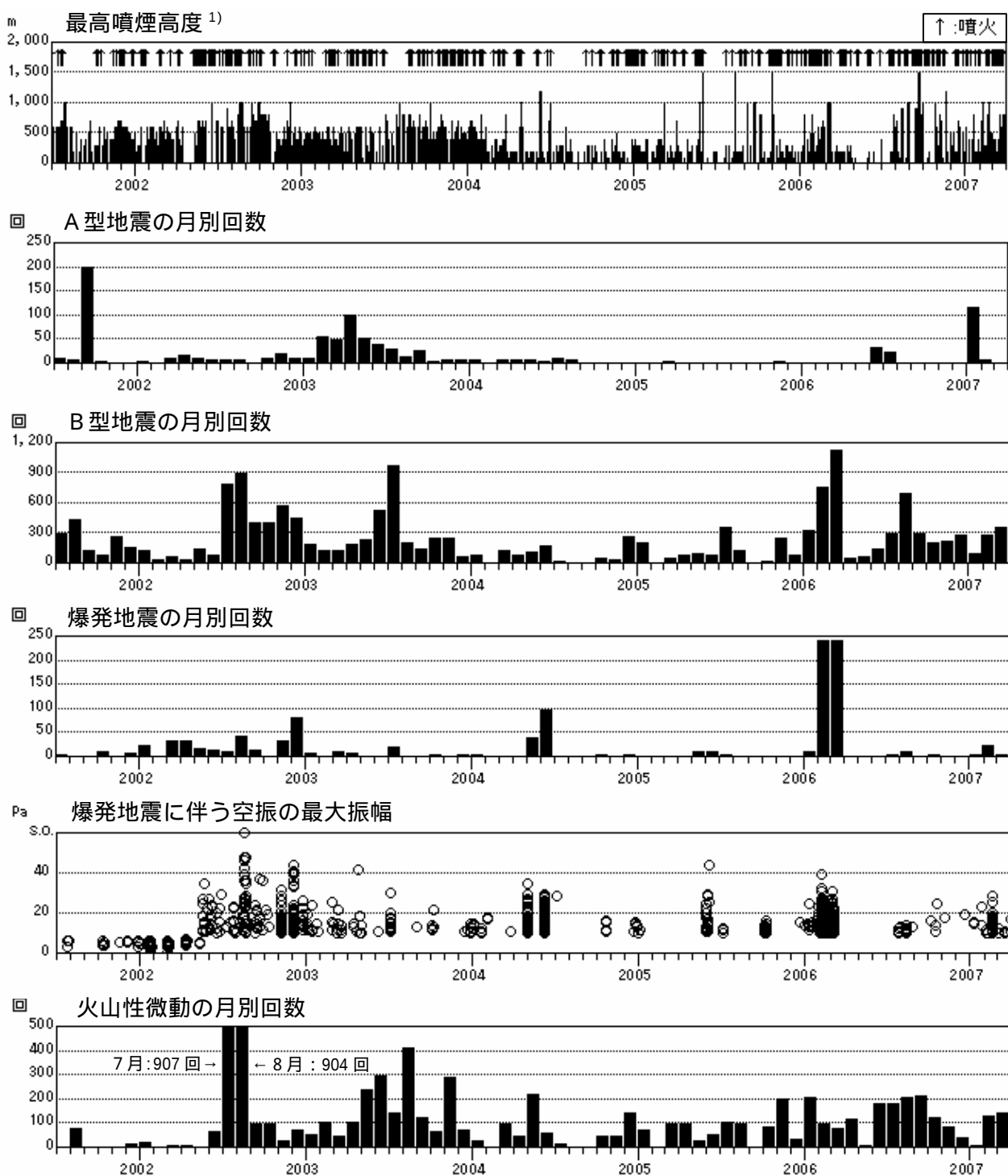
図 2 諏訪之瀬島 火山活動経過図(2001 年 7 月～2007 年 3 月)
