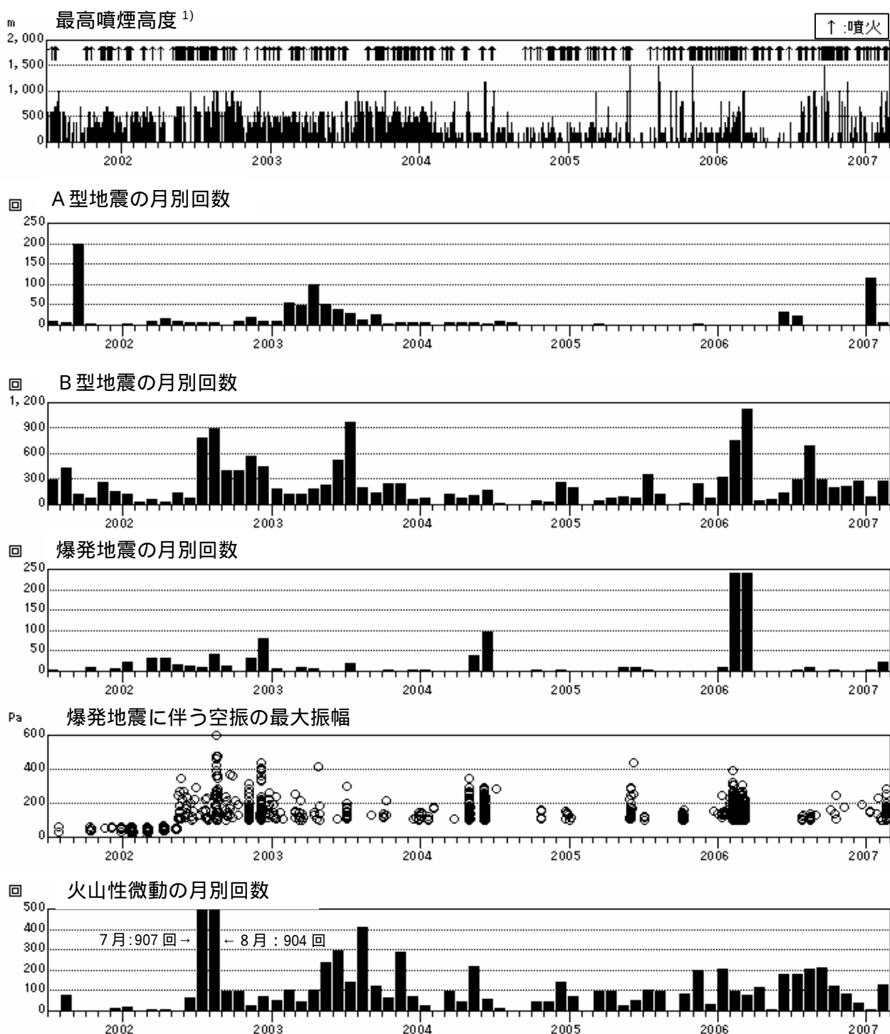
図 2 諏訪之瀬島 火山活動経過図(2001 年 7 月～2007 年 2 月)
