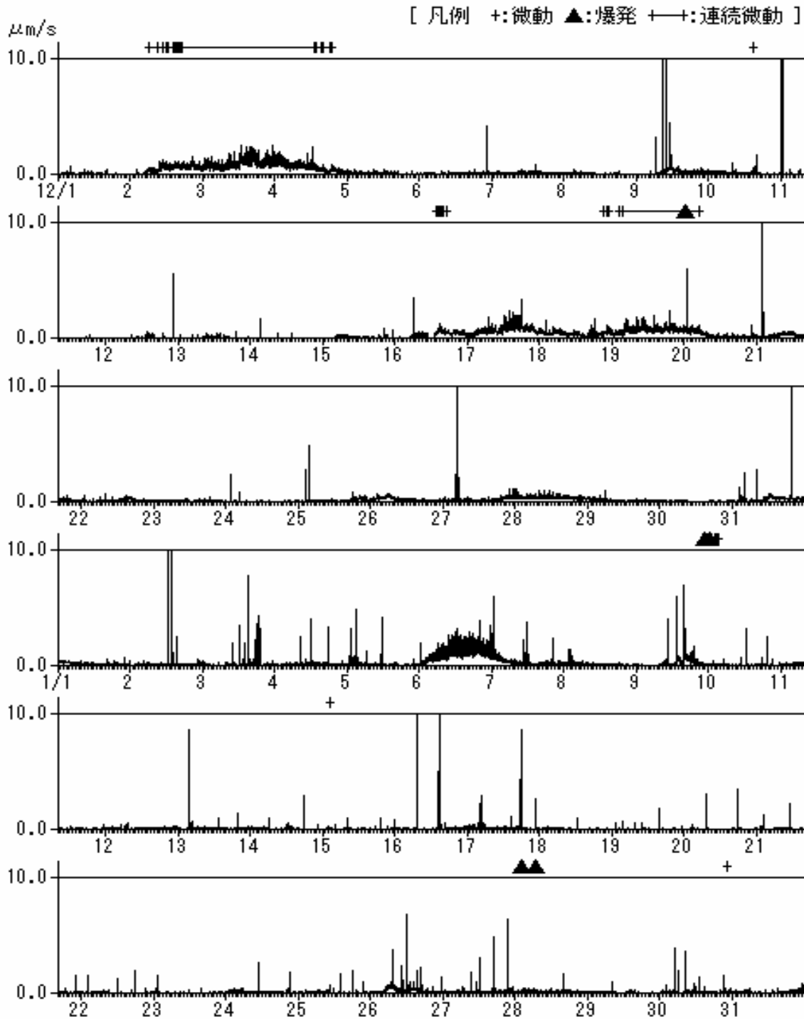
図3 1分間平均振幅の時間変化（SWA1 上下成分） （2006 年 12 月 1 日～2007 年 1 月 31 日）
