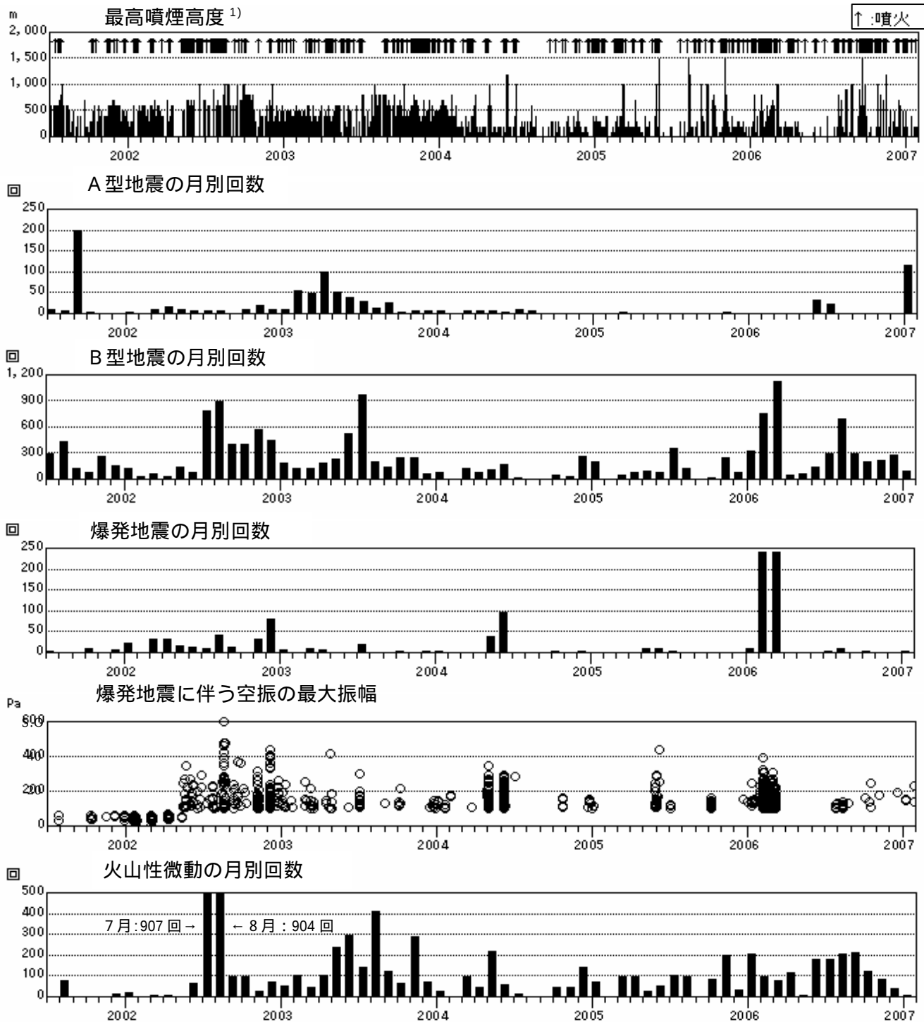
図 2 火山活動経過図(2001 年 7 月～2007 年 1 月)
