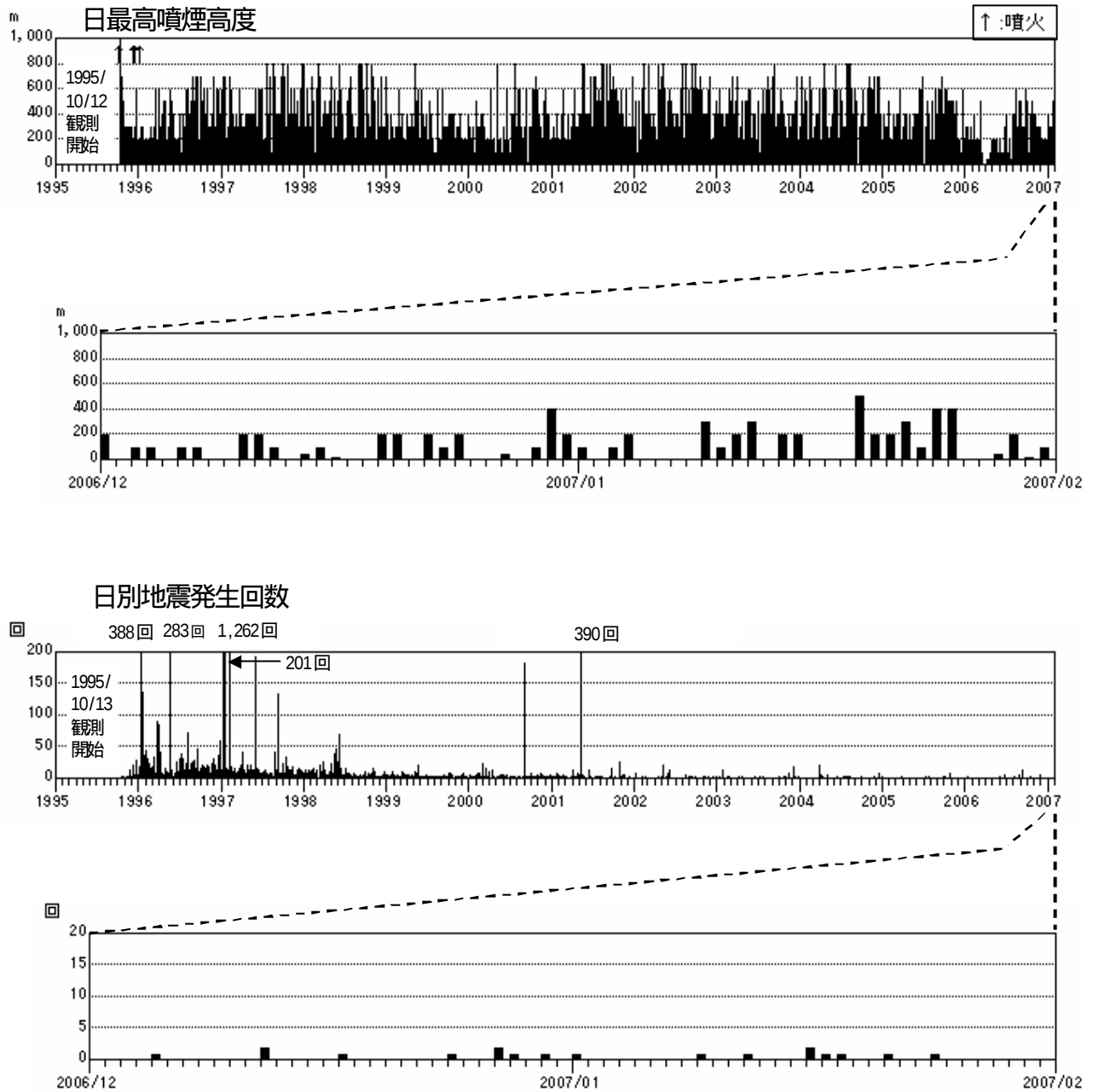
図2 火山活動経過図(1995年10月12日～2007年1月31日)
