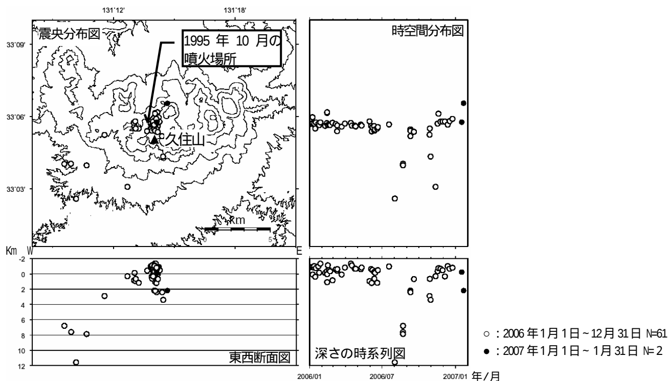
図3 火山性地震の震源分布図(2006年1月1日～2007年1月31日)
