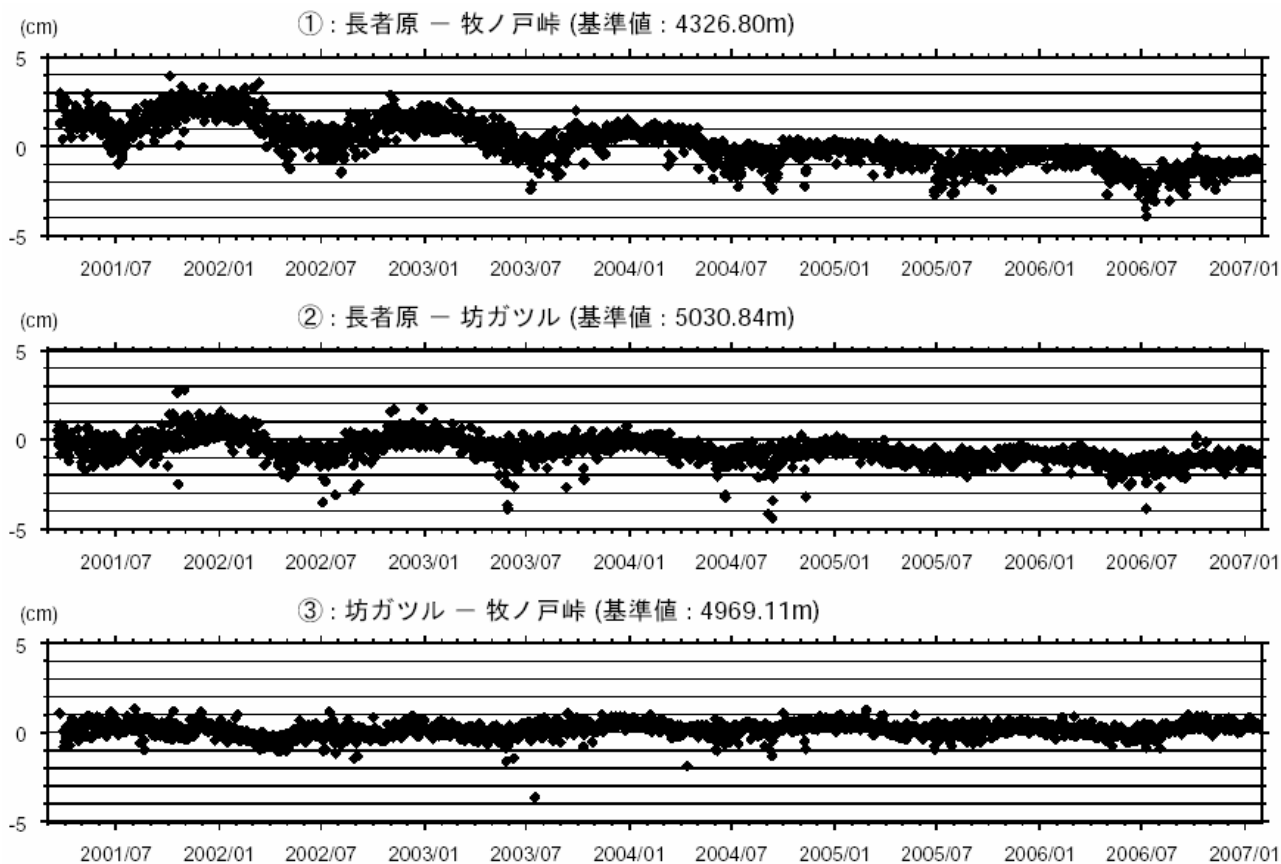
図4 GPS連続観測による基線長変化図(2001年3月1日～2007年1月31日)
