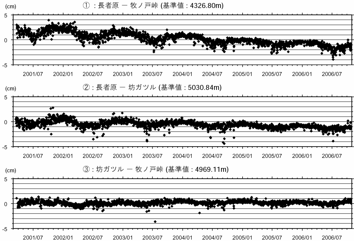
図3 GPSによる基線長変化(2001年3月1日~2006年10月31日)
