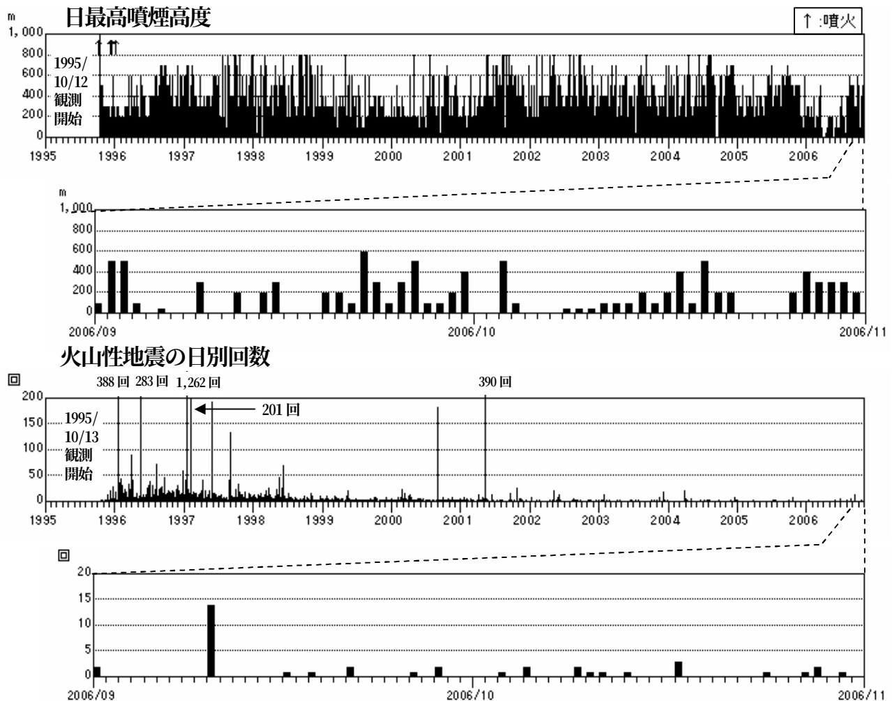
図1 火山活動経過図(1995 年 10 月 12 日～2006 年 10 月 31 日)
