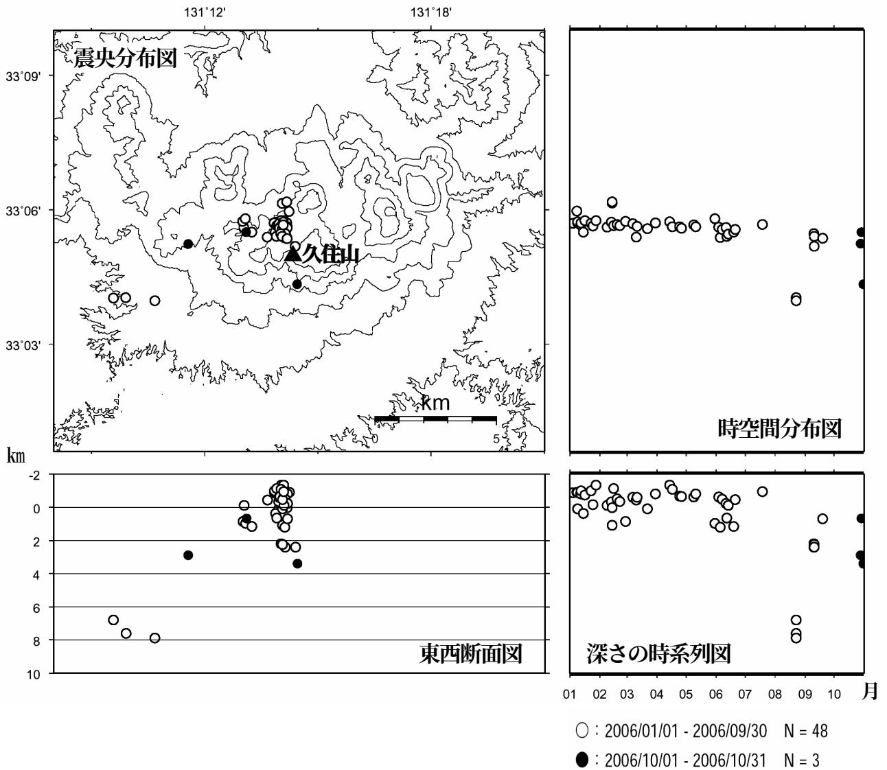
図2 火山性地震の震源分布(2006 年 1 月 1 日～10 月 31 日)
