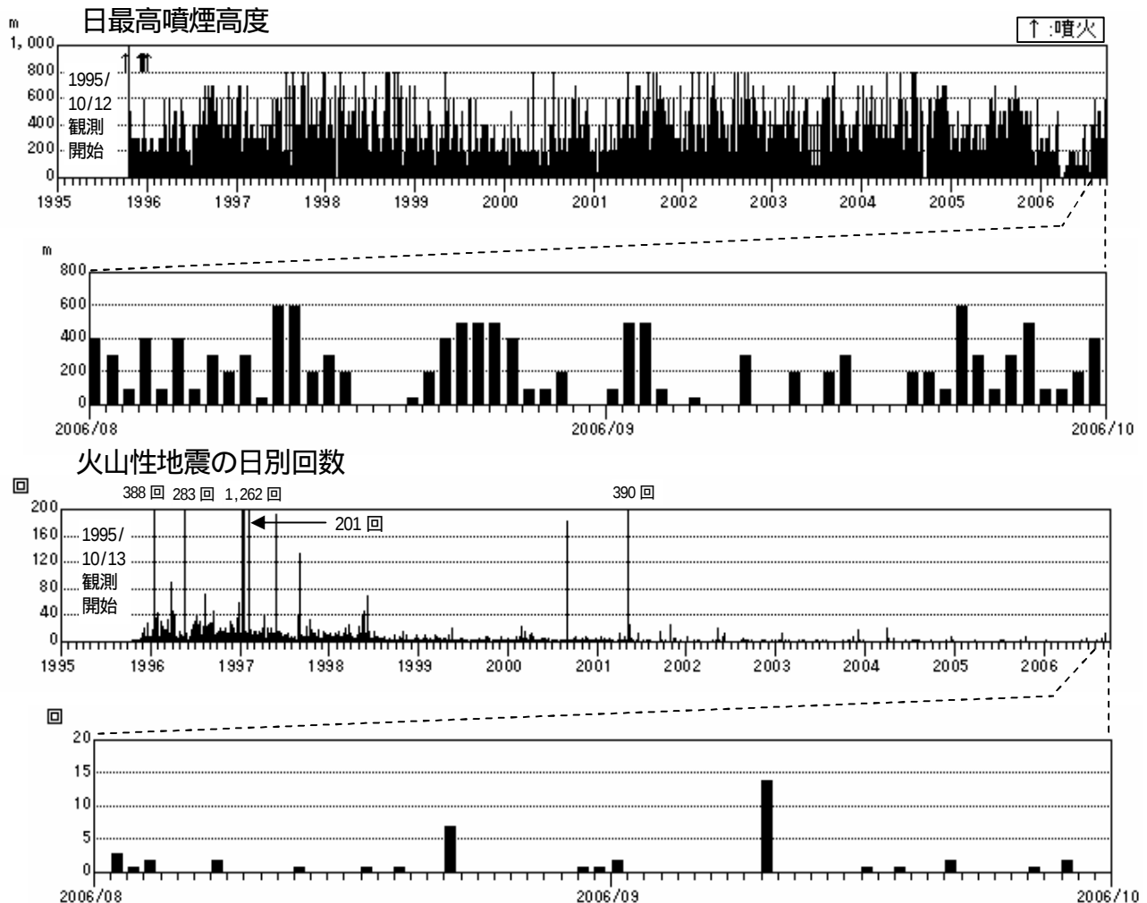
図1 火山活動経過図(1995 年 10 月 12 日～2006 年 9 月 30 日)
