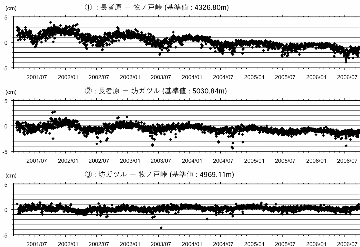
図3 GPSによる基線長変化(2001年3月1日~2006年9月30日)
