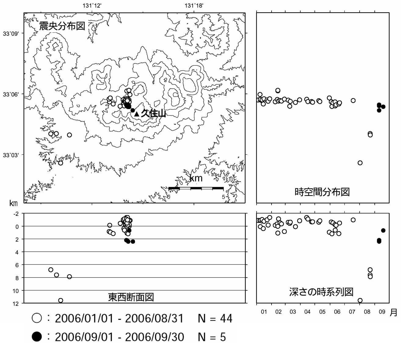
図2 火山性地震の震源分布(2006 年 1 月 1 日～ 9 月 30 日)
