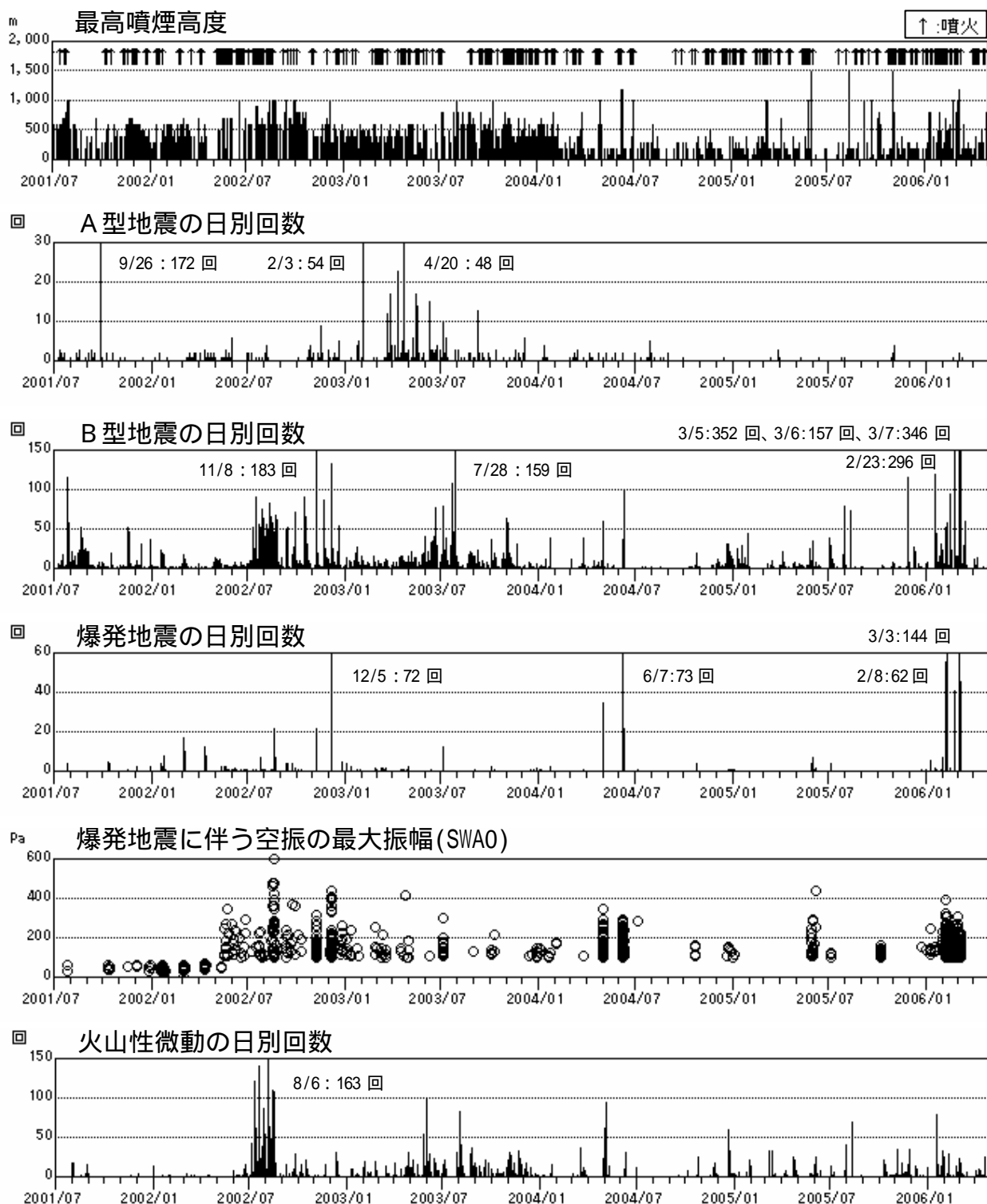
図2 火山活動経過図(2001年7月～2006年4月)
