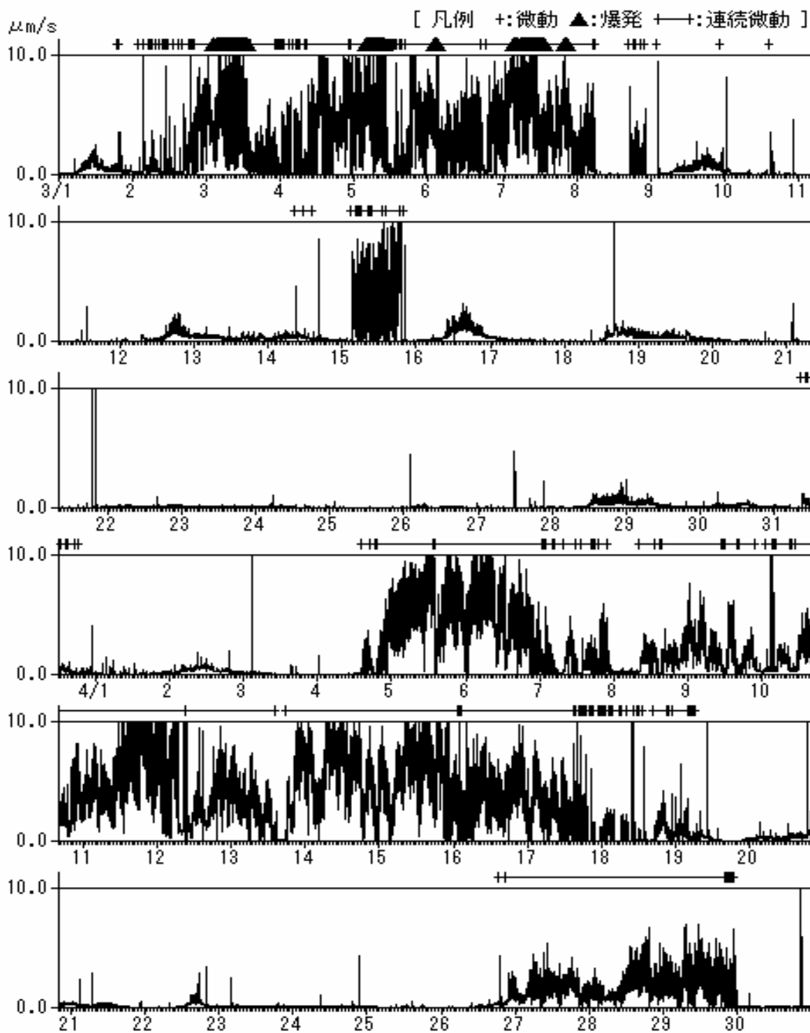
図3 1分間平均振幅の時間変化図(2006年3月1日～4月30日) 火山性連続微動は、4月4～19日と26～29日に発生しました。
