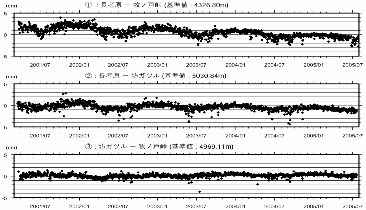
図3 GPSによる基線長変化図(2001年3月1日~2005年7月31日)
