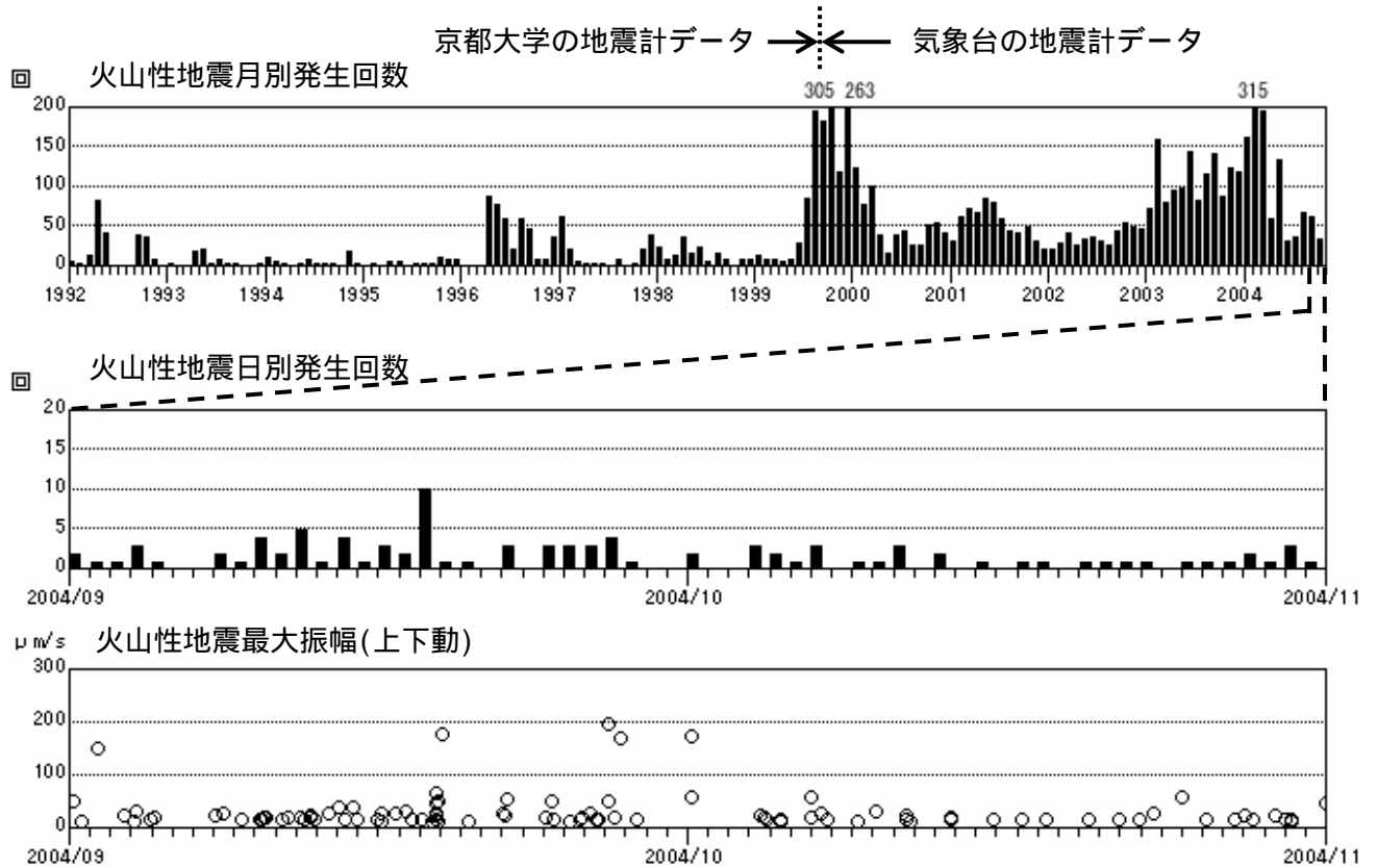
図 1 火山性地震活動経過図(1992年1月1日~2004年10月31日) 1999年9月12日までは、京都大学のデータを利用。
