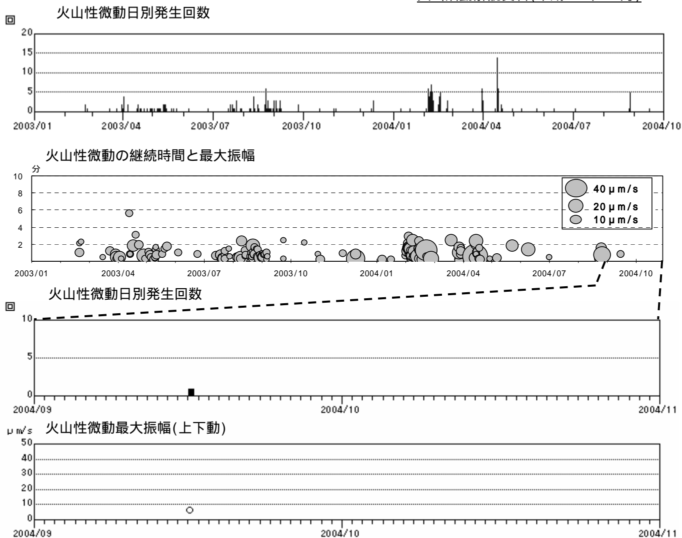
図2 火山性微動活動経過図(2003年1月1日~2004年10月31日)
