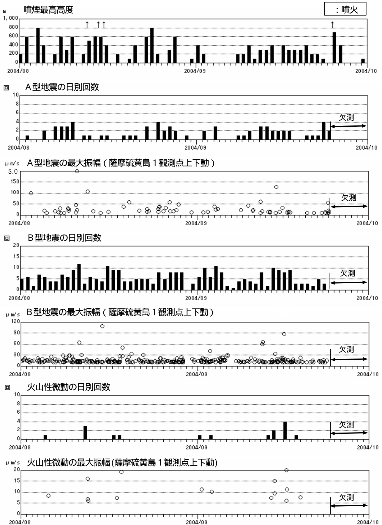
図3 薩摩硫黄島火山活動経過図(2004年8月1日～9月30日)
