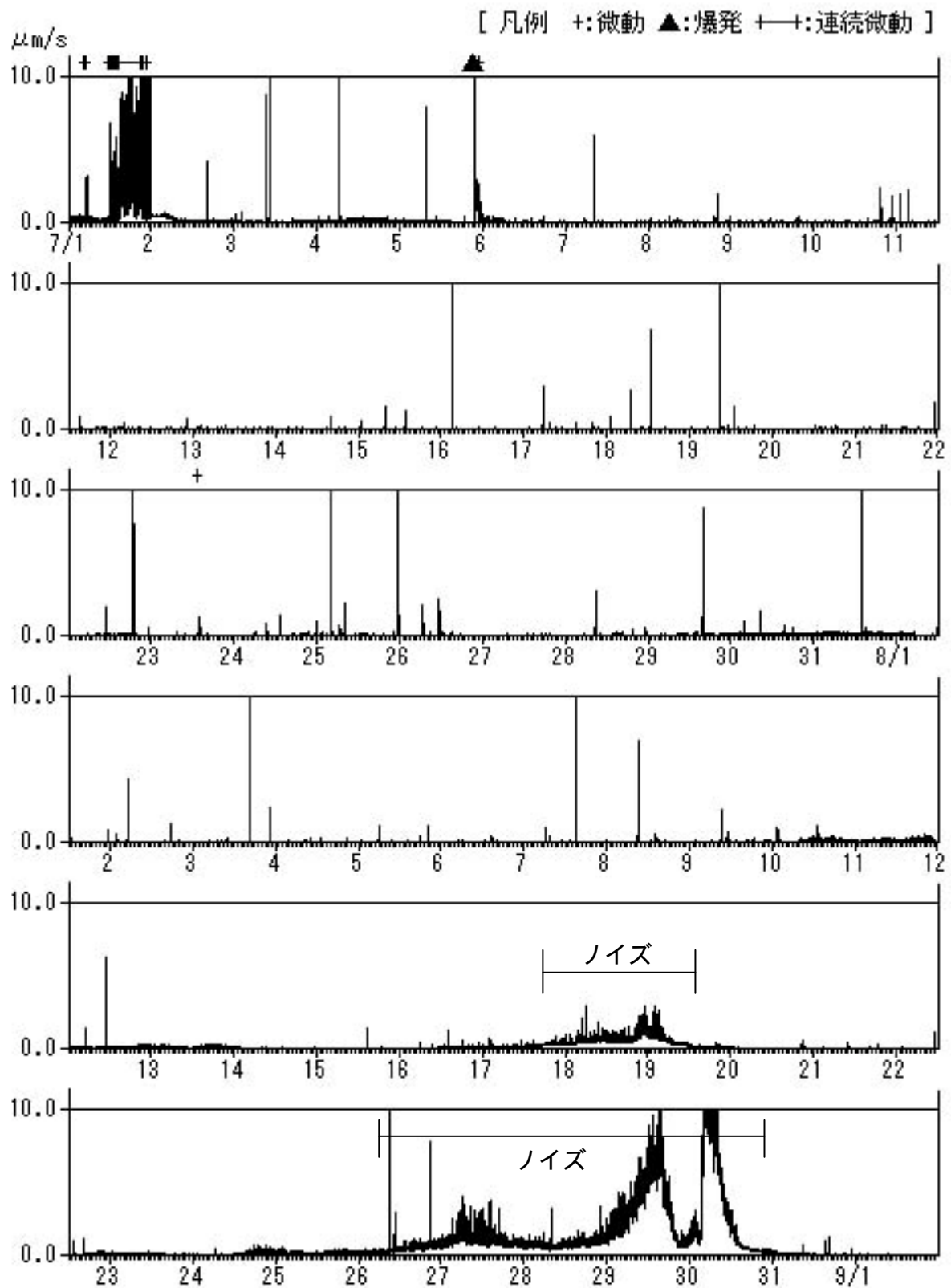
図4 地震計(上下動)の1分間平均振幅の変化(2004年7月1日～8月31日)
