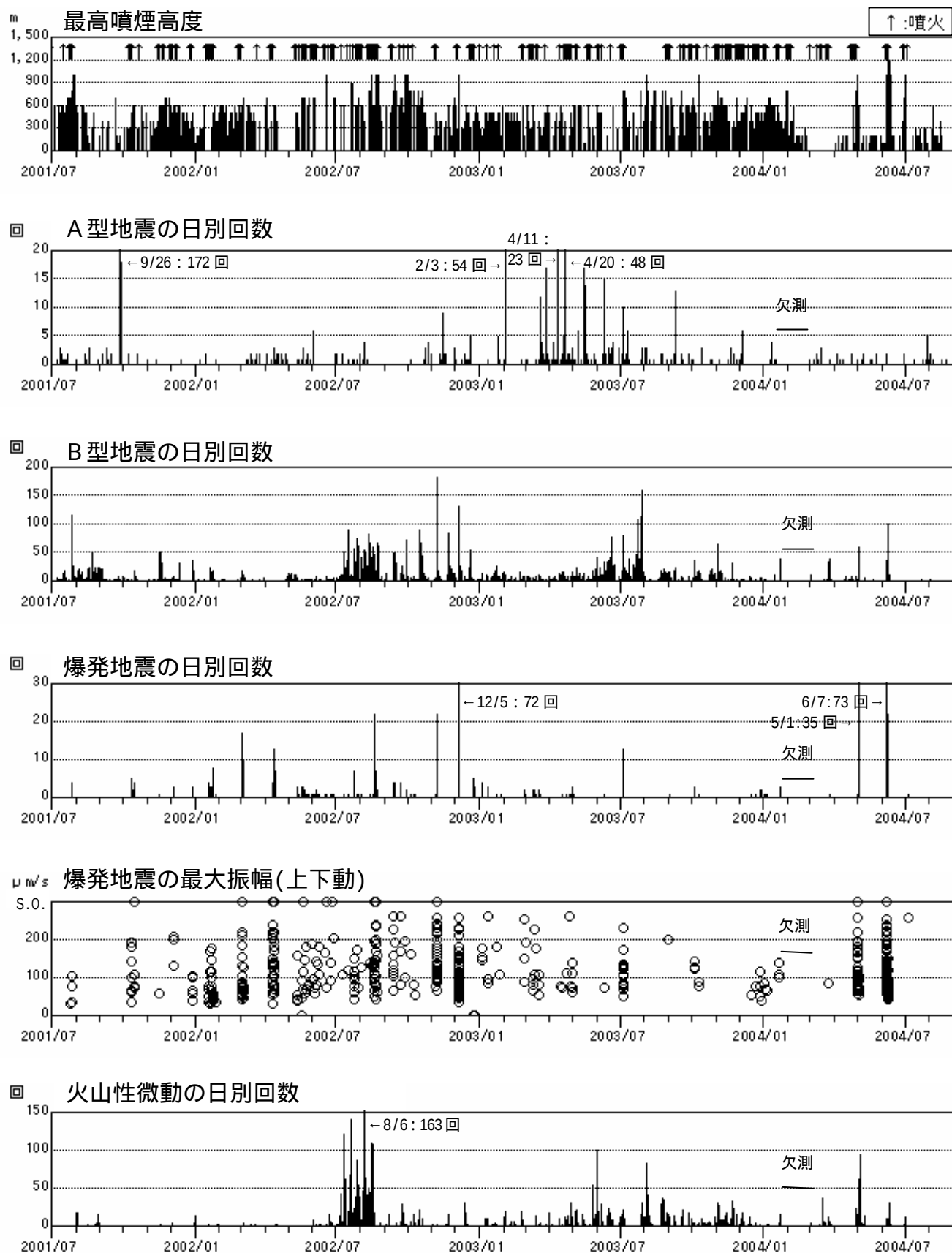
図2 火山活動経過図(2001年7月～2004年8月)
