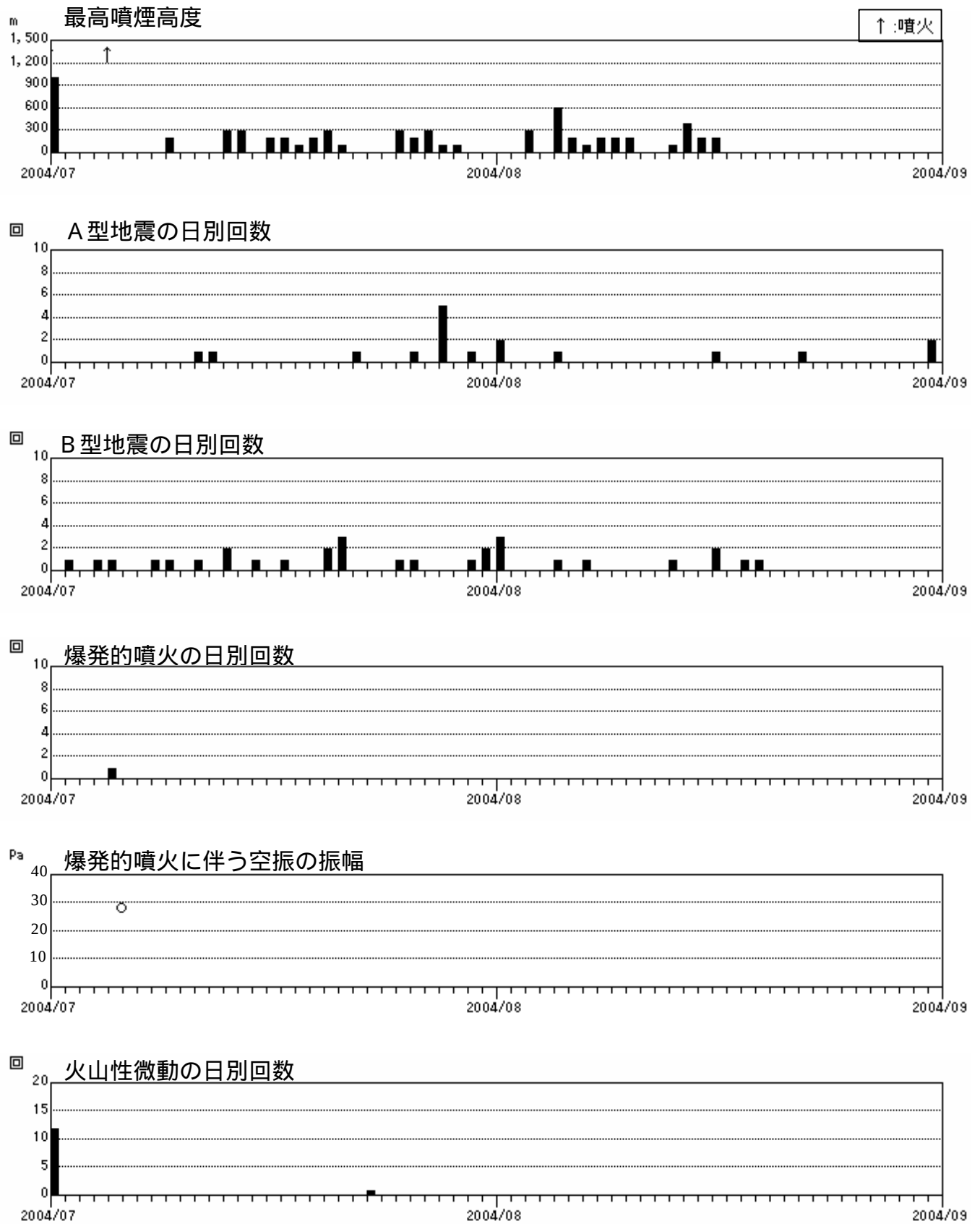
図 3 火山活動経過図(2004 年 7 月 1 日～ 8 月 31 日)
