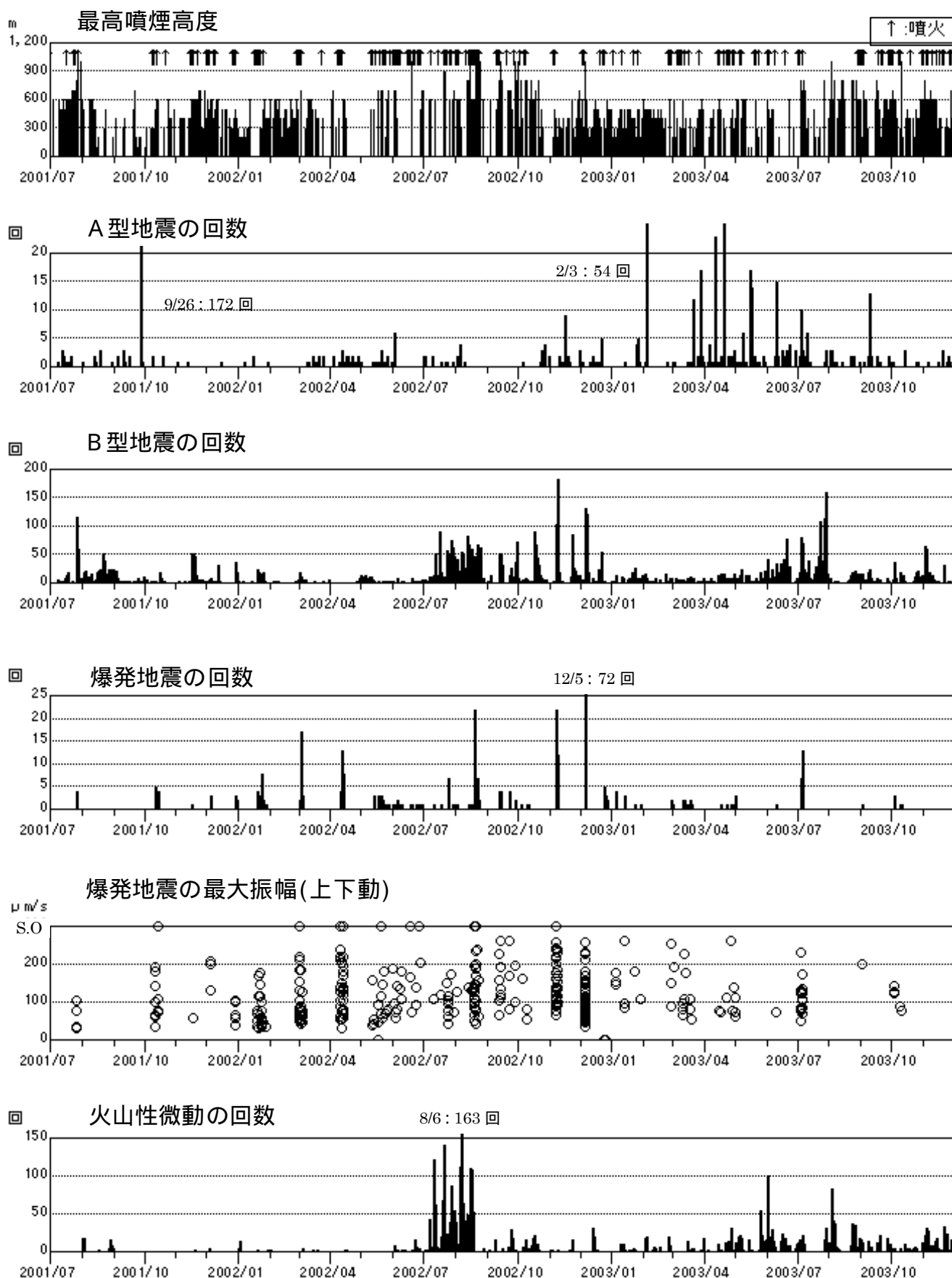
図2 火山活動経過図(2001年7月～2003年11月)
