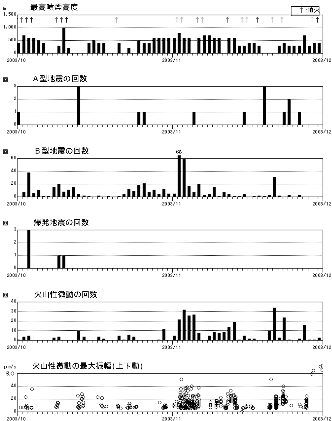
図3 火山活動経過図(2003年10月1日～2003年11月30日)
