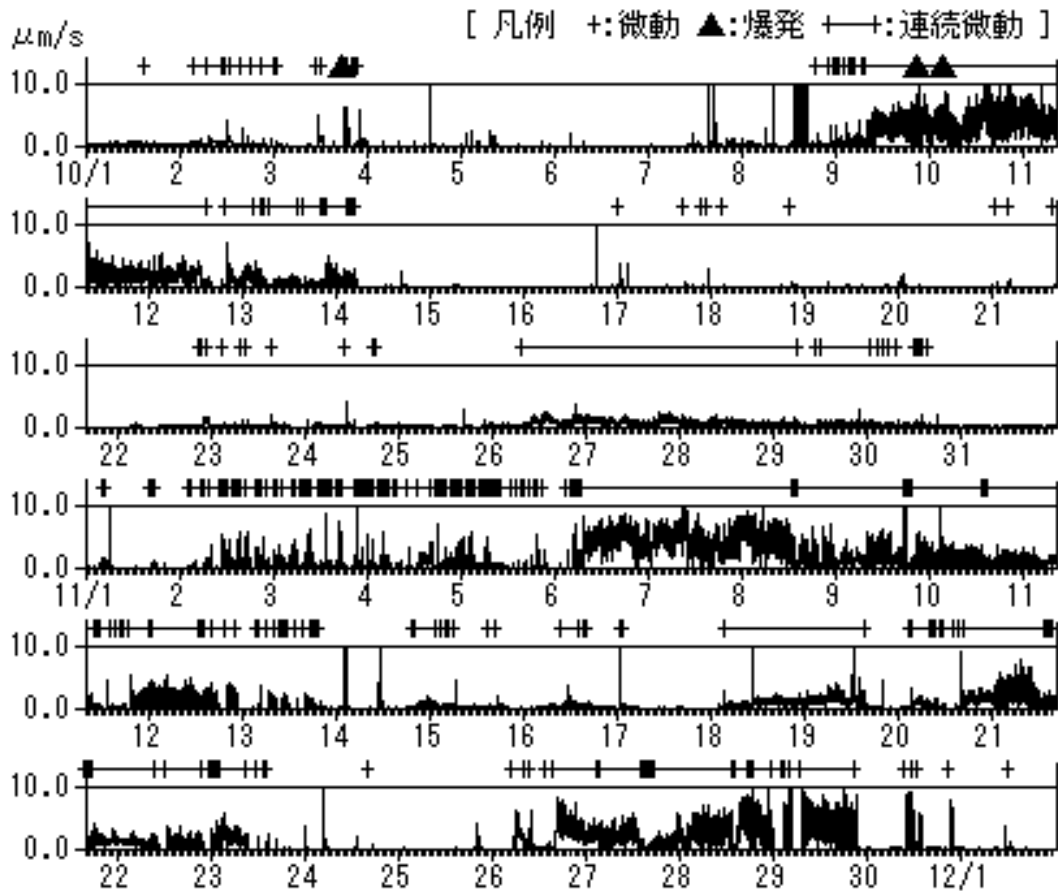
図4 地震計(上下動)の1分間平均振幅の変化(2003年10月1日~11月30日)
