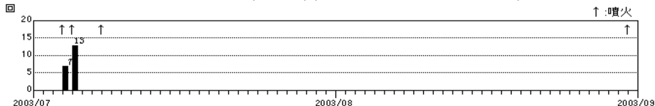
図 10 爆発地震の日別回数(2003 年 7 月 1 日～ 8 月 31 日)
