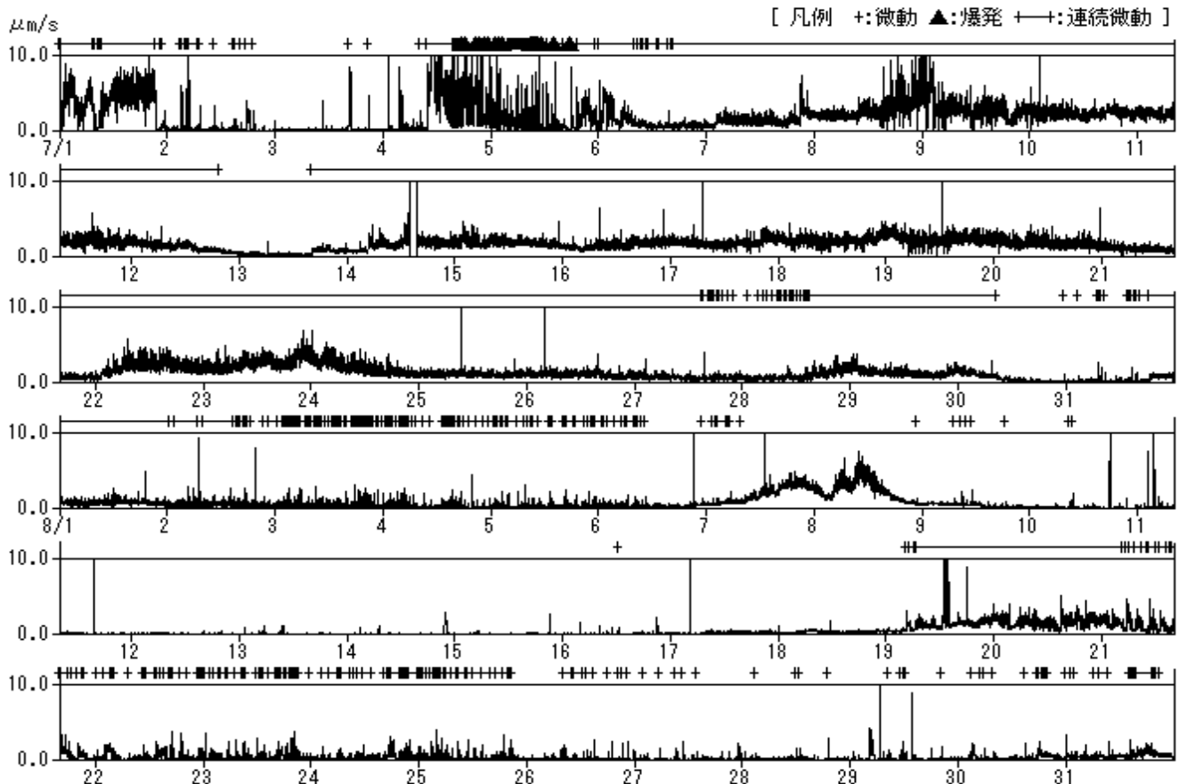
図 4 1 分間平均振幅の時間変化(上下動)(2003 年 7 月 1 日 ~ 8 月 31 日)
