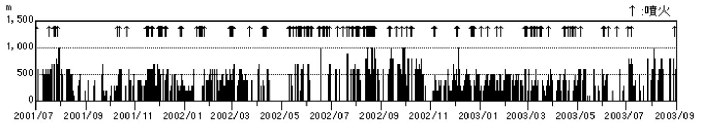
図 1 日別噴煙最高高度(2001 年 7 月 ~ 2003 年 8 月)
