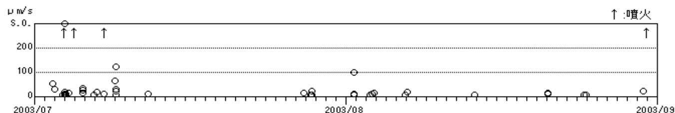
図7 A型地震の最大振幅(上下動)(2003年7月1日～8月31日)
