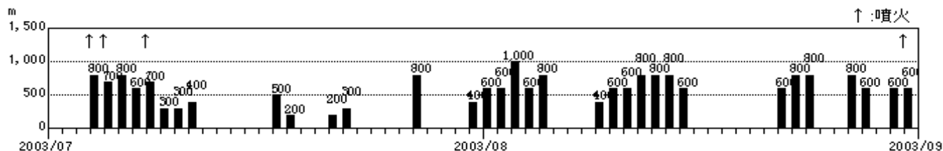
図5 日別噴煙最高高度(2003年7月1日～8月31日)
