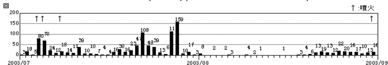
図 8 B 型地震の日別回数(2003 年 7 月 1 日～ 8 月 31 日)
