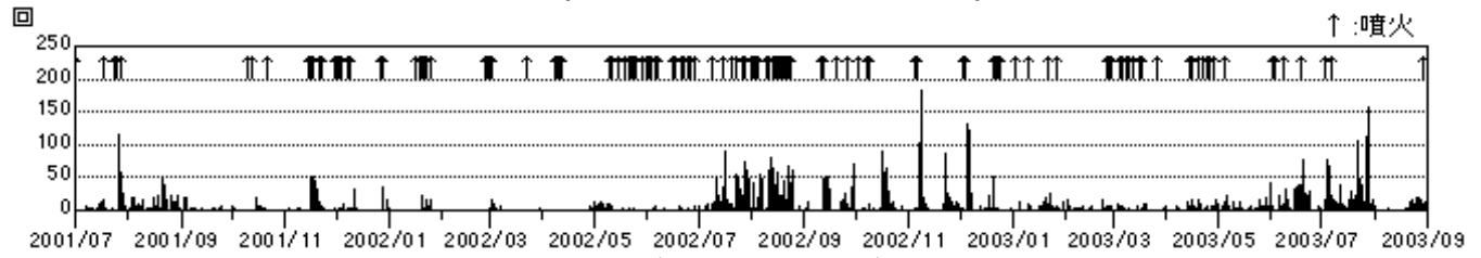
図 3 B 型地震の日別回数(2001 年 7 月 ~ 2003 年 8 月)
