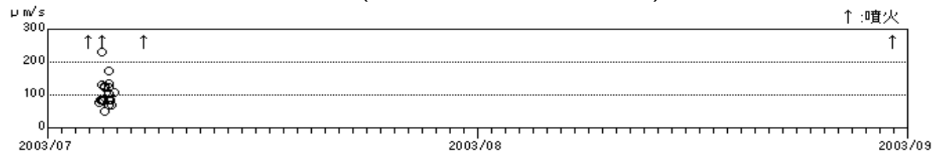
図 11 爆発地震の最大振幅(上下動)(2003 年 7 月 1 日～8 月 31 日)
