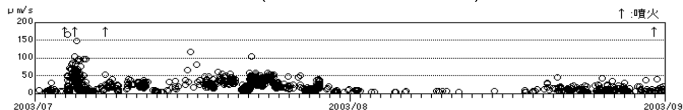
図9 B型地震の最大振幅(上下動)(2003年7月1日～8月31日)
