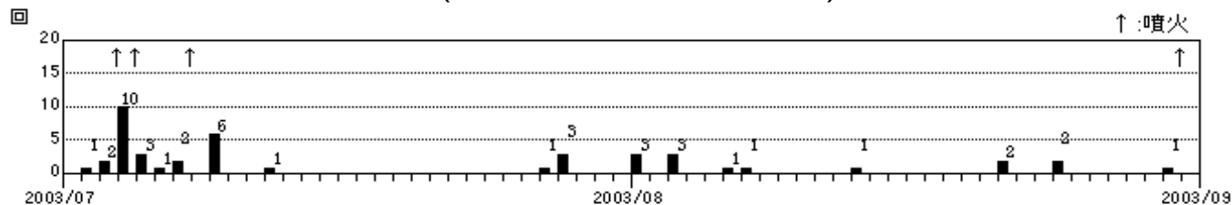
図6 A型地震の日別回数(2003年7月1日～8月31日)
