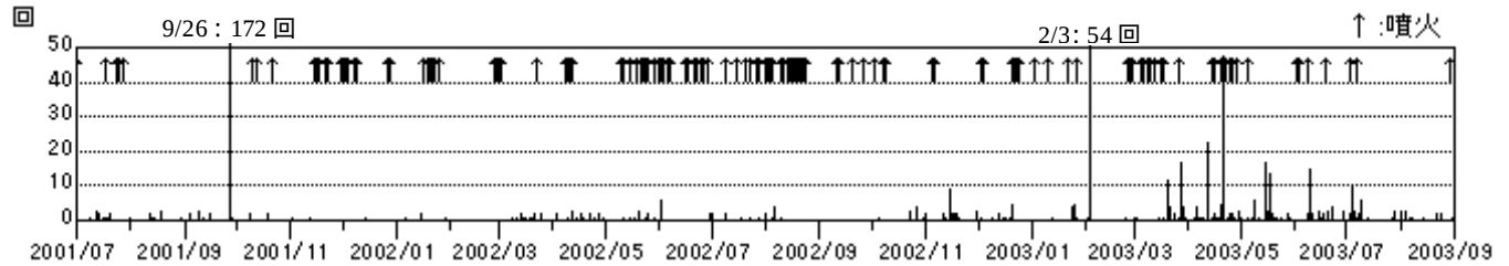
図 2 A 型地震の日別回数(2001 年 7 月 ~ 2003 年 8 月)
