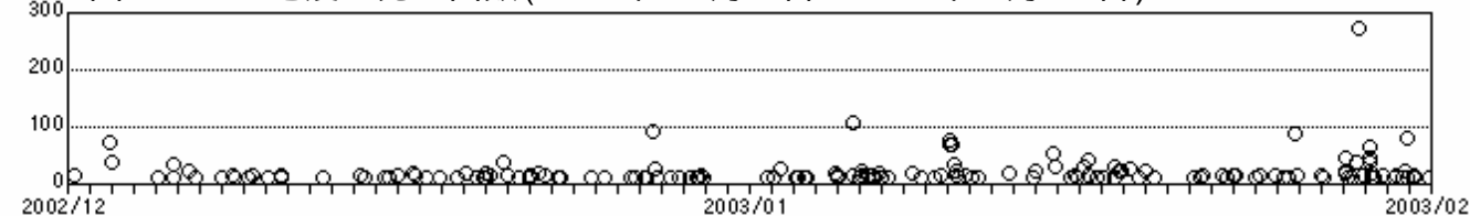
図7 B型地震の最大振幅分布(上下動)(2002年12月1日~2003年1月31日)
