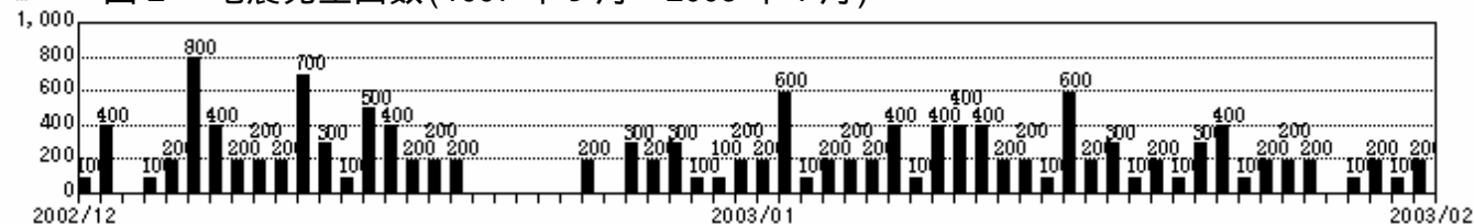
図 3 噴煙の日最高高度(2002 年 12 月 1 日～2003 年 1 月 31 日)
