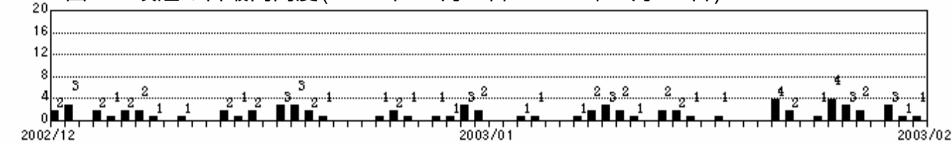
図 4 A 型地震の発生回数(2002 年 12 月 1 日～2003 年 1 月 31 日)
