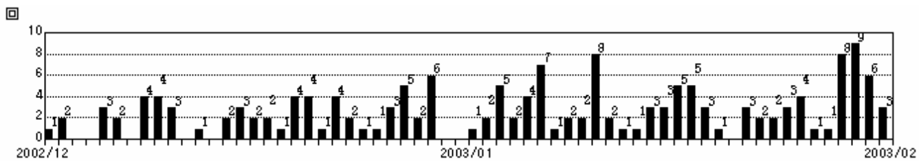
図6 B型地震の発生回数(2002年12月1日~2003年1月31日)
