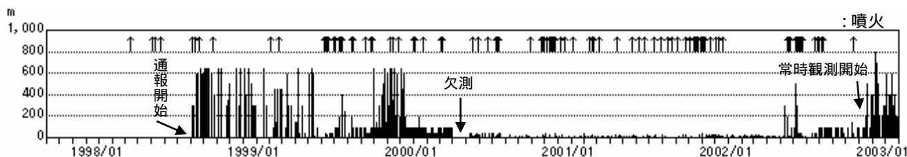
図 1 噴煙の日最高高度(1998 年 8 月～2003 年 1 月)
