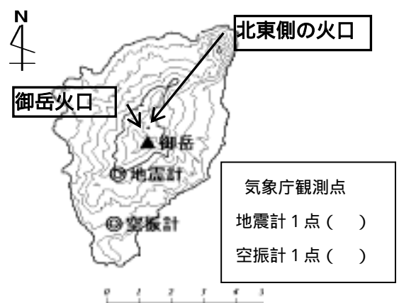
図12 観測点配置図
