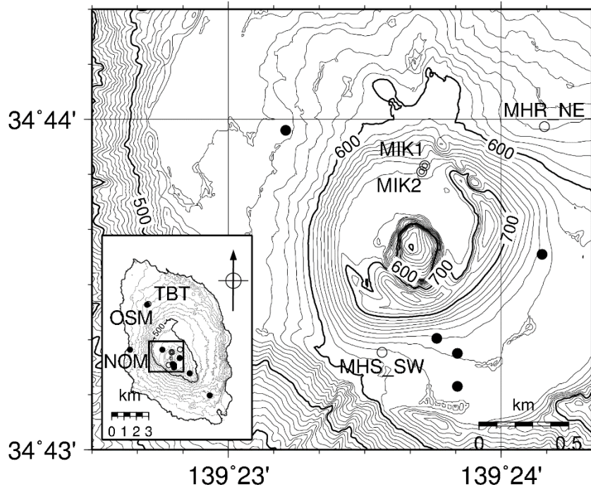
第1図 三原山火口付近と伊豆大島全域の全磁力連続観測点配置 (◎：地磁気観測所、○：気象庁地震火山部、●：東京大学地震研究所)。MIK1・MIK2は2007年3月、TBT・MHR_NS・MHS_SWは2013年3月に観測を開始した。この地図の作成には、国土地理院発行の「数値地図10mメッシュ(火山標高)」を使用した。(承認番号 平29情使、第798号)
