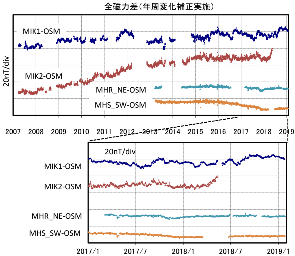
第3図 年周変化補正後の全磁力日平均値差 (上図：2007年3月～2019年1月、下図：2017年1月～2019年1月)
