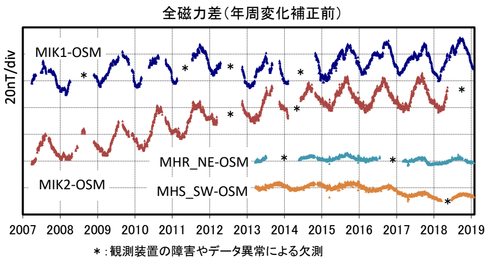
第2図 各連続観測点と参照点OSMの全磁力日平均値差(2007年3月～2019年1月) Fig. 2. Daily mean values of the geomagnetic total intensities at the stations MIK1, MIK2, MHR_NE and MHS_SW with reference to the station OSM from March 2007 to January 2019.
