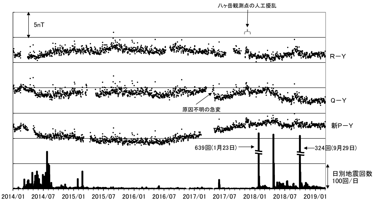
第3図 全磁力連続観測による全磁力値の変化及び日別地震回数（2014年1月～2019年2月28日）。連続観測点新P、QおよびRにおける八ヶ岳地球電磁気観測所（東京大学地震研究所）（Y）との全磁力の日平均値差。最下段に草津白根山で観測された日別地震回数を示す。
