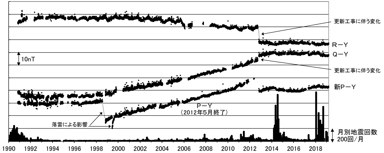
第2図 全磁力連続観測による全磁力値の変化及び月別地震回数（1990年1月～2019年2月28日）。連続観測点P、Q、Rおよび新Pにおける八ヶ岳地球電磁気観測所（東京大学地震研究所）（Y）との全磁力の日平均値差。最下段に草津白根山で観測された月別地震回数を示す。
