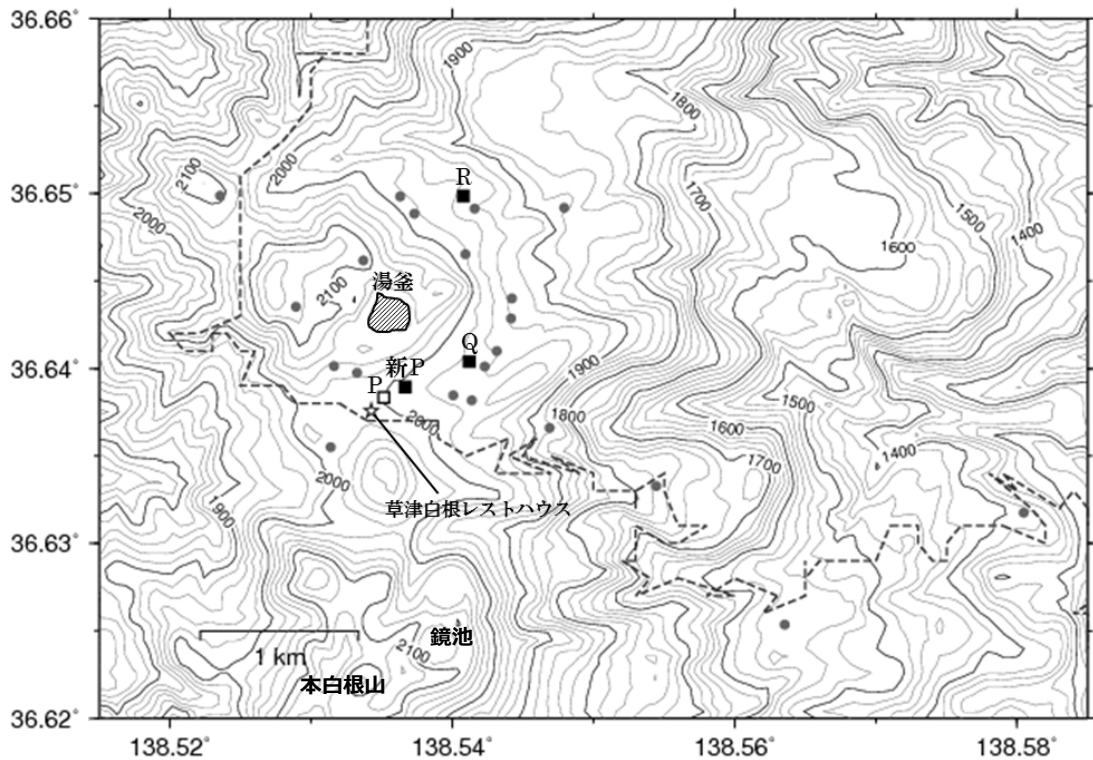
第 1 図 全磁力連続観測点 (P, Q, R, 新 P) の配置図
