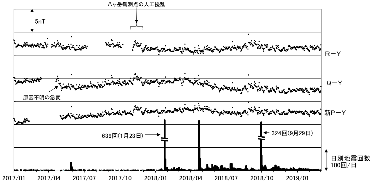
第4図 全磁力連続観測による全磁力値の変化及び日別地震回数（2017年1月～2019年2月28日）。連続観測点新P、QおよびRにおける八ヶ岳地球電磁気観測所（東京大学地震研究所）（Y）との全磁力の日平均値差。最下段に草津白根山で観測された日別地震回数を示す。
