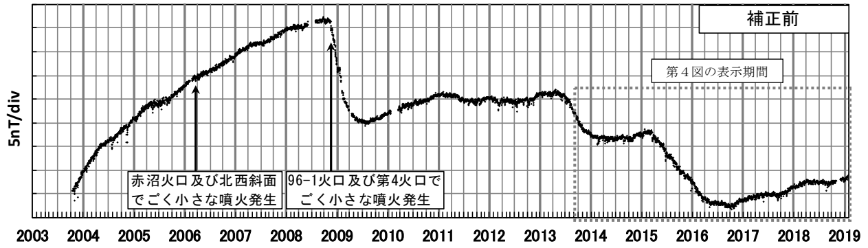
第5図 ポンマチ南東と女満別観測施設の全磁力日平均値差 (2003年10月16日～2019年1月31日) 年周変化量と太陽活動等によるノイズ量を補正していない。
