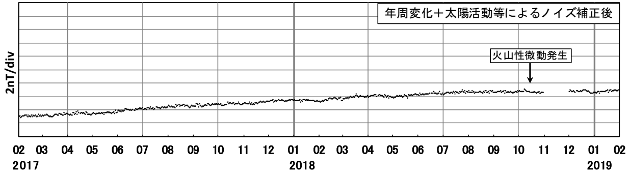
第3図 ポンマチ南東と女満別観測施設の全磁力日平均値差 (2017年2月1日～2019年1月31日) 年周変化量と太陽活動等によるノイズ量を補正している。
