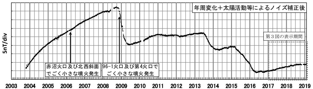
第2図 ポンマチ南東と女満別観測施設の全磁力日平均値差 (2003年10月16日～2019年1月31日) 年周変化量と太陽活動等によるノイズ量を補正している。
