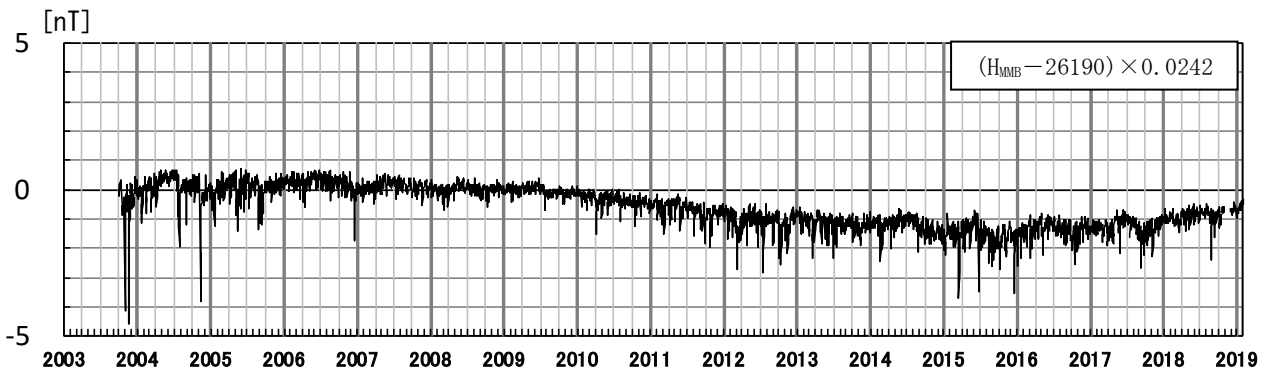
第7図 女満別観測施設の地磁気水平成分 ( H_{\text{MMB}} ) から求めた太陽活動等によるノイズ量 (2003年10月16日～2019年1月31日)
