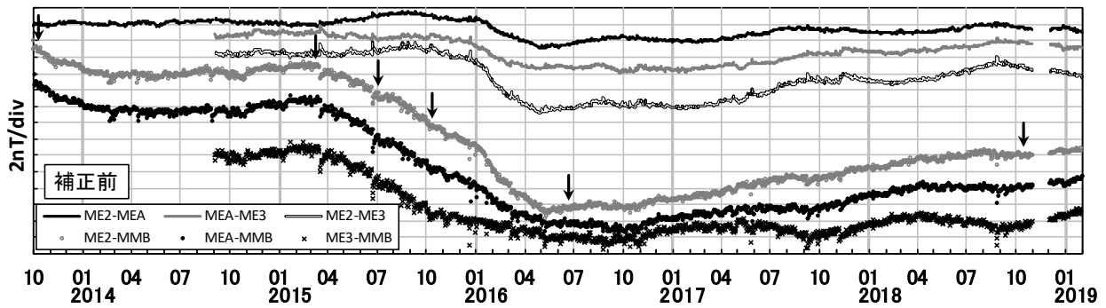
第4図 各連続観測点 (MEA、ME2、ME3) と女満別観測施設 (MMB) の全磁力日平均値差及び各連続観測点間の全磁力日平均値差 (2013年10月1日～2019年1月31日) 年周変化量と太陽活動等によるノイズ量を補正していない。矢印は火山性微動の発生日を示す。
