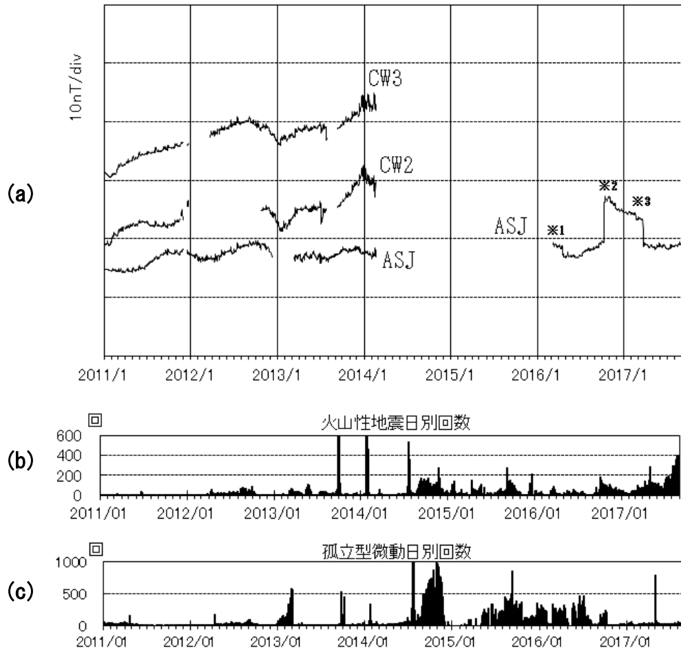
第2図 2011年1月から2017年8月まで連続観測点CW2、CW3、ASJにおける全磁力日平均値と参照点AHKの日平均値との差(a)、火山性地震日別回数(b)、孤立型微動日別回数(c)
