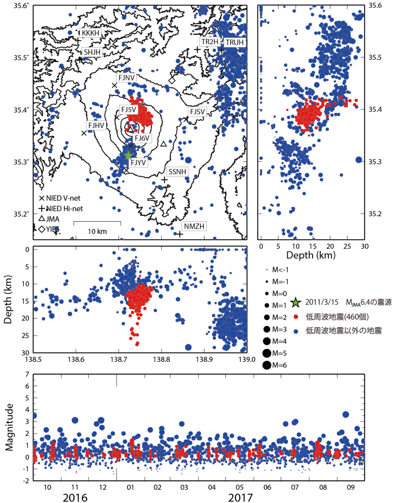
図1 富士山の震源分布および時空間分布図
