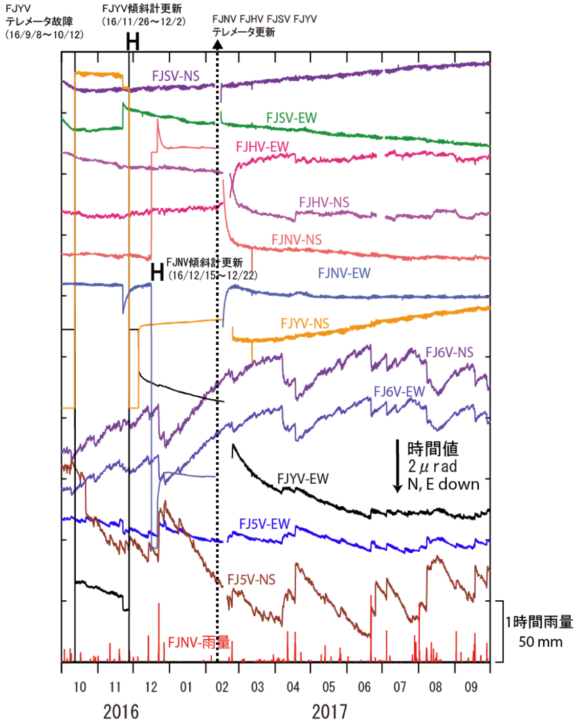
第4図 富士山火山活動観測網による傾斜変動観測結果
