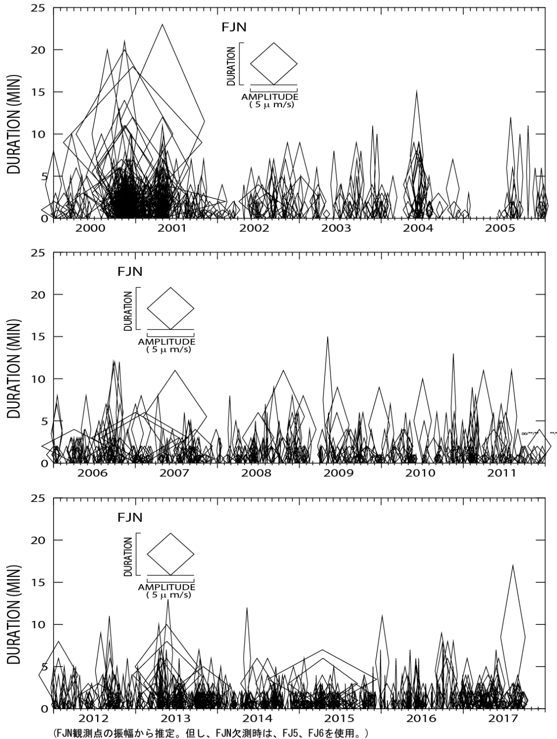
図2 富士山の低周波地震活動の時間変化を示す菱形ダイアグラム(1997年から2017年9月30日) 菱形の高さは特定の観測点で記録された低周波地震活動の振動継続時間、その幅はその最大振幅を示す。
