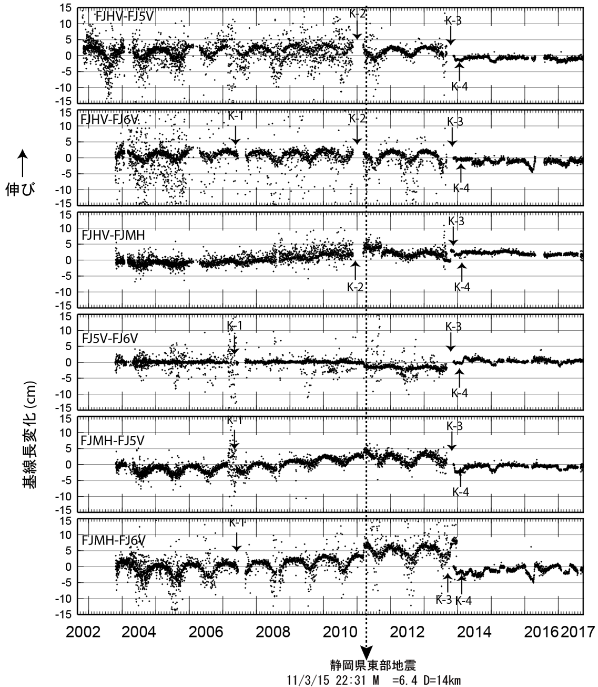
第5図 防災科学技術研究所・富士山火山活動観測網によるGNSS観測結果。表示期間は2002年10月24日～2017年9月30日で、表示データは基線長変化の日平均値。
