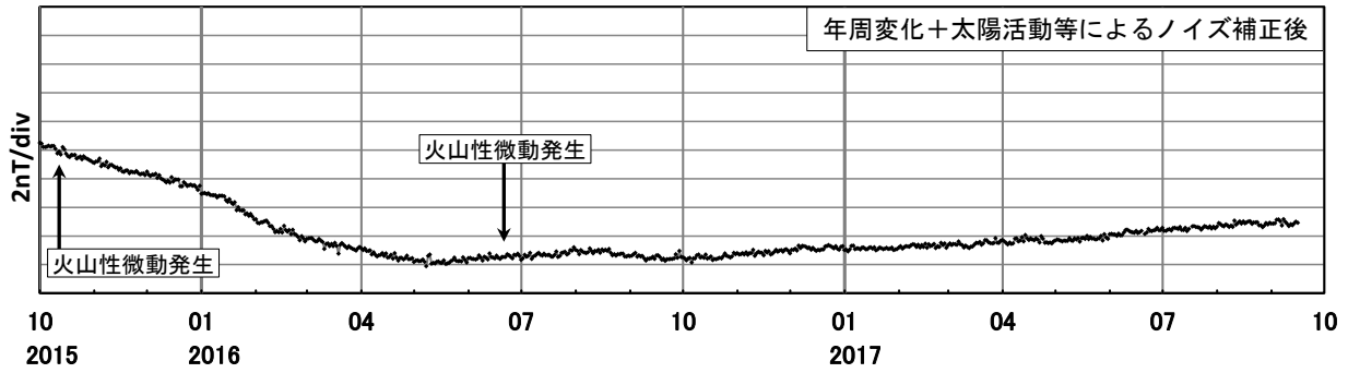
第3図 ポンマチ南東と女満別観測施設の全磁力日平均値差（2015年10月1日～2017年9月16日） 年周変化補正と太陽活動等によるノイズ補正を行っている。
