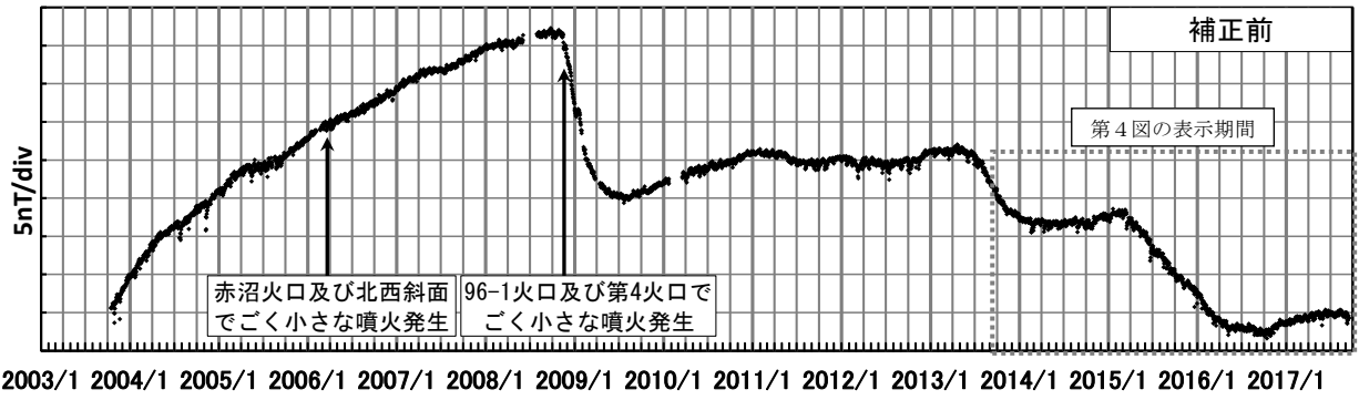
第5図 ポンマチ南東と女満別観測施設の全磁力日平均値差 (2003年10月16日～2017年9月16日) 年周変化補正と太陽活動等によるノイズ補正を行っていない。
