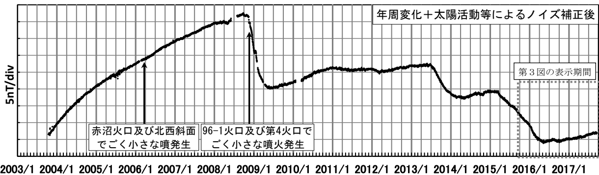
第2図 ポンマチ南東と女満別観測施設の全磁力日平均値差 (2003年10月16日～2017年9月16日) 年周変化補正と太陽活動等によるノイズ補正を行っている。
