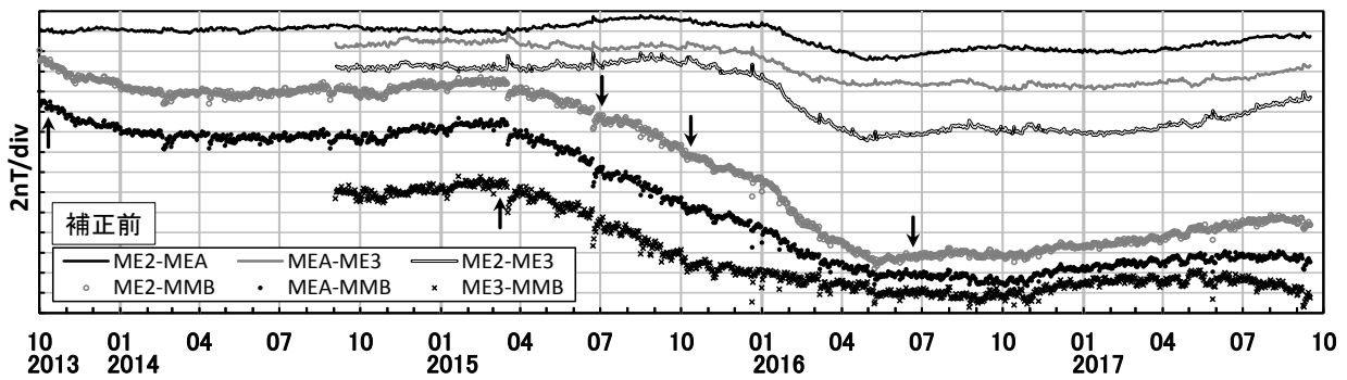
第4図 各連続観測点（MEA、ME2、ME3）と女満別観測施設（MMB）の全磁力日平均値差及び連続観測点間の全磁力日平均値差（2013年10月1日～2017年9月16日） 年周変化補正と太陽活動等によるノイズ補正を行っていない。図中の矢印は火山性微動の発生日を示す。
