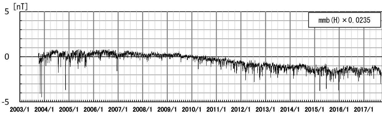
第7図 女満別観測施設の地磁気水平成分から求めた太陽活動等によるノイズ量 (2003年10月16日～2017年9月16日)
