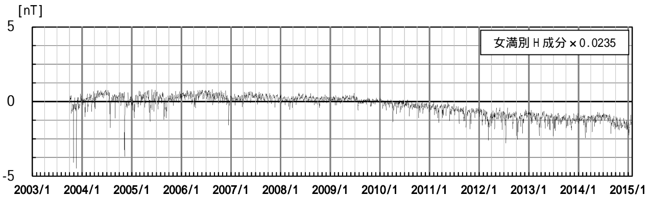
第7図 MMBの地磁気水平成分から求めた太陽活動等によるノイズ量(2003年10月16日~2015年1月31日)
