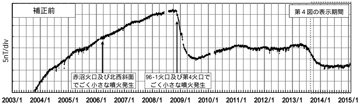
第5図 各種補正前のMEAとMMBの全磁力日平均値差（2003年10月16日～2015年1月31日）
