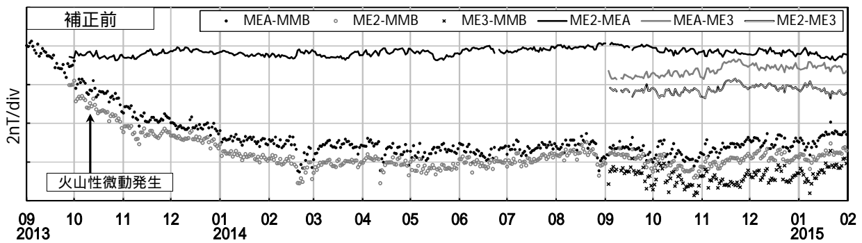
第4図 各種補正前のMEA、ME2、ME3とMMBの全磁力日平均値差及び連続観測点間の全磁力日平均値差（2013年9月1日～2015年1月31日）
