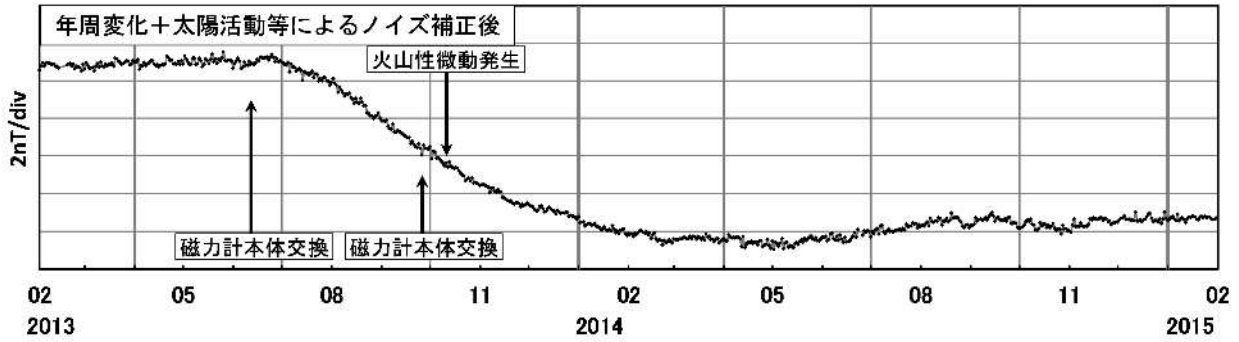
第3図 年周変化補正と太陽活動等によるノイズ補正後のMEAとMMBの全磁力日平均値差（2013年2月1日～2015年1月31日）
