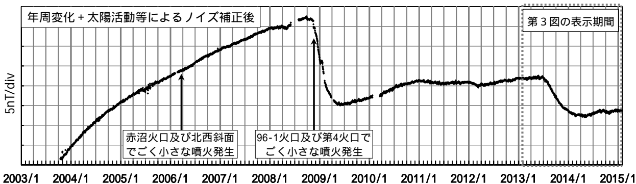
第2図 年周変化補正と太陽活動等によるノイズ補正後の MEA と MMB の全磁力日平均値差 (2003年10月16日~2015年1月31日)
