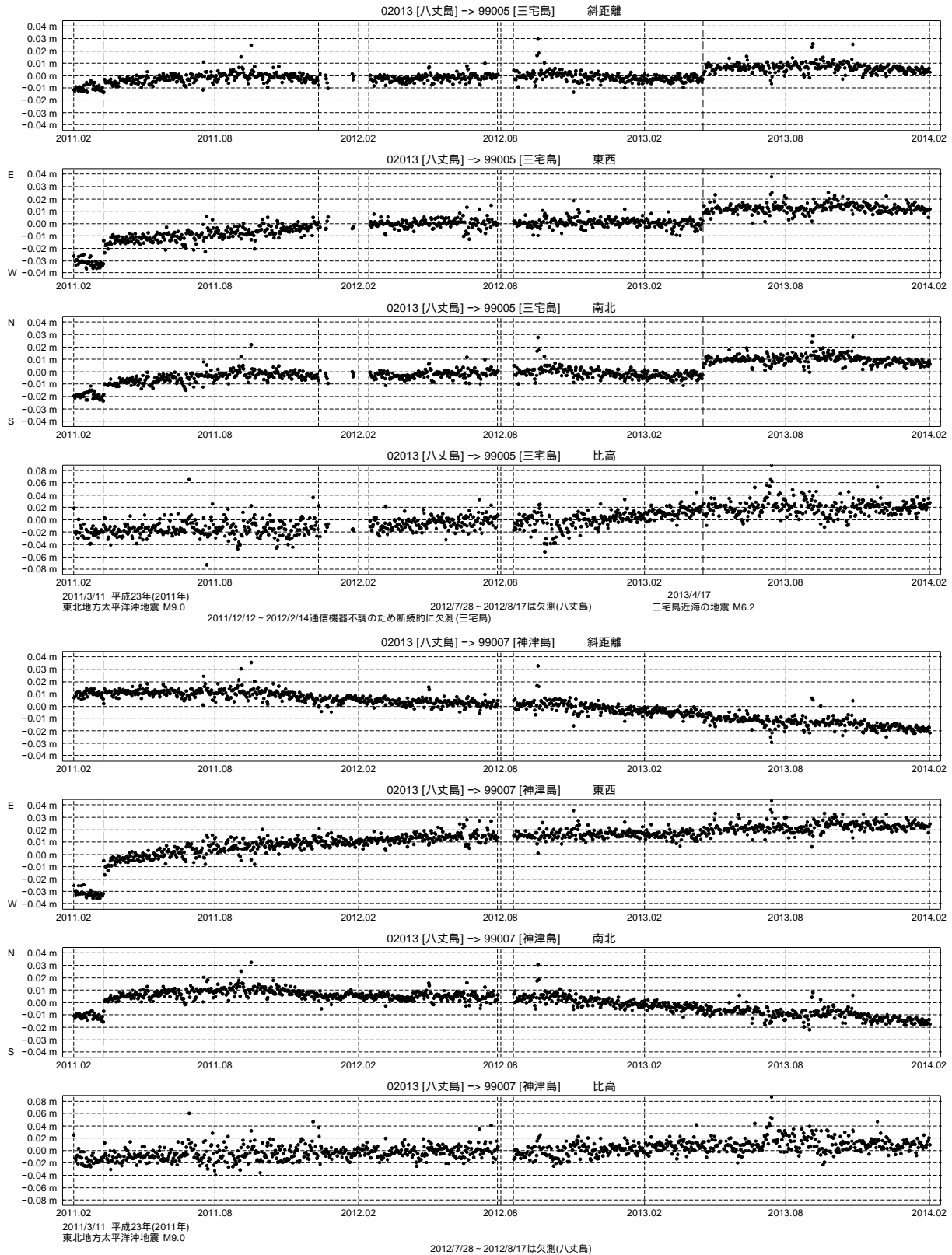
第 6 図 八丈島基点での三宅島および神津島の GPS 連続観測結果 (2011/2/1～2014/1/31)
