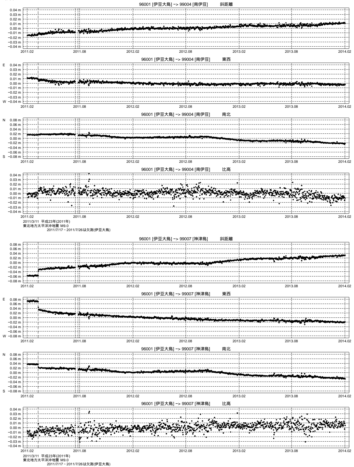
第 3 図 伊豆大島基点での南伊豆および神津島の GPS 連続観測結果 (2011/2/1 ~ 2014/1/31)
