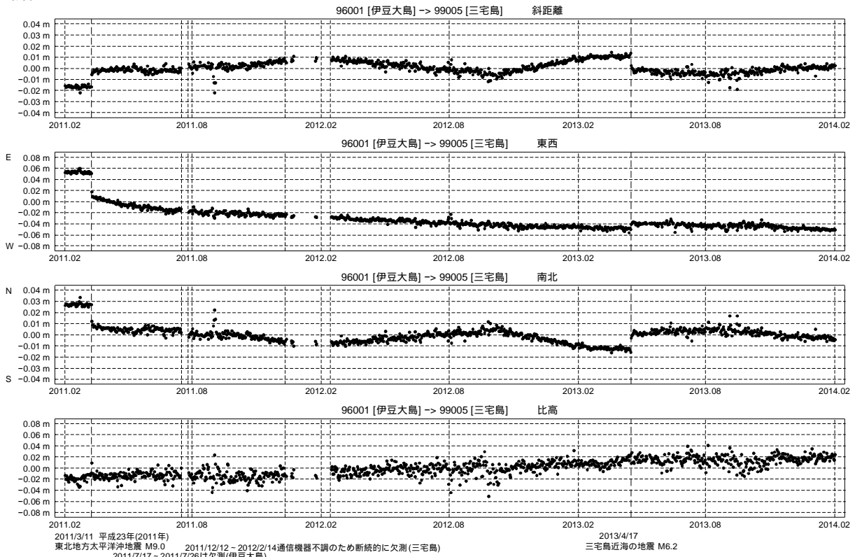
第 4 図 伊豆大島基点での三宅島の GPS 連続観測結果 (2011/2/1 ~ 2014/1/31)
