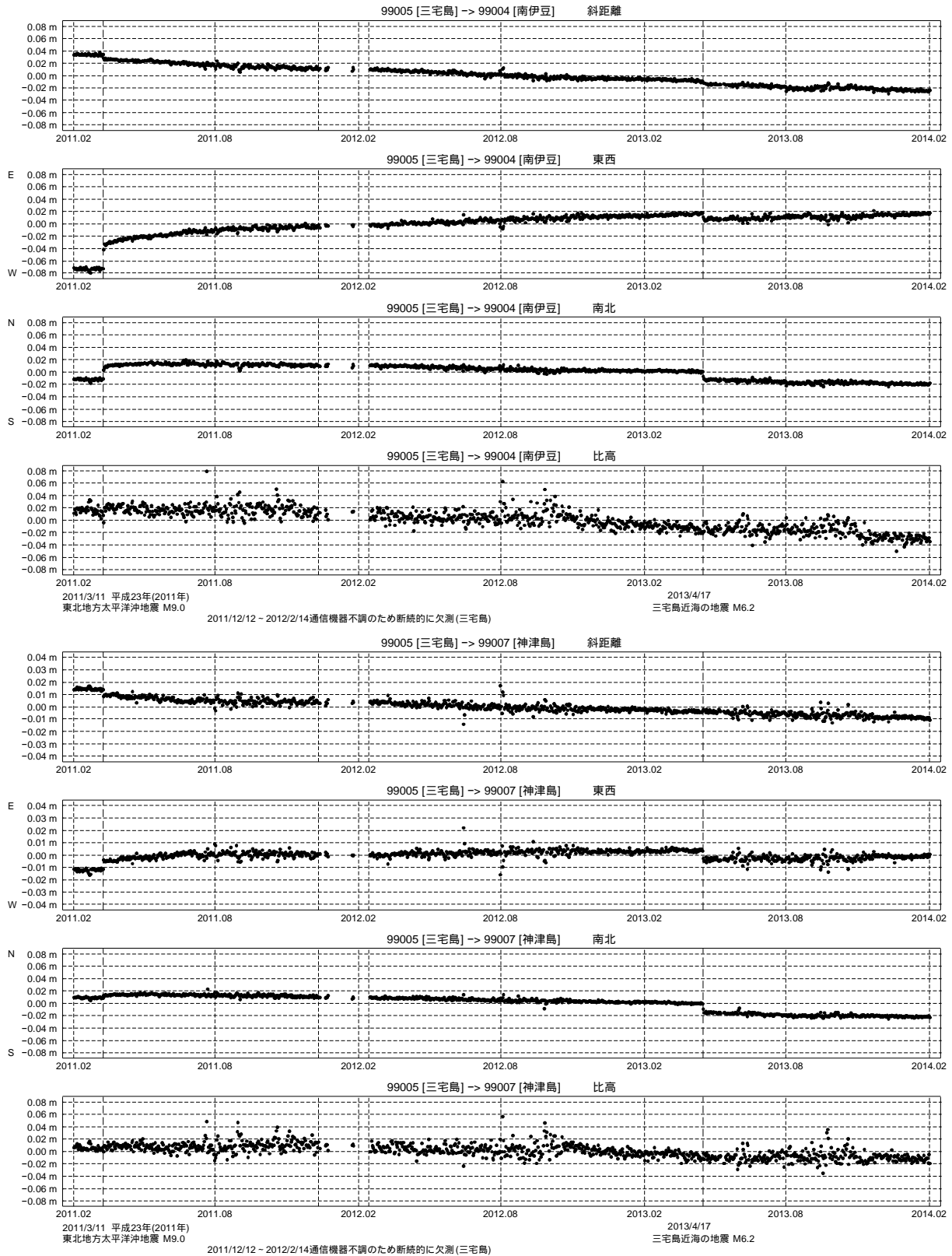
第 5 図 三宅島基点での南伊豆および神津島の GPS 連続観測結果 (2011/2/1～2014/1/31)
