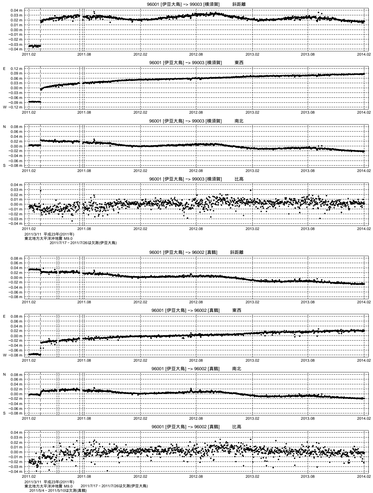
第 2 図 伊豆大島基点での横須賀および真鶴の GPS 連続観測結果 (2011/2/1～2014/1/31)
