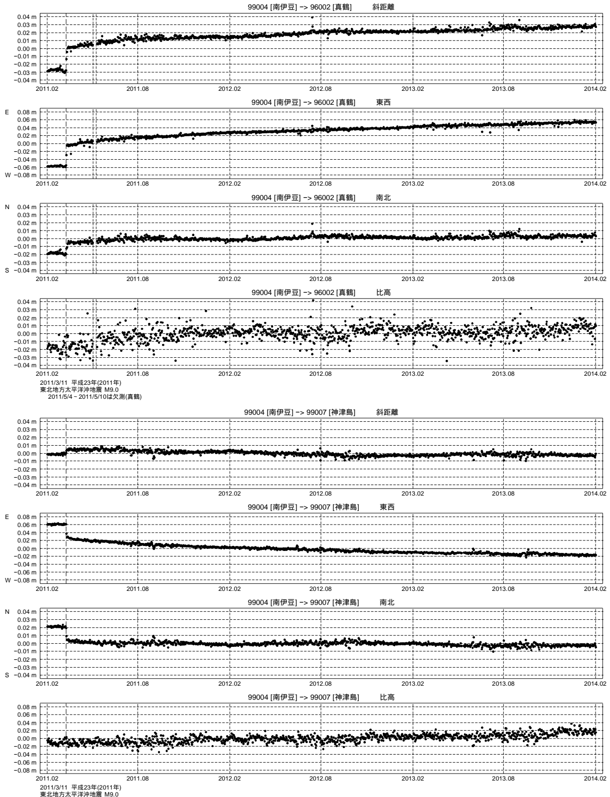
第 7 図 南伊豆基点での真鶴および神津島の GPS 連続観測結果 (2011/2/1～2014/1/31)
