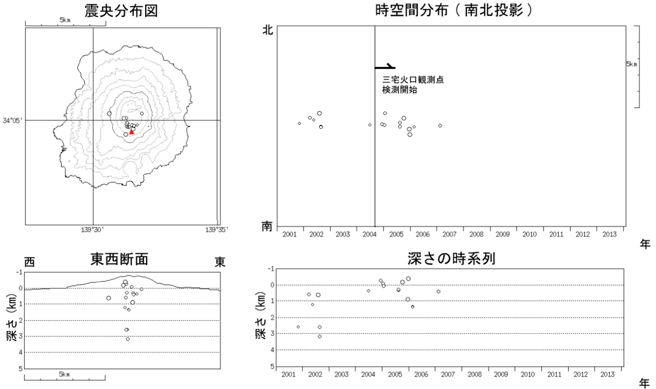
第 8 図 - 三宅島 低周波地震の震源分布 (2001 年 1 月 1 日 ~ 2014 年 1 月 31 日)
