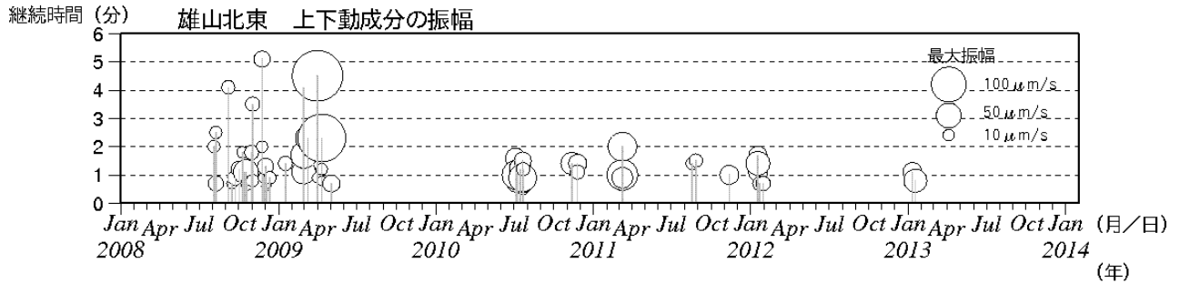
第 9 図 三宅島 単発的な火山性微動の活動経過図 (2008 年 1 月 1 日 ~ 2014 年 1 月 31 日)
