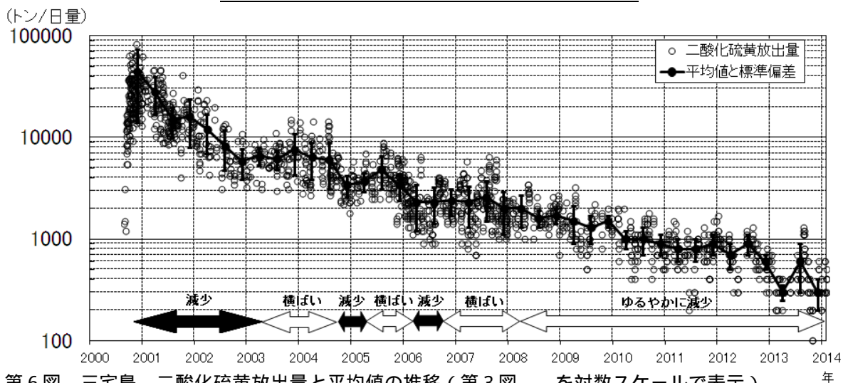
第 6 図 三宅島 二酸化硫黄放出量と平均値の推移 (第 3 図 - を対数スケールで表示)
