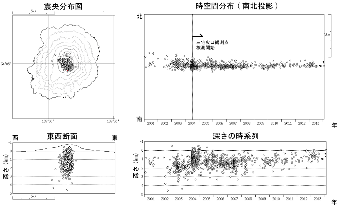
第 8 図 - 三宅島 やや低周波地震の震源分布 (2001 年 1 月 1 日 ~ 2014 年 1 月 31 日)
