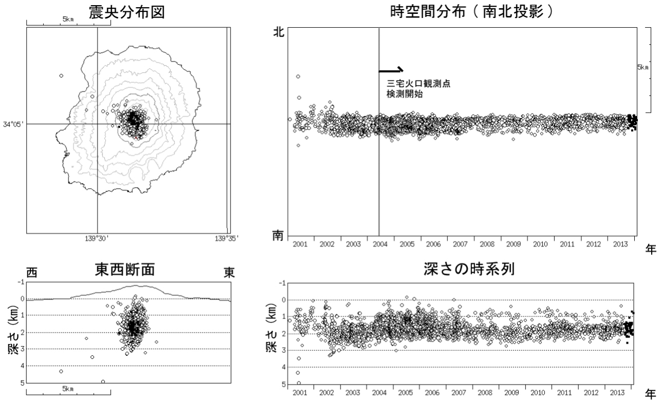
第 8 図 - 三宅島 高周波地震の震源分布 (2001 年 1 月 1 日 ~ 2014 年 1 月 31 日)
