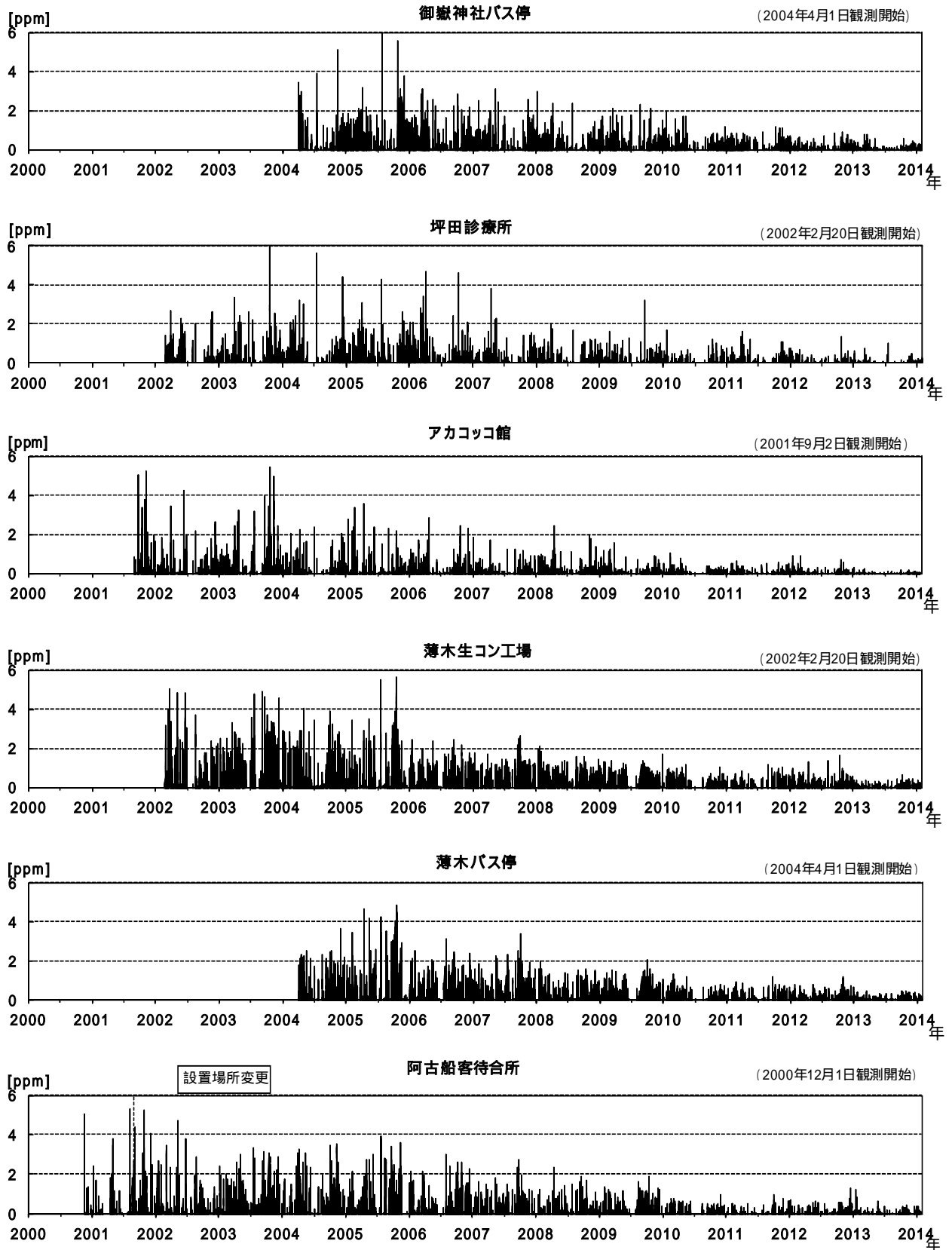
第 7 図 - 三宅島 火山ガス観測結果 ( 1 時間値 )( 2000 年 ~ 2014 年 1 月 ) グラフは三宅村から提供された火山ガスデータをもとに気象庁が作成。
