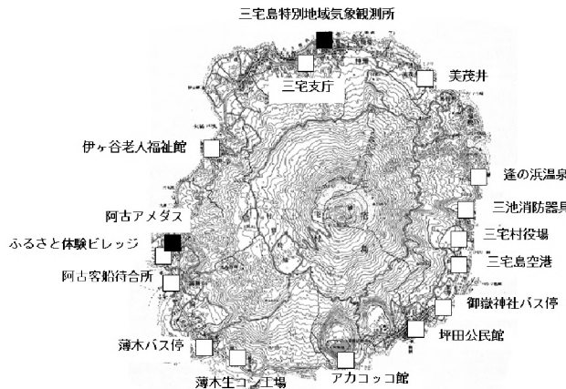
第7図 - 三宅島 火山ガス観測結果（1時間値）と三宅島特別地域気象観測所の風向風速（気象庁）（2000年～2014年1月）および三宅村火山ガス観測点配置図
