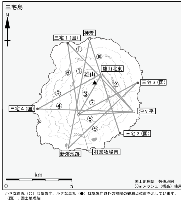
第 11 図 三宅島 GNSS 基線図
