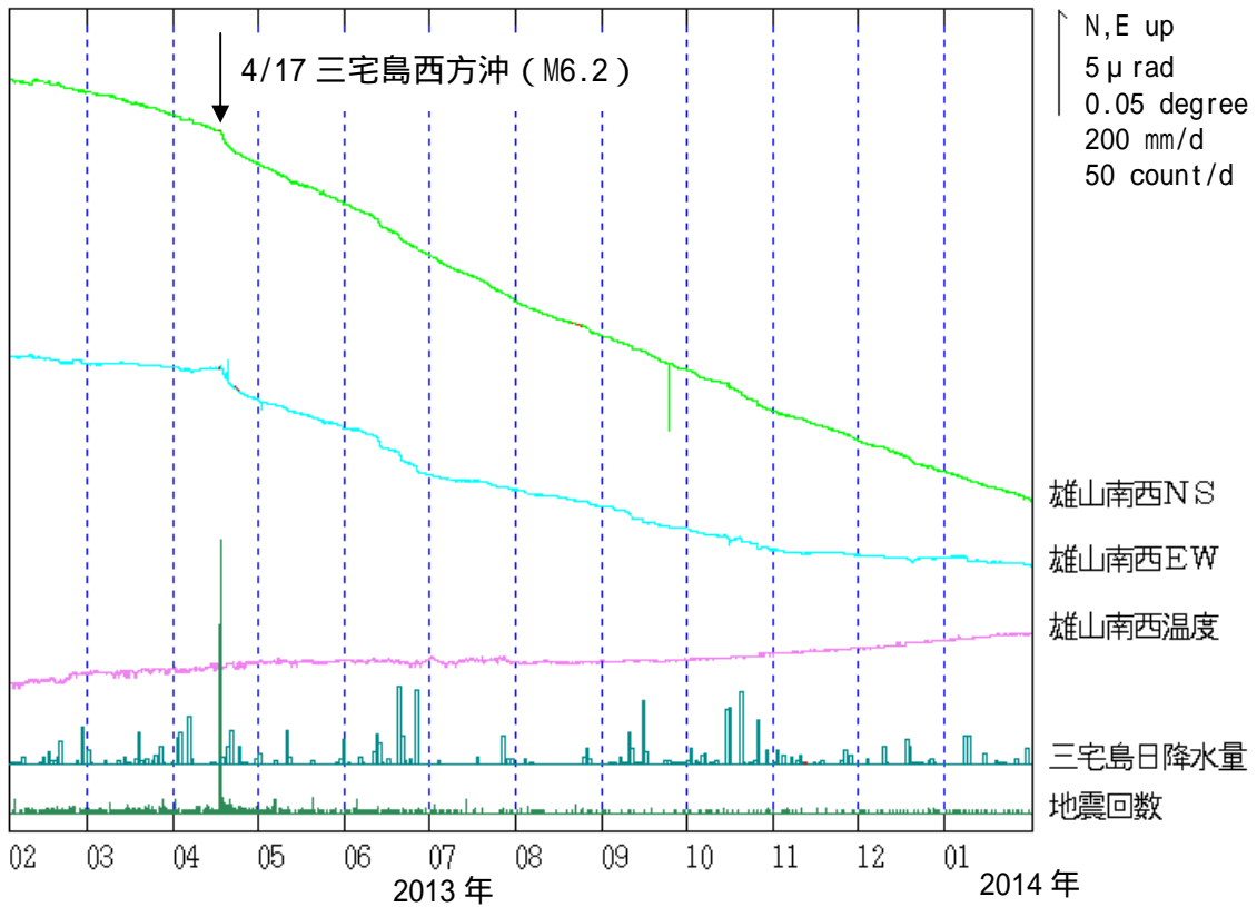
第 12 図 三宅島 雄山南西観測点における傾斜変動
