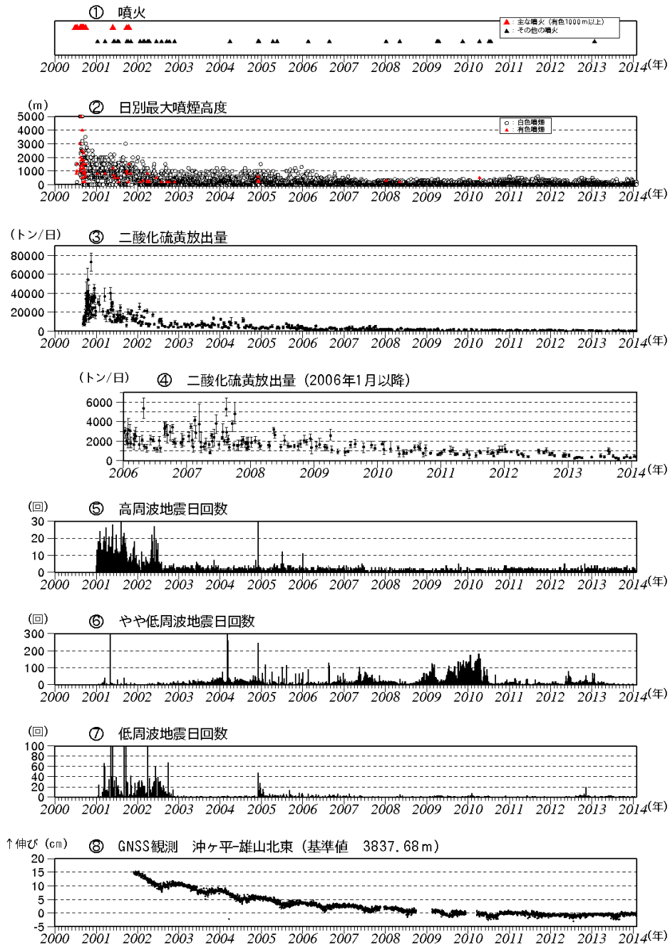
第 5 図 三宅島 火山活動経過図 (2000 年 1 月 1 日 ~ 2014 年 1 月 31 日)
