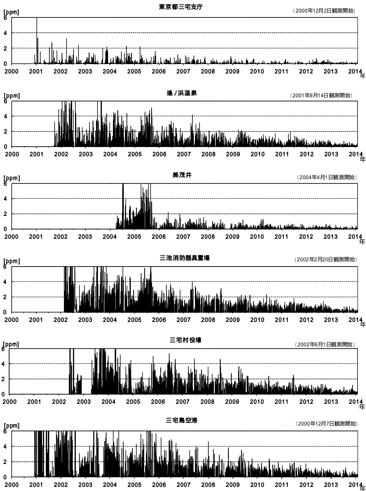
第 7 図 - 三宅島 火山ガス観測結果 ( 1 時間値 ) ( 2000 年 ~ 2014 年 1 月 ) グラフは三宅村から提供された火山ガスデータをもとに気象庁が作成。
