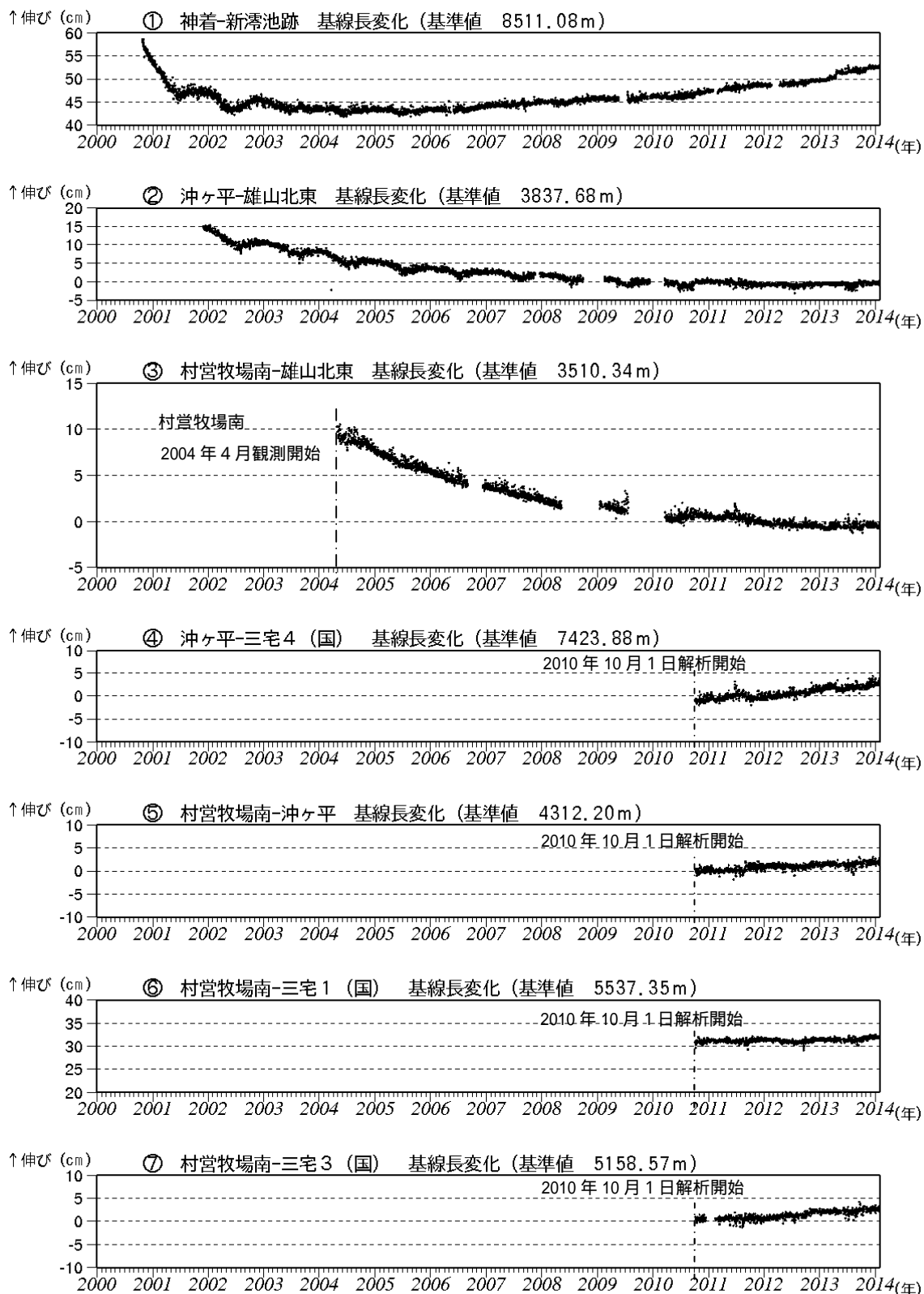
第10図 - 三宅島 GNSS連続観測による基線長変化 (2000年10月～2014年1月31日)
