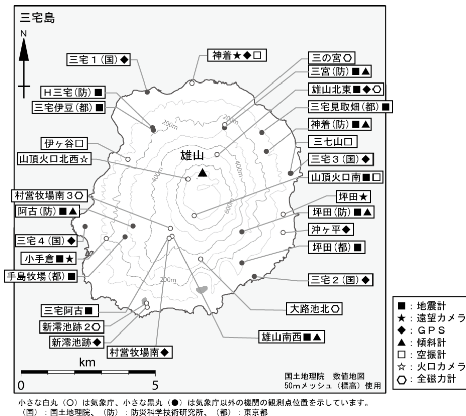
第 1 図 三宅島 観測点配置図
