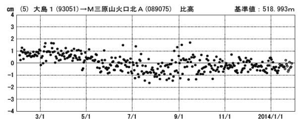
第2図(b) 伊豆大島のGNSS連続観測結果(比高:左列2009年2月~2014年1月、右列2013年2月~2014年1月)
