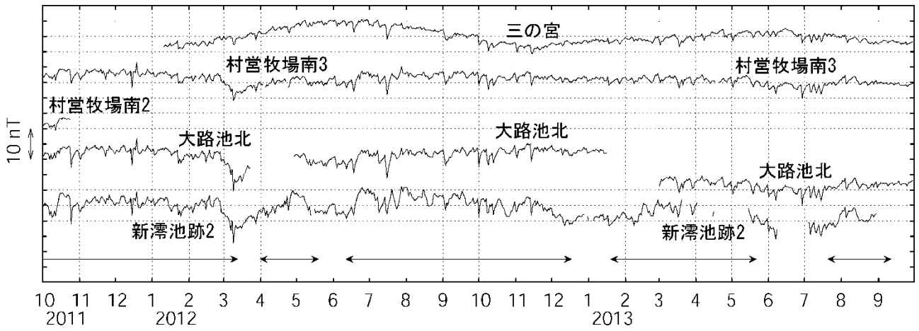
第2図 気象庁観測点の全磁力値と雄山北東（参照点）の全磁力値の日平均差（2011年10月～2013年9月）
