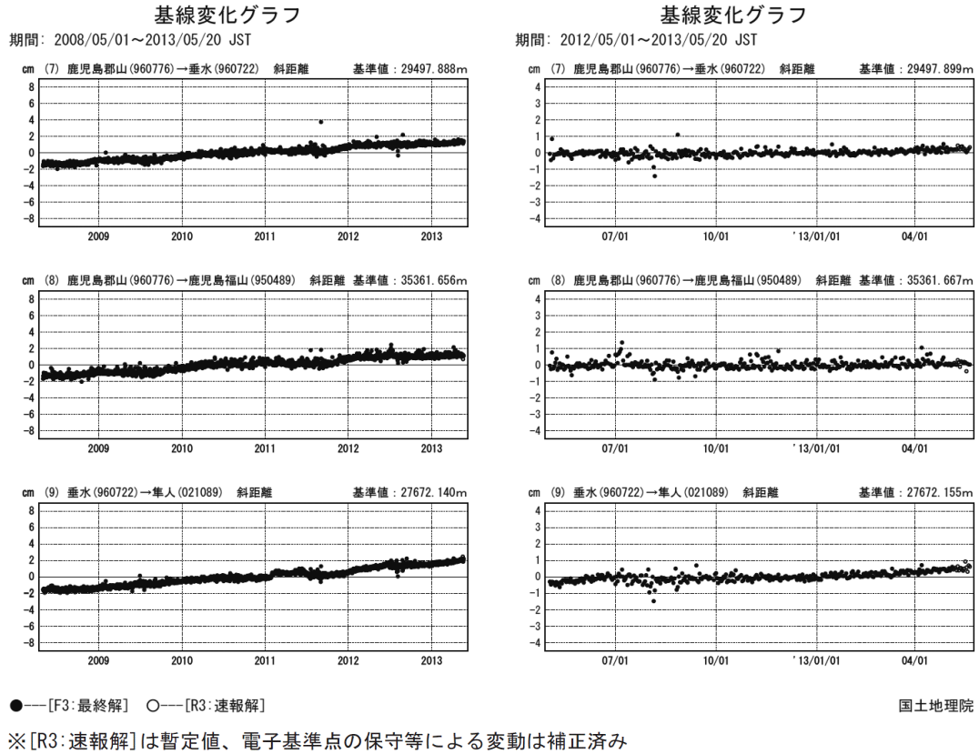
第2図(b) 桜島周辺のGNSS連続観測結果(基線長 左列:2008年5月~2013年5月、右列:2012年5月~2013年5月)
