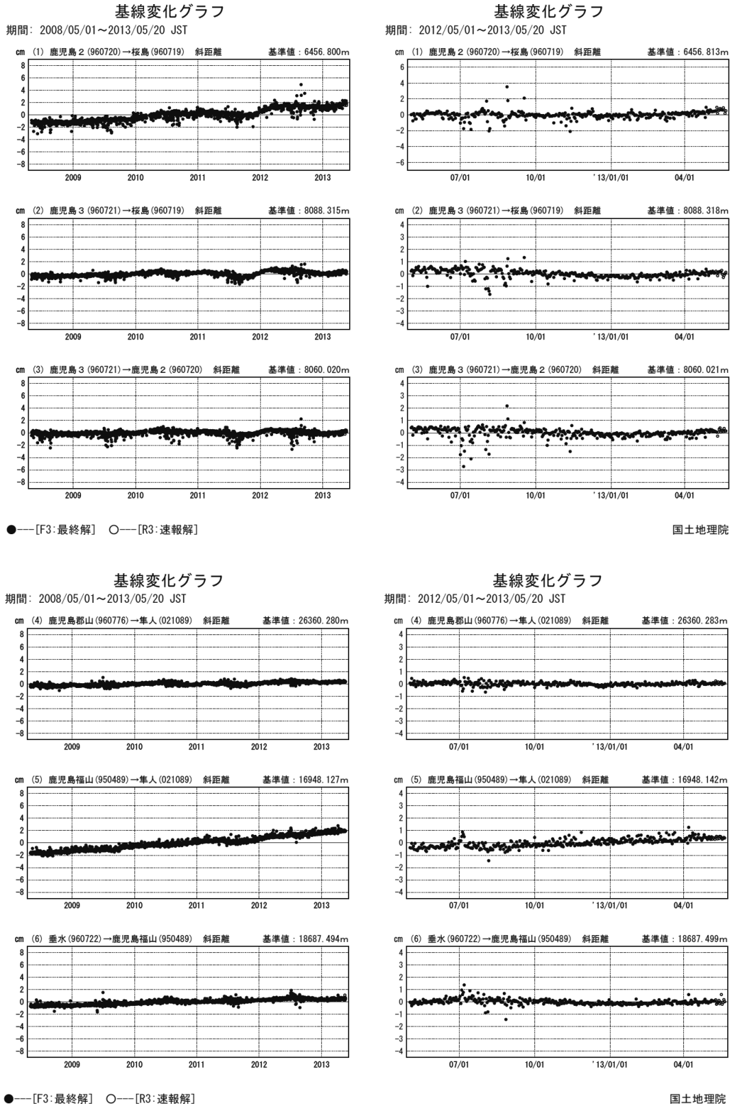
第2図(a) 桜島周辺のGNSS連続観測結果(基線長 左列:2008年5月～2013年5月、右列:2012年5月～2013年5月)
