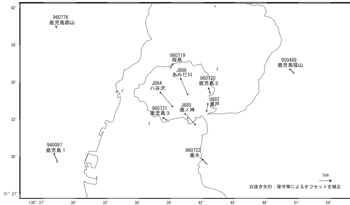
第4図 桜島におけるGNSS連続観測点(国土地理院・気象庁観測点統合解析による)水平変動ベクトル図 (上段: 2013年1月~2013年4月、下段: 2012年4月~2013年4月)
