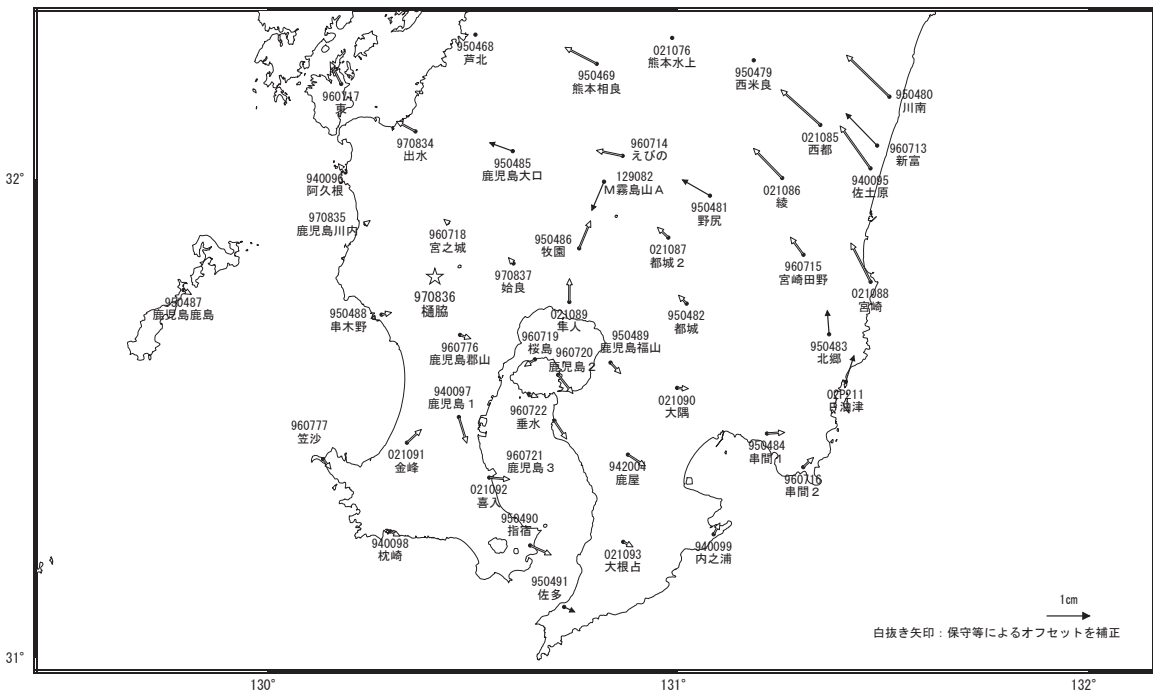
第3図 桜島周辺におけるGNSS観測点の水平変動ベクトル図(上段:2013年2月~2013年5月、下段:2012年5月~2013年5月)
