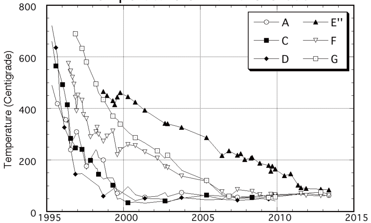
第3図 平成新山ドームの噴気ガスの温度変化。
