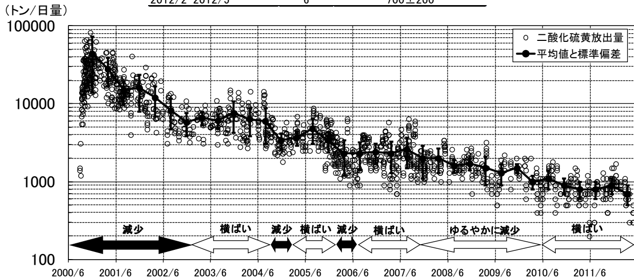
第4図* 三宅島 二酸化硫黄放出量と平均値の推移 (第3図-③を対数スケールで表示)
