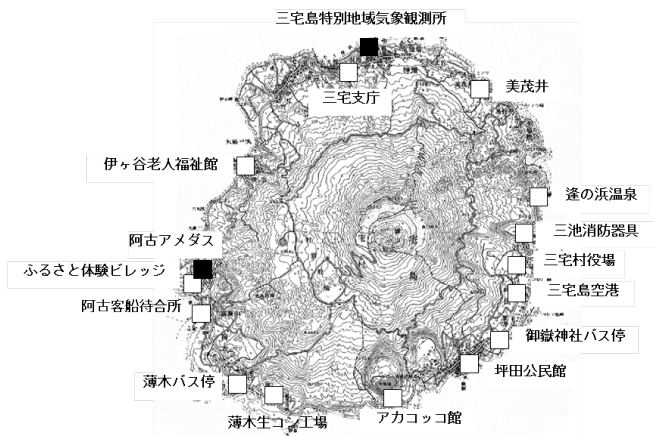
第5図※-③ 三宅島 火山ガス観測結果（1時間値）と三宅島特別地域気象観測所の風向風速（気象庁） （2000年～2012年5月）および三宅村火山ガス観測点配置図 グラフは三宅村から提供された火山ガスデータをもとに気象庁が作成 この地図の作成には、国土地理院発行の『2万5千分の1地形図（三宅島）』を使用した。
