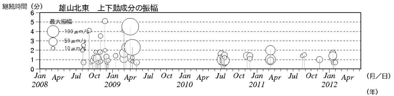
第7図 三宅島 単発的な火山性微動の活動経過図 (2008年1月1日~2012年5月31日)
