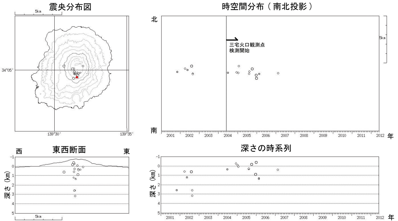
第6図※-③ 三宅島 低周波地震の震源分布 (2001年1月1日~2012年5月31日)
