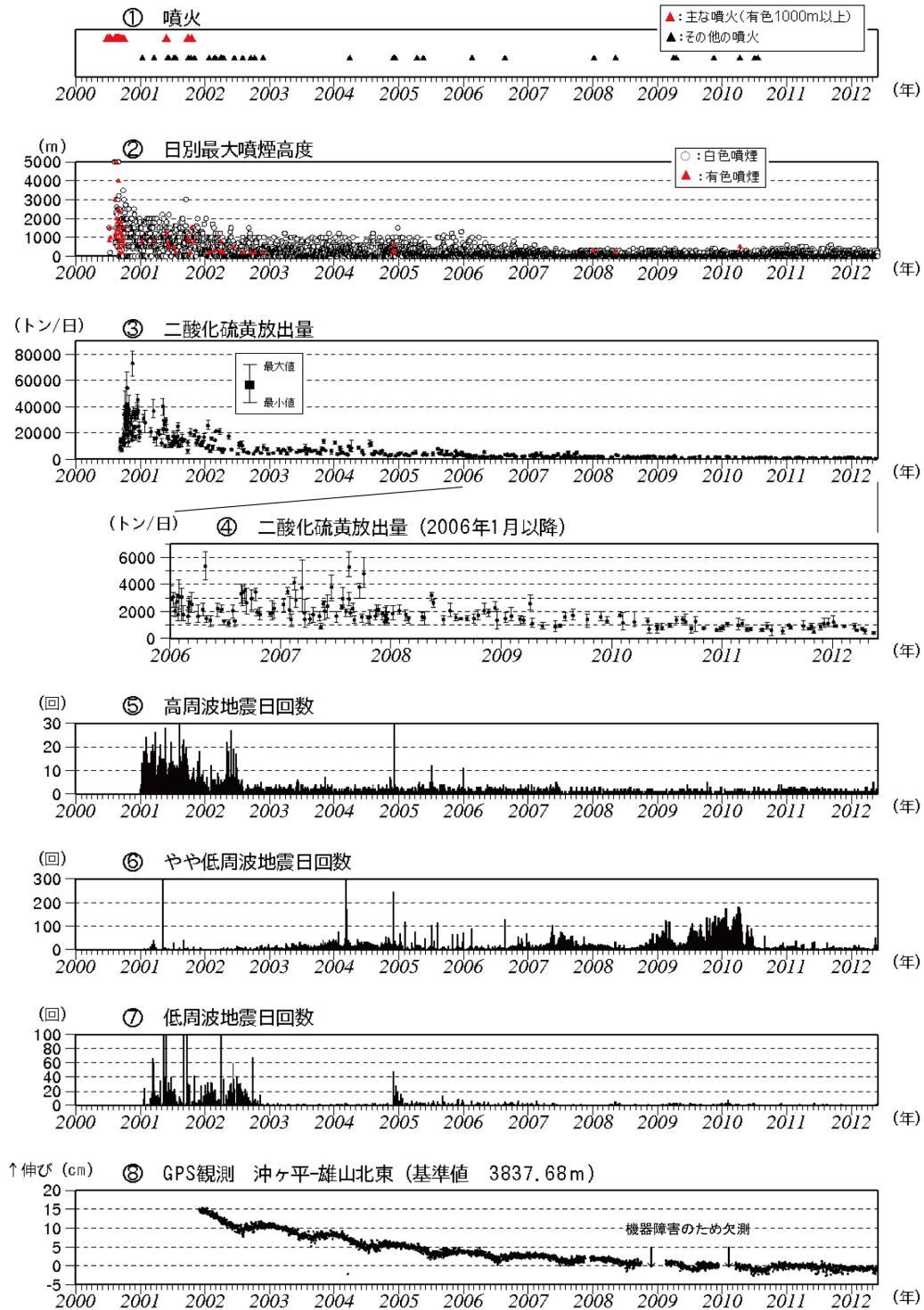
第3図※ 三宅島 火山活動経過図 (2000年1月1日～2012年5月31日)
