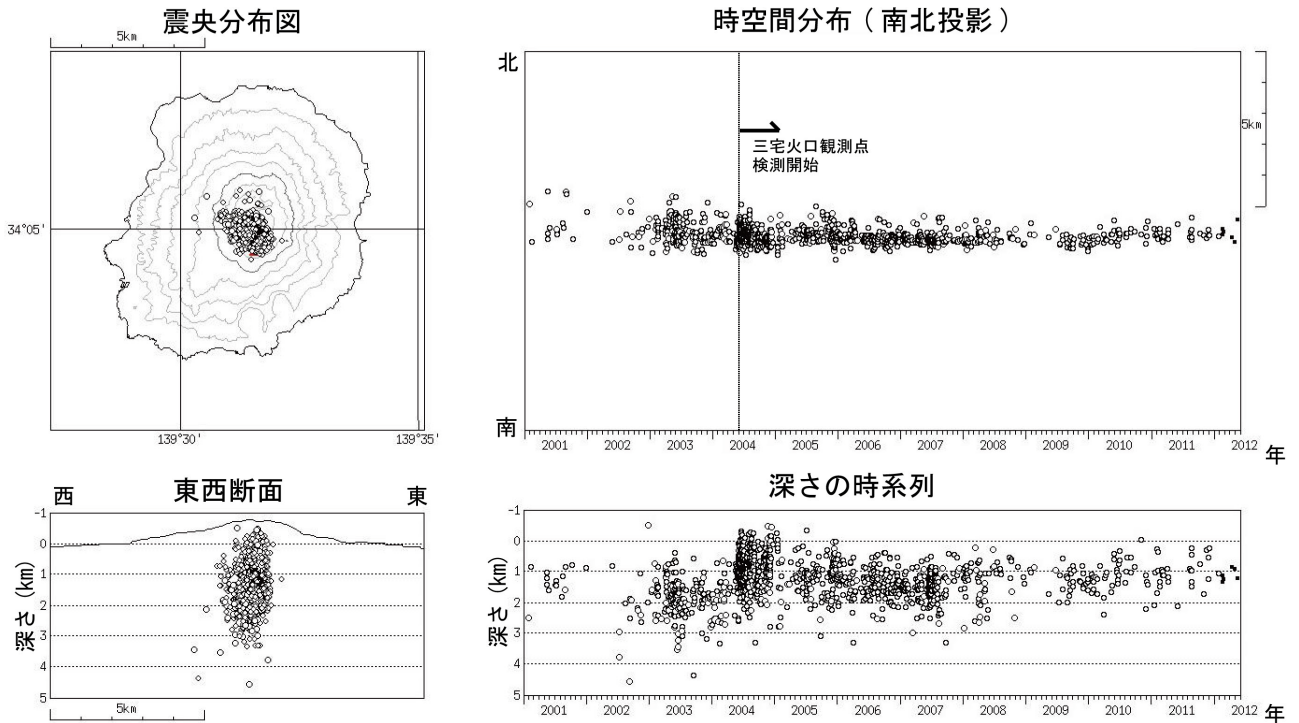
第6図*② 三宅島 やや低周波地震の震源分布 (2001年1月1日~2012年5月31日) ○ : 2001年1月1日~2012年1月31日 ● : 2012年2月1日~5月31日 この地図の作成には、国土地理院発行の『数値地図50mメッシュ (標高)』を使用した。 ・今期間、やや低周波地震は5月に一時的にやや多い状態だったが、それ以外の期間は少ない状態で経過している。
