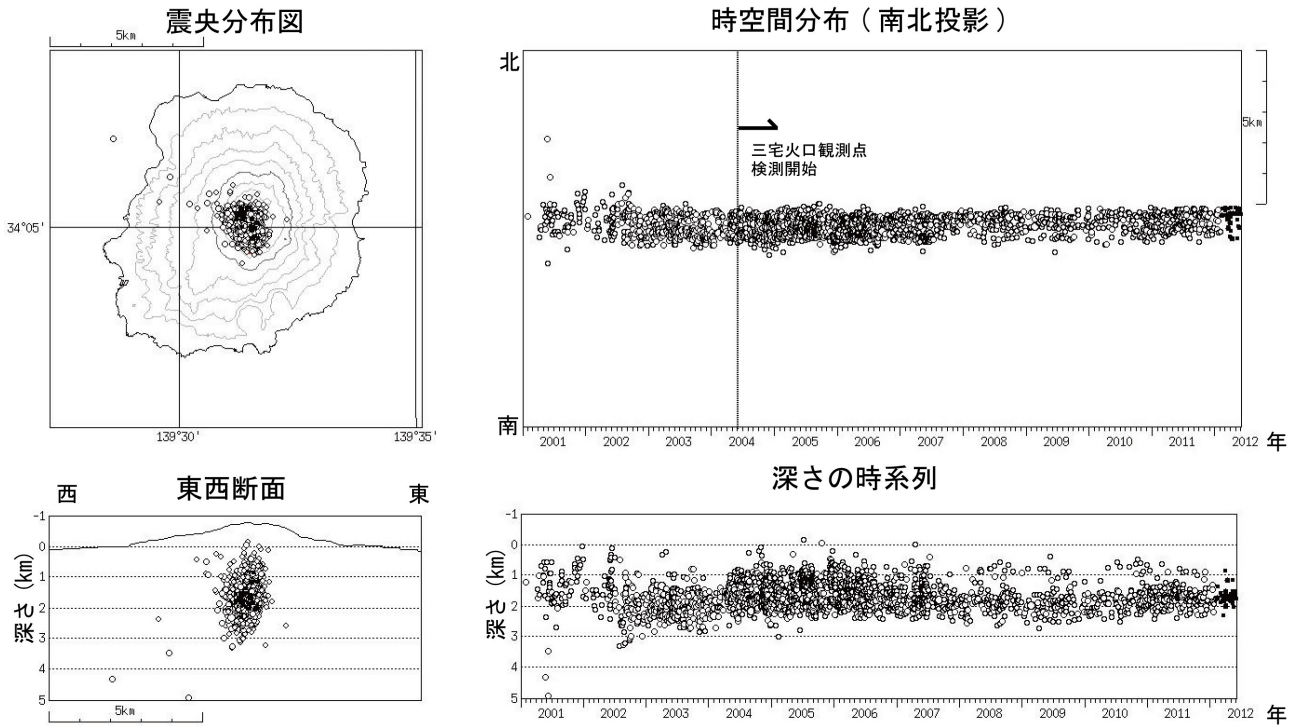
第6図*① 三宅島 高周波地震の震源分布 (2001年1月1日~2012年5月31日) ○ : 2001年1月1日~2012年1月31日 ● : 2012年2月1日~5月31日 この地図の作成には、国土地理院発行の『数値地図50mメッシュ (標高)』を使用した。 ・今期間、高周波地震は少ない状態で経過した。
