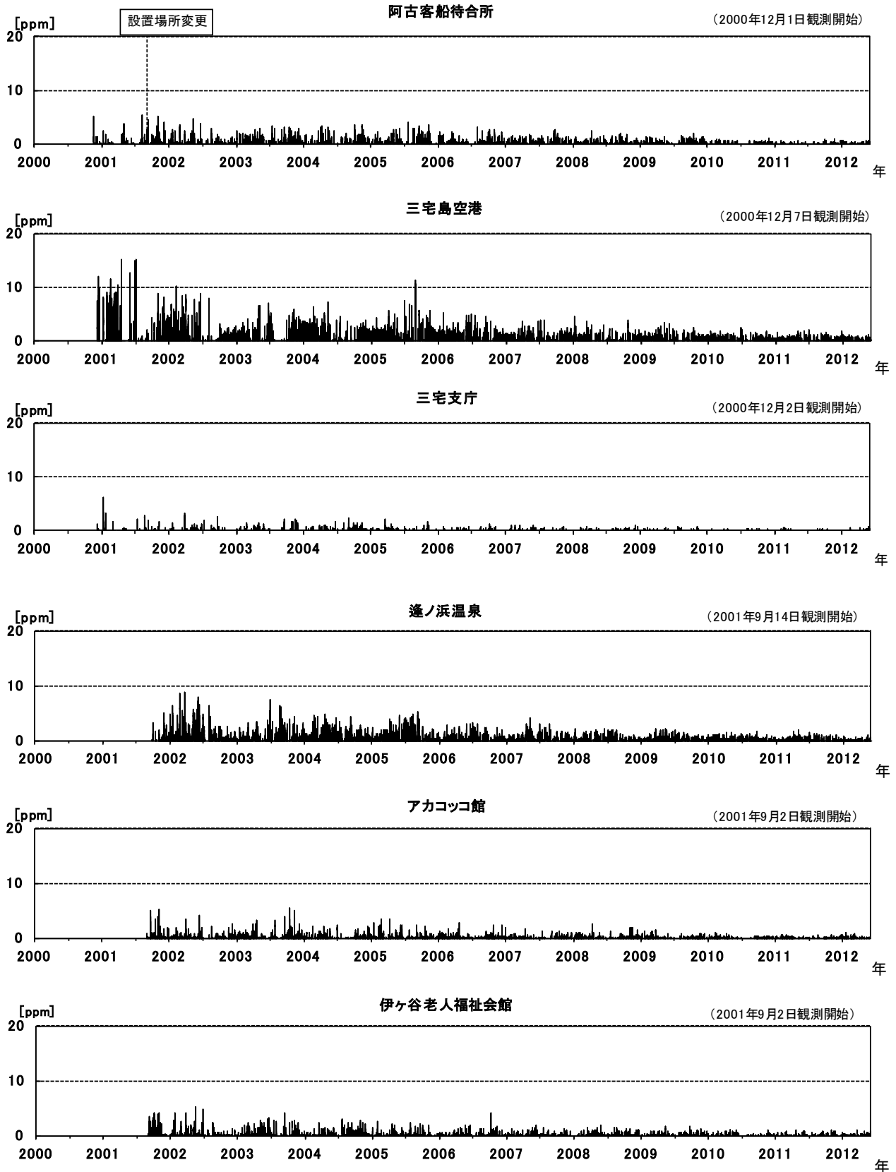
第5図*—① 三宅島 火山ガス観測結果（1時間値）（2000年～2012年5月） グラフは三宅村から提供された火山ガスデータをもとに気象庁が作成。
