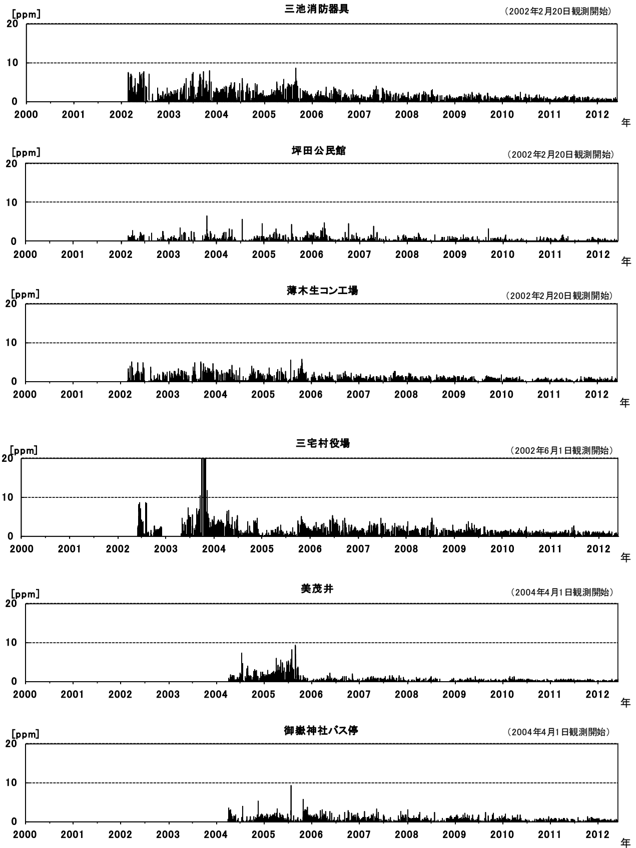
第5図*—② 三宅島 火山ガス観測結果（1時間値）（2000年～2012年5月） グラフは三宅村から提供された火山ガスデータをもとに気象庁が作成。
