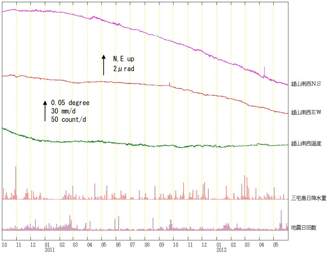
第9図 三宅島 雄山南西観測点における傾斜変動 (2010年10月1日～2012年5月31日、時間値、潮汐補正済み)
