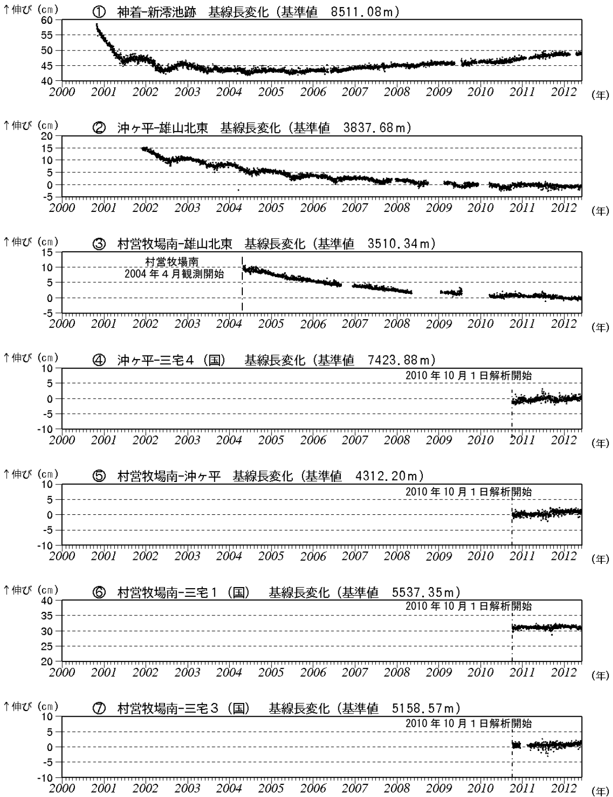
第8図*—① 三宅島 GPS連続観測による基線長変化 (2000年10月～2012年5月31日)
