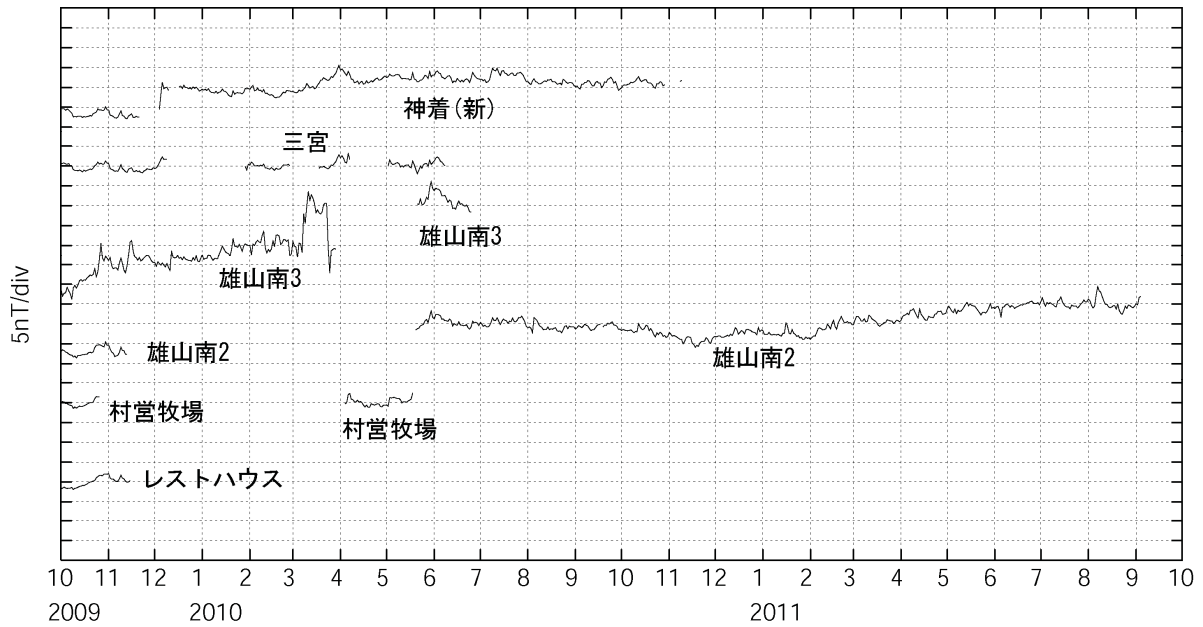
第3図 東京大学各観測点の全磁力値と参照点の全磁力値の日平均差 (2009年10月～2011年9月)
