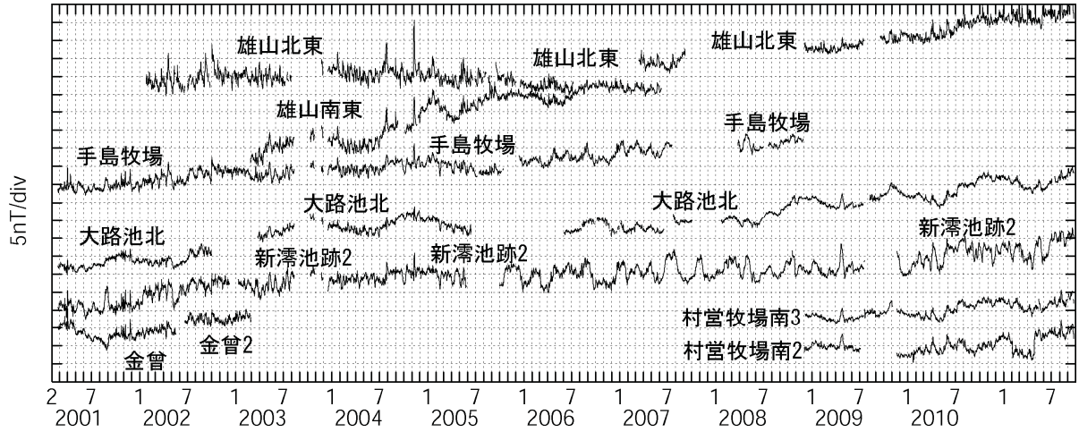
第4図 気象庁観測点の全磁力値と参照点の全磁力値の日平均差 (2001年2月～2011年9月)
