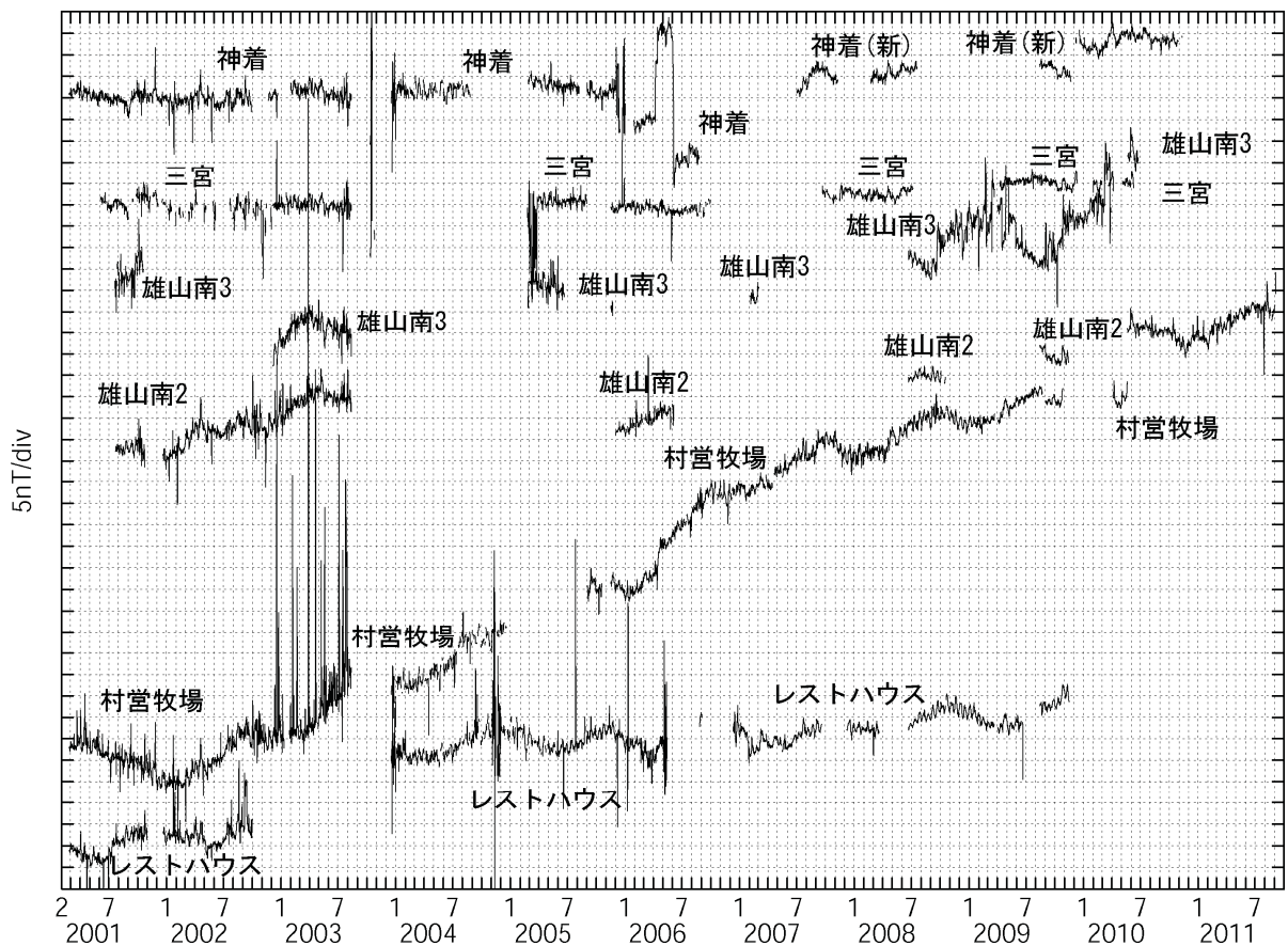
第5図 東京大学地震研究所観測点の夜間全磁力変化(参照点との単純差) (2001年2月～2011年9月)
