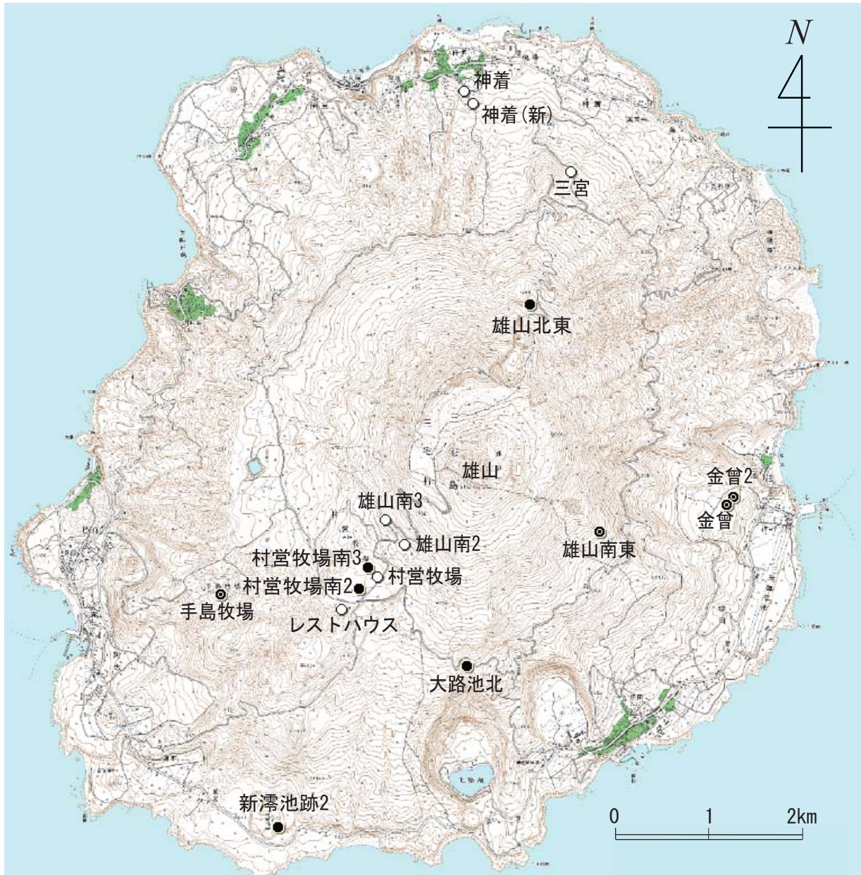
第1図 全磁力観測点配置図 (●: 気象庁、◎: 気象庁 (観測終了)、○: 東大地震研究所 (観測終了))。
