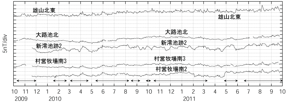
第2図 気象庁観測点の全磁力値と参照点の全磁力値の日平均差 (2009年10月～2011年9月)。
