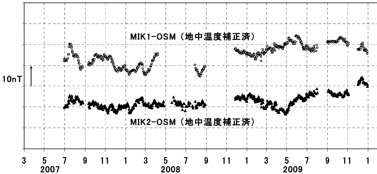
第3図 地中温度補正後の全磁力日平均値差
