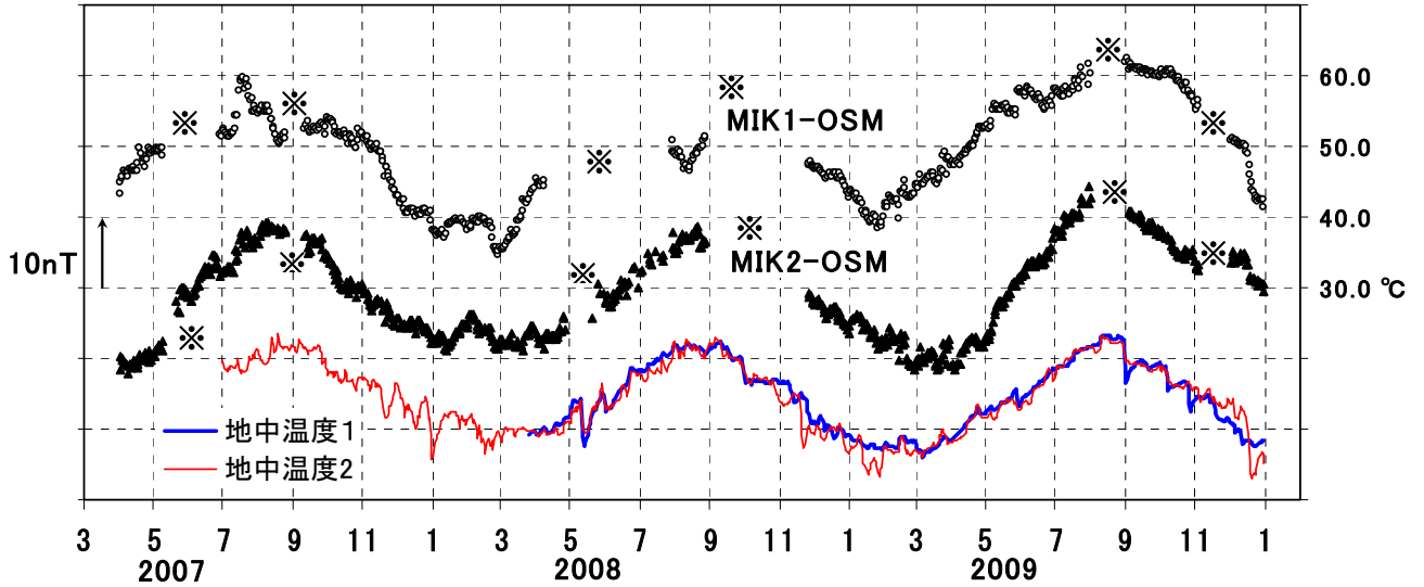
第2図 2007年4月から2009年12月までの連続観測点MIK1、MIK2における全磁力日平均値と参照点OSMの日平均値との差および観測点近傍の地中温度（※は観測装置の障害による欠測期間）
