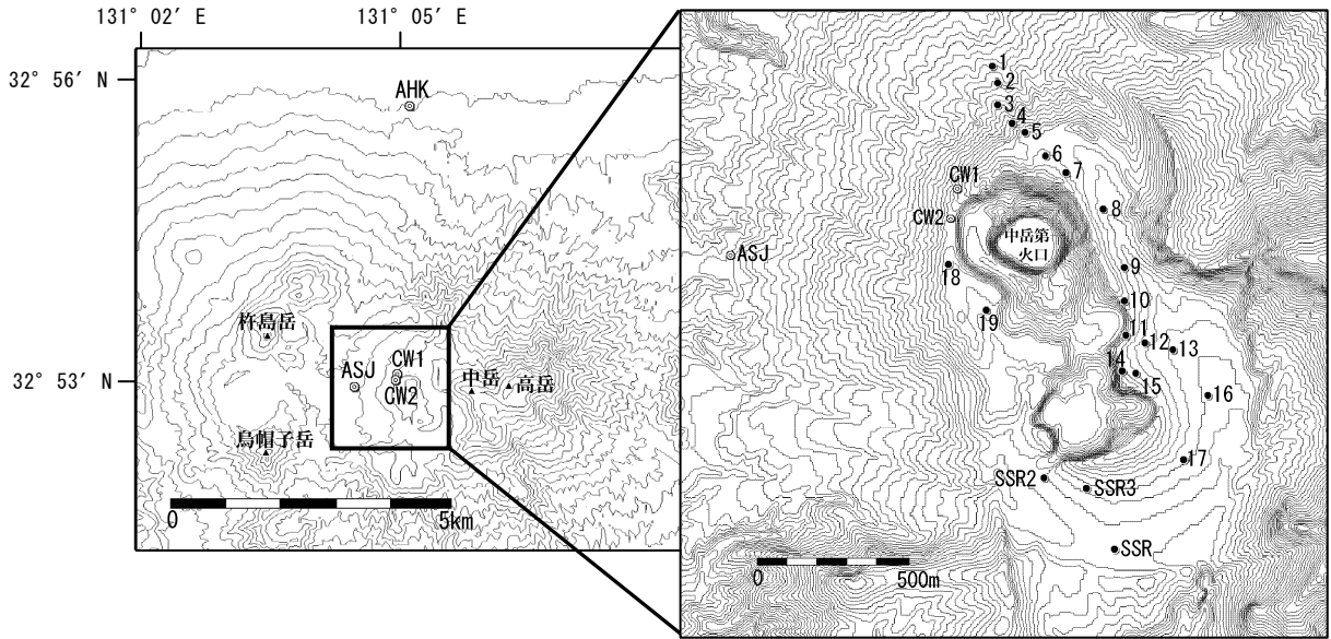
第1図 全磁力観測点配置図(◎：連続観測点 ●：繰返し観測点)
