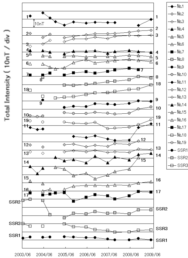
第2図 2003年6月から2009年5月までの繰返し観測点における全磁力と参照点AHKとの全磁力との差
