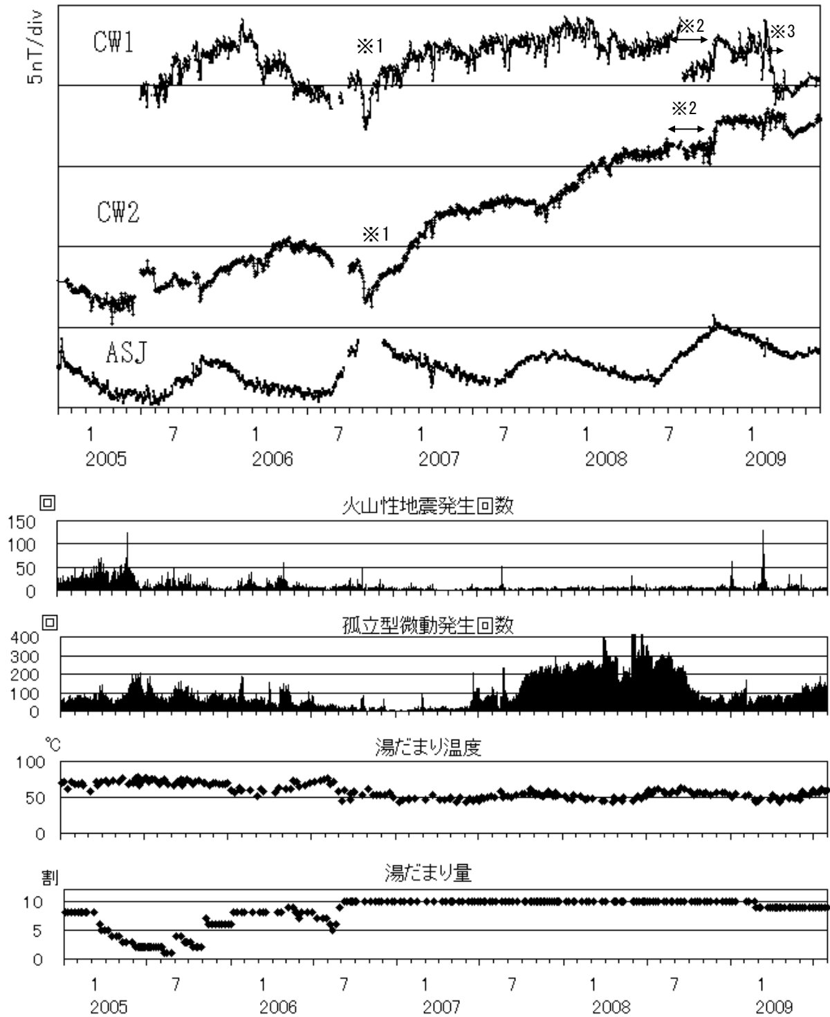
第3図 2004年11月から2009年5月まで連続観測点CW1、CW2、ASJにおける全磁力日平均値と参照点AHKの日平均値との差、火山性地震発生回数、孤立型微動発生回数、湯だまり温度、湯だまり量。
