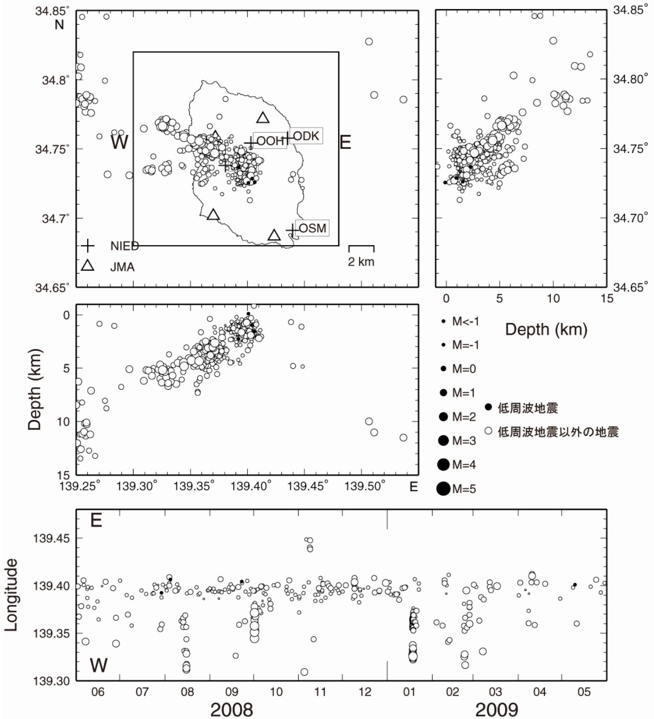
第1図 伊豆大島の震源分布および時空間分布図。低周波地震は●で示す。表示期間は2008年6月1日～2009年5月31日。
