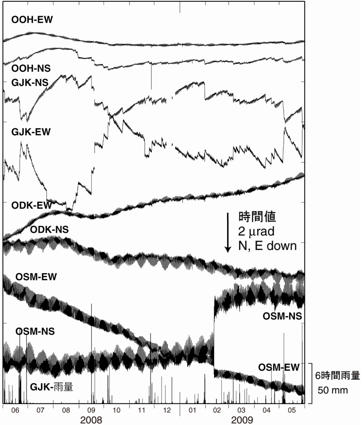
第2図 防災科学技術研究所・伊豆大島火山活動観測網による傾斜変動観測結果。表示期間は2008年6月1日~2009年5月31日で、表示データは時値(毎正時の値)。破線で示す時期にドリフトの方向が変化している。
