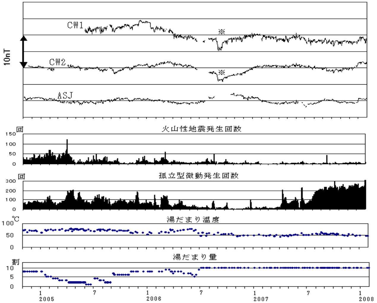
第3図 連続観測点CW1、CW2、ASJの全磁力変化からAHKの全磁力及び地磁気観測所鹿屋出張所の地磁気3成分を参照して広域的変動を除去した残差、火山性地震発生回数、孤立型微動発生回数、湯だまり温度。※印の変化の原因は不明。
