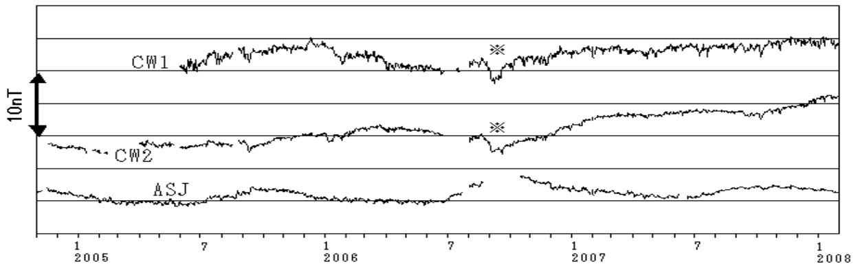
第2図 2004年11月から2008年1月まで連続観測点CW1、CW2、ASJにおける全磁力日平均値と参照点AHKの日平均値との差。※印の変化の原因は不明。
